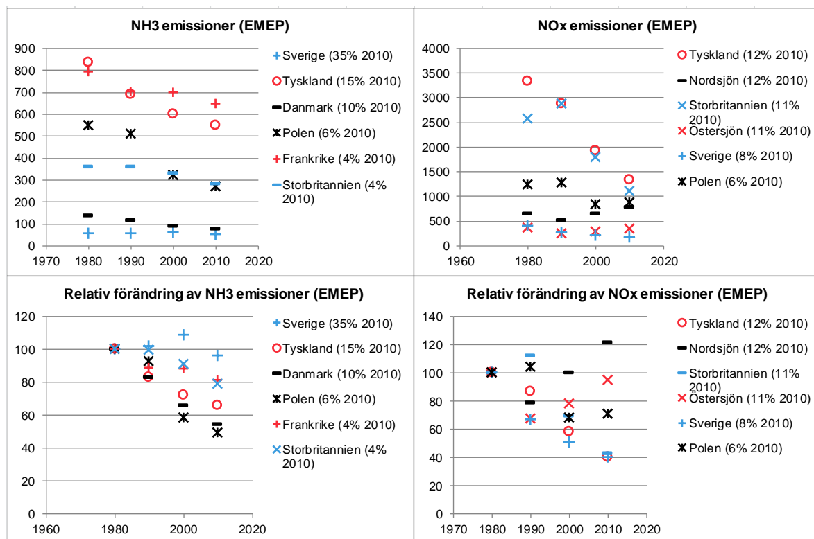
Figur 6.4. Årliga totala emissioner för de 6 länder som enligt beräkningar med EMEP modellen bidrog mest till nedfallet i Sverige 2010. Värdet i % efter landets namn indikerar hur stor del av den svenska totaldepositionen 2010 som kom från landet. Övre panelerna visar ländernas totala emission i Gg år -1 . Data är från EMEP data note 1/2012.
