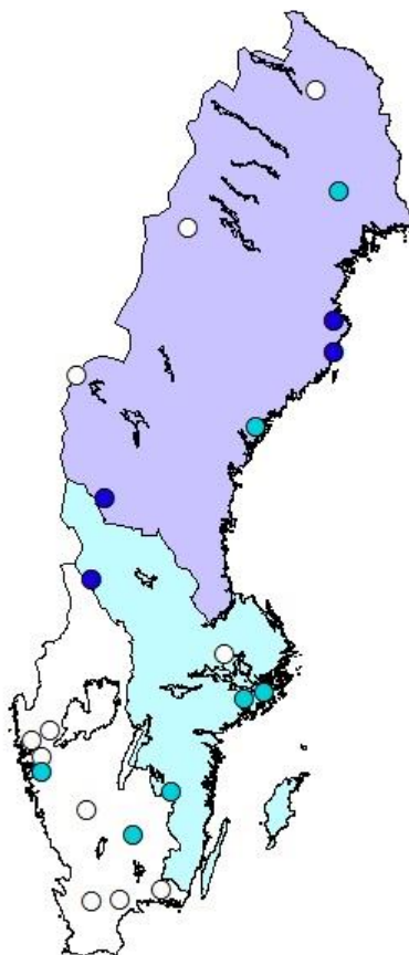
(b) \text{NO}_3^- + \text{NH}_4^+ deposition KLIMATMATCH
