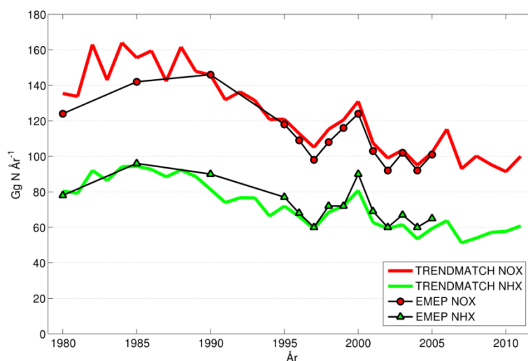
Figur 6.10. Modellerad totaldeposition av \text{NO}_3^- och \text{NH}_4^+ ( \text{GgN år}^{-1} ) till Sverige 1980-2011. MATCH-resultat från denna studie (TRENDMATCH), EMEP resultat från Klein m.fl. (2007).
