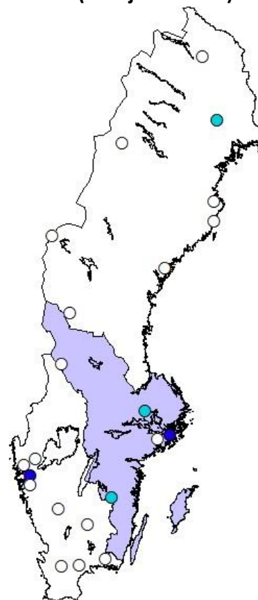
(c) \text{NO}_3^- + \text{NH}_4^+ deposition Mätdata (som jämförelse)
