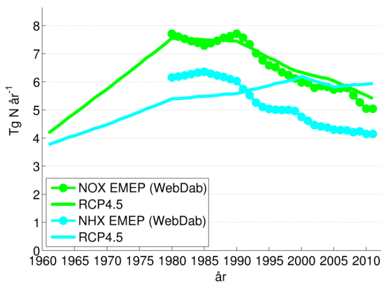
Figur 5.1. Tidsutveckling av årliga emissioner av \text{NO}_y och \text{NH}_x ( \text{TgN år}^{-1} ) i MATCH-området i perioden 1960-2011. MATCH-området framgår av Figur 5.2.
