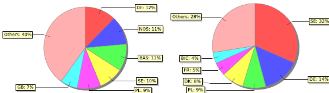
Figur 6.1. Fördelningen av källor för den svenska totaldepositionen av \text{NO}_y (till vänster) och \text{NH}_x (till höger) för år 2010. Data är från EMEP data note 1/2012.
