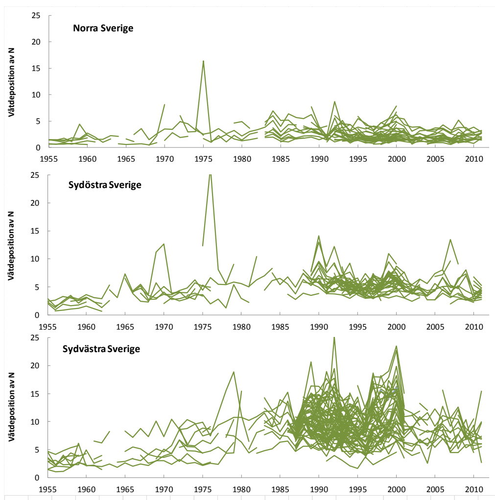
Figur. 3.5. Våtdeposition av oorganiskt kväve ( \text{NO}_3 + \text{NH}_4^+ ) ( \text{kg ha}^{-1} \text{år}^{-1} ) för mätstationer i de tre områdena N, SÖ, och SV från 1955 till 2011. Mätplatser med mindre än fem års data är inte medtagna.
