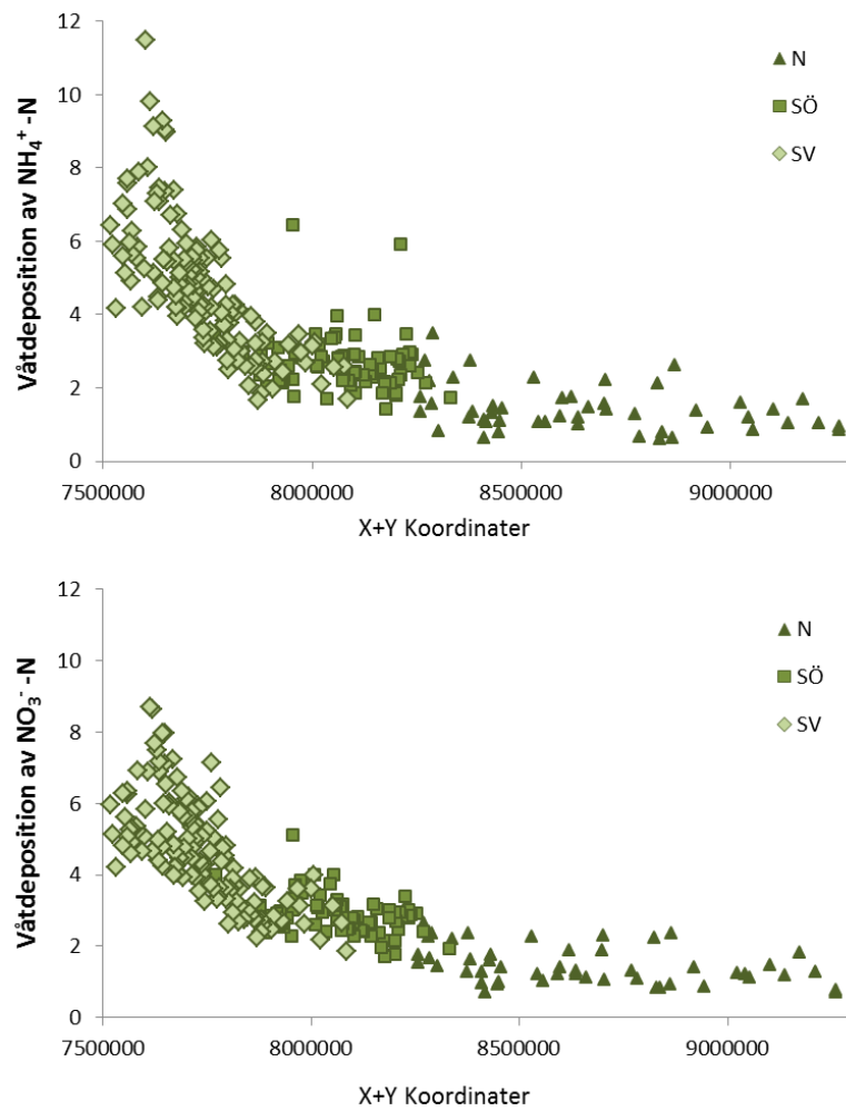
Figur 3.3. Aritmetriska medelvärden av våtdepositionen av NH 4 + och NO 3 - (kg ha -1 år -1 ) för perioden 1990-2000 då flest mätningar fanns. Mätningarna är uppdelade på de tre områdena N, SÖ och SV.
