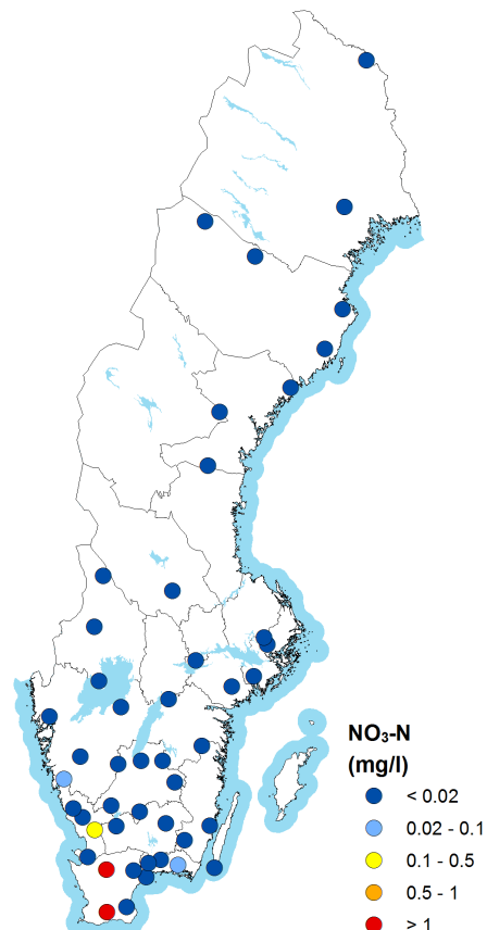
Figur 12. Koncentrationen av nitrat ( \text{NO}_3\text{-N} ) i markvattnet på 50 cm djup vid olika platser inom Krondroppsnetet redovisat som medianvärde från de senaste tre årens mätningar (2016–2018). Ytor med mindre än tre mätvärden under treårsperioden, samt ytor som har avverkats eller gödslats har tagits bort.
