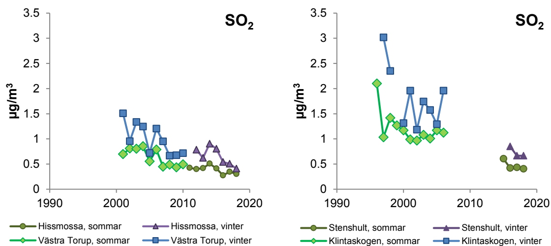
Figur 13. Lufthalter av svaveldioxid ( \text{SO}_2 ) som medelvärden för sommar- respektive vinterhalvtår för Västra Torup/Hissmossa sedan 2001, och Klintaskogen/Stenshult sedan 1996. Det finns en signifikant minskning av lufthalterna vid Västra Torup/Hissmossa både sommar och vinter sedan 2001 och vid Klintaskogen/Stenshult sedan 1996 under sommarhalvtåret och sedan 1997 under vinterhalvtåret.
