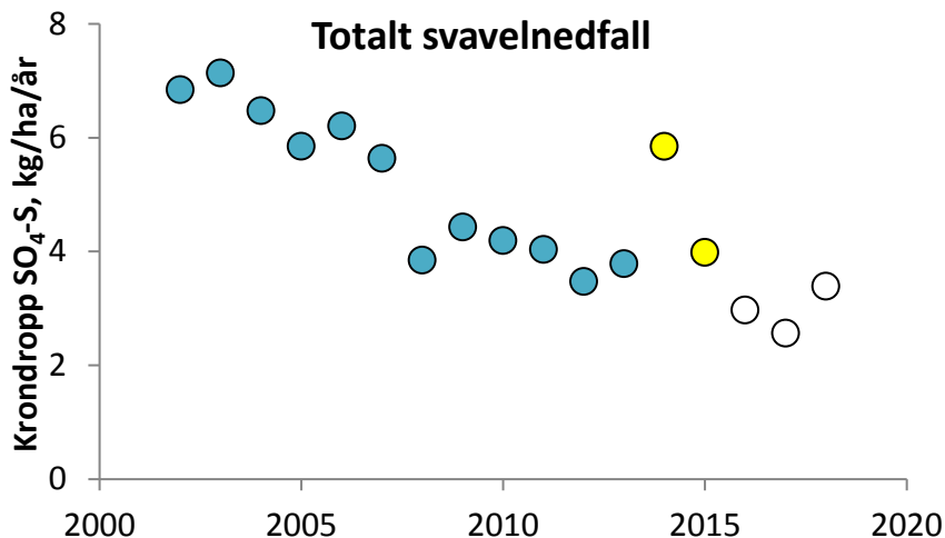
Figur 16. Årliga medelvärden för nedfall av svavel ( SO_4-S_{ex} ) mätt som krondropp för fyra platser i Skåne, Maryd, Arkelstorp A/B, Klintaskogen/Stenshult och Västra Torup/Hissmossa, under 1996/97–2017/18. Mätningarna 1996/97–2012/13 är markerade med blå symboler. Dessa mätningar utgör år före sänkningen av svavelhalten i fartygsbränsle. De hydrologiska åren 2013/14 och 2014/15 är markerade med gult då de är påverkade av vulkanutbrottet på Island (31 augusti 2014 – 27 februari 2015). Åren 2015/16–2017/18 är markerade med vitt och inträffar efter den senaste sänkningen av svavelhalten i fartygsbränslet. Hänsyn har inte tagits till att mätplatserna flyttats kortare sträckor.
