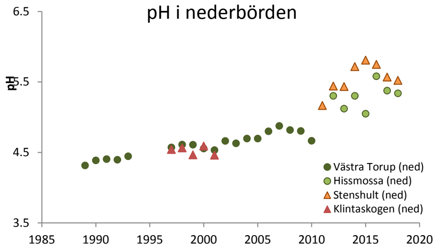
Figur 17. pH i nederbörden vid Västra Torup, Hissmossa, Klintaskogen och Stenshult. Nederbörden mäts månadsvis och pH-värdet medelvärdesbildas för hydrologiskt år, oktober–september.
