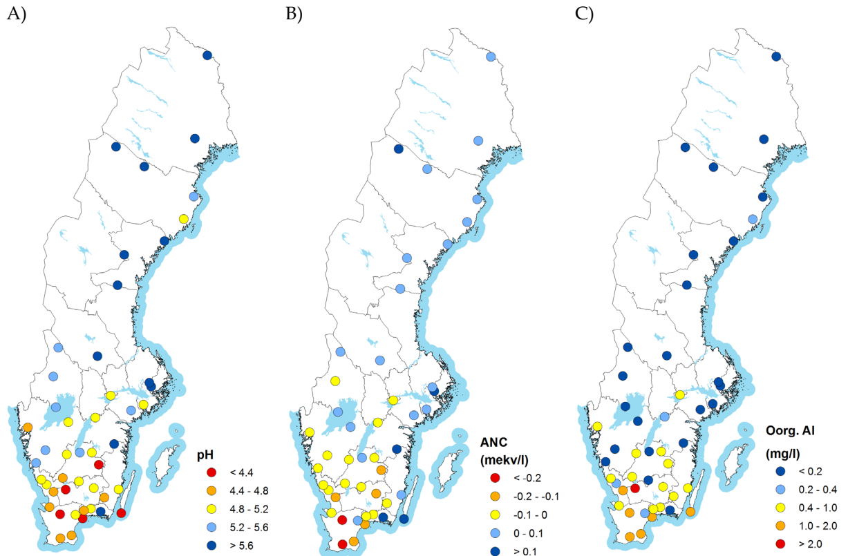
Figur 24. pH (A), ANC (B) och Oorg. AI (C) i markvattnet på 50 cm djup vid olika platser inom Krondroppsnätet. Det värde som anges är medianvärdet under de senaste tre åren (2016–2018). ANC i avrinnande vattnet bör vara betydligt över 0 när det når vattendragen. Ytor med mindre än tre mätvärden under treårsperioden, samt ytor som har avverkats eller gödslats har tagits bort.
