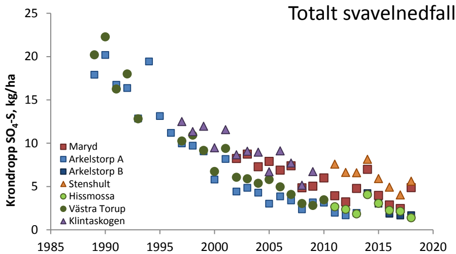
Figur 15. Årligt nedfall av svavel till Maryd, Arkelstorp, Stenshult, Hissmossa, Västra Torup och Klintaskogen i Skåne län, mätt som krondropp. Bidraget från havssalt har exkluderats. Beräkningarna gäller hydrologiskt år, oktober–september. Mätningarna vid Arkelstorp flyttades en kortare sträcka 2013, vilket indikeras med olika symboler för Arkelstorp A och B. Mätningarna vid Hissmossa ersatte Västra Torup och Stenshult ersatte Klintaskogen
