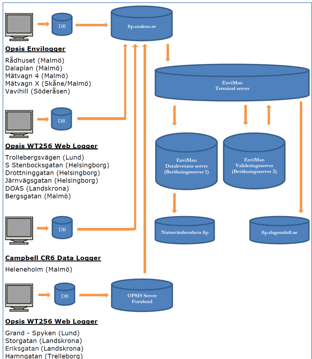
Figur 8. Principskiss över EnviMan-systemets uppbyggnad för insamling av mätdata i Skåne.
