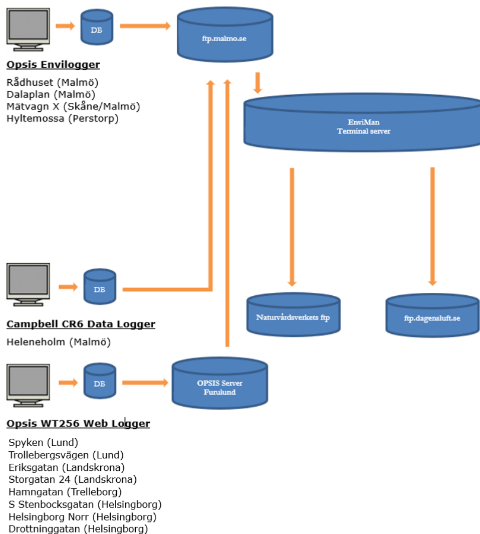
Figur 8. Principskiss över EnviMan-systemets uppbyggnad för insamling av mätdata i Skåne Dataloggning på mätstationerna
