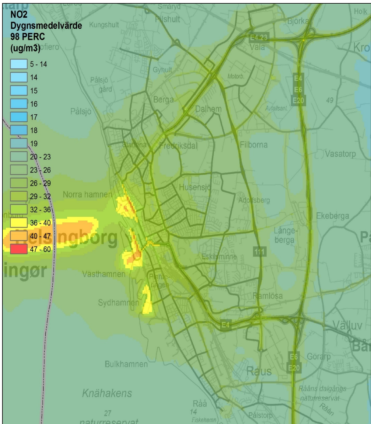
Figur 7. Beräknade dygnsnedelvärden av kvävedioxid i tätorten (µg/m 3 ).
