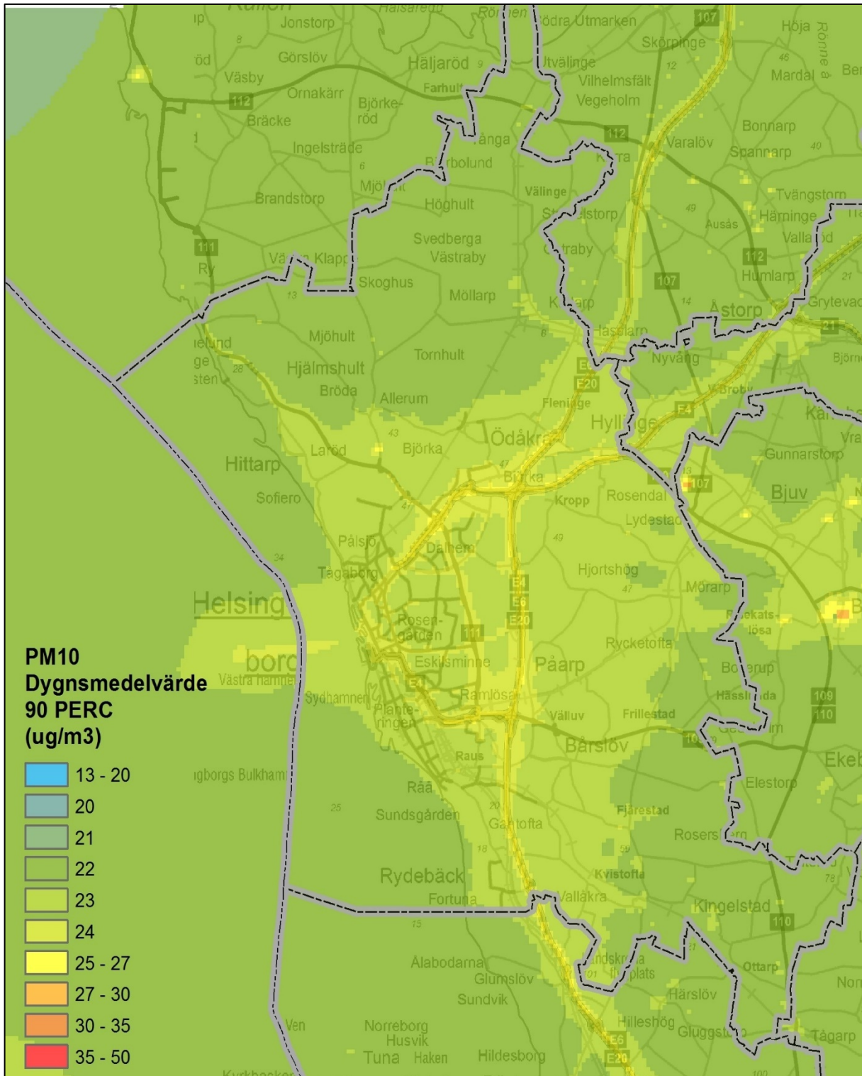
Figur 14. Beräknade dygnsmedelvärden av partiklar PM 10 inom kommunen (µg/m 3 ).
