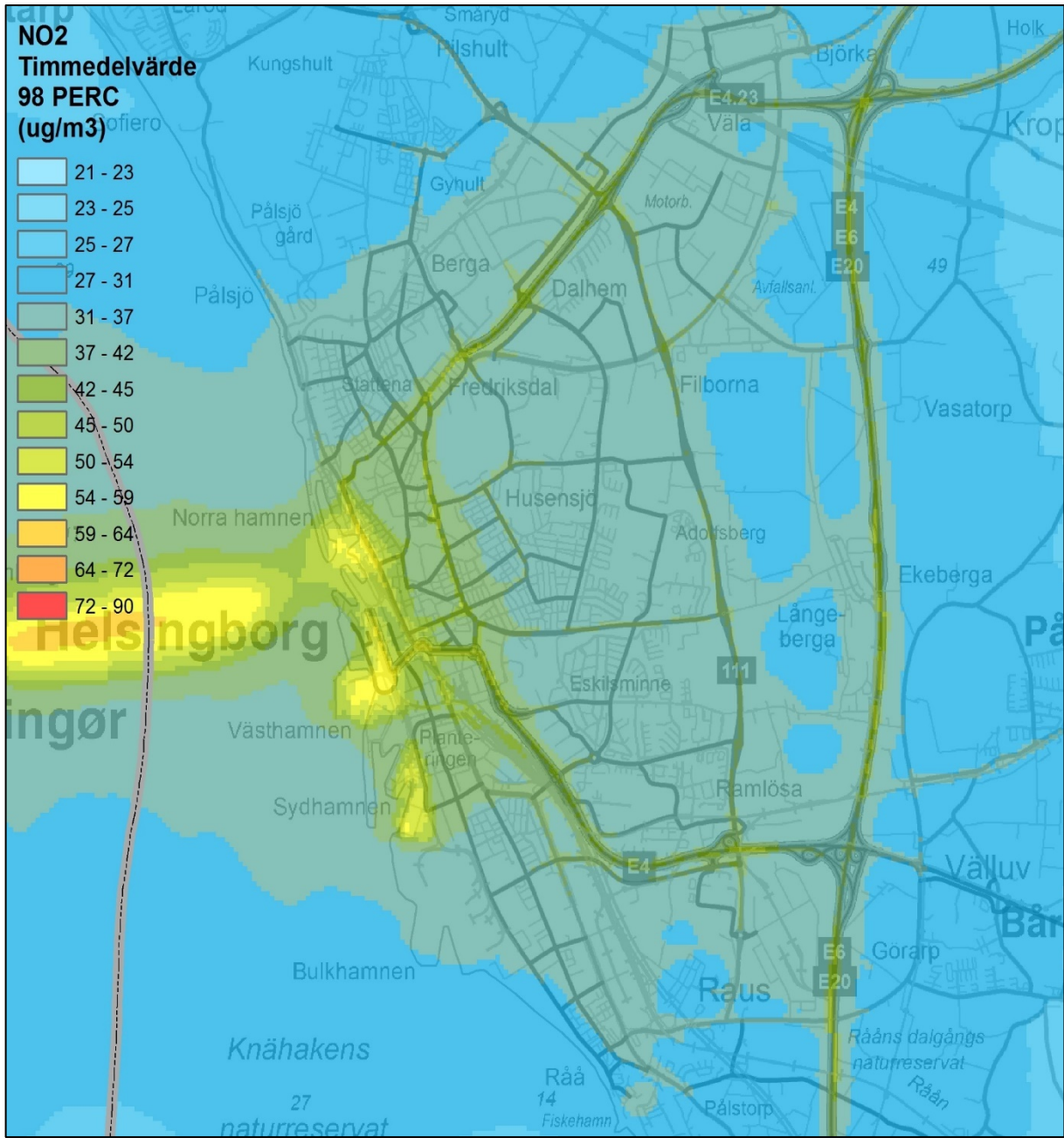
Figur 9. Beräknade timmedelvärden av kvävedioxid i tätorten (µg/m 3 ).
