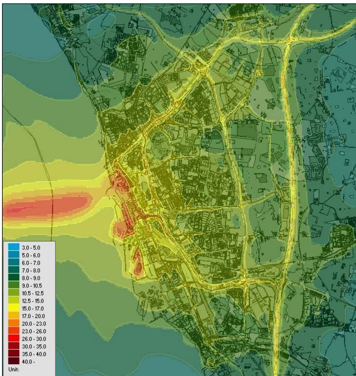
Figur 4. Beräknade årsmedelvärden av kvävedioxid i tätorten ( \mu\text{g}/\text{m}^3 ).
