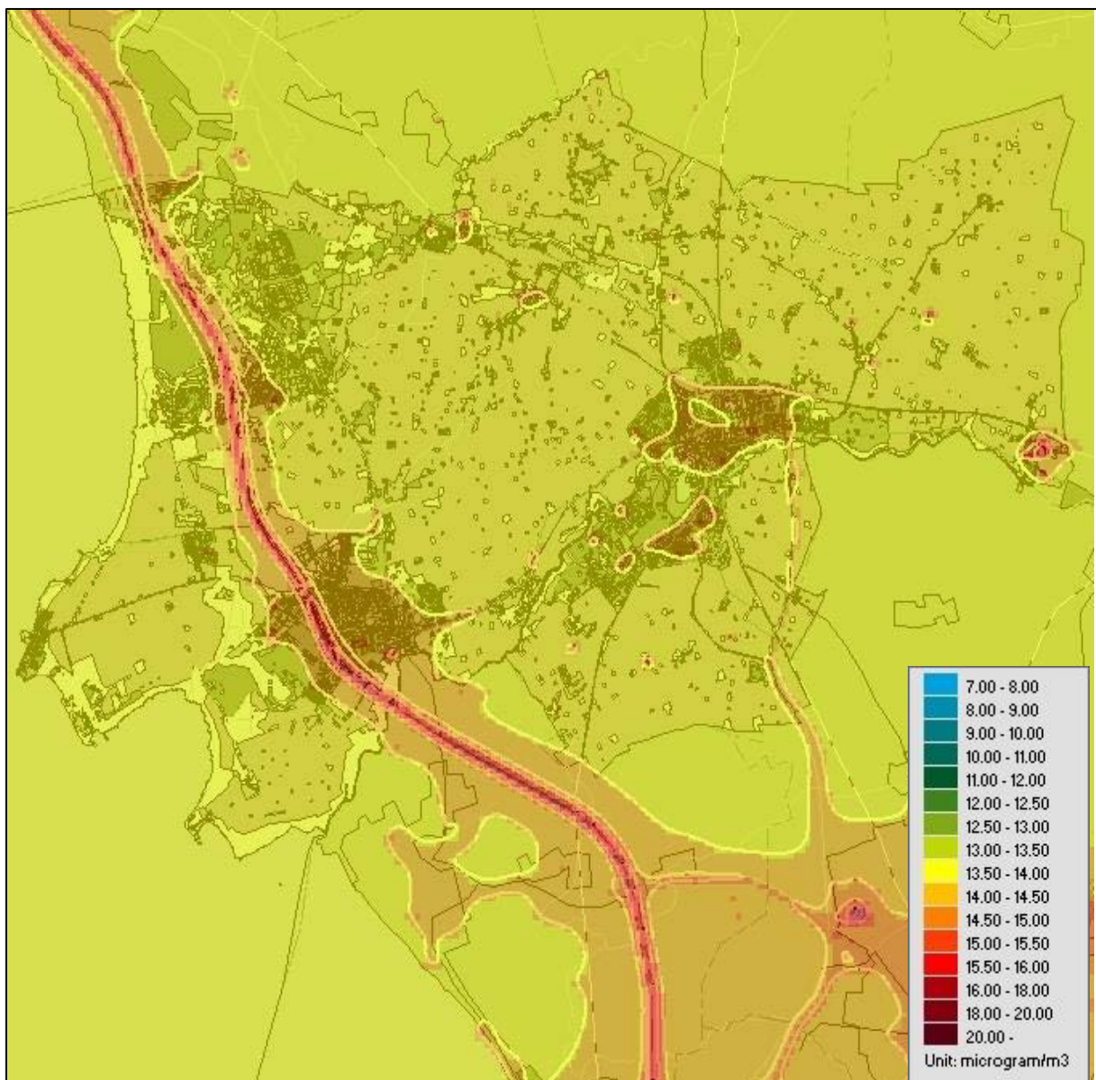
Figur 13. Beräknade årsmedelvärden av partiklar PM_{10} inom kommunen ( \mu\text{g}/\text{m}^3 ).
