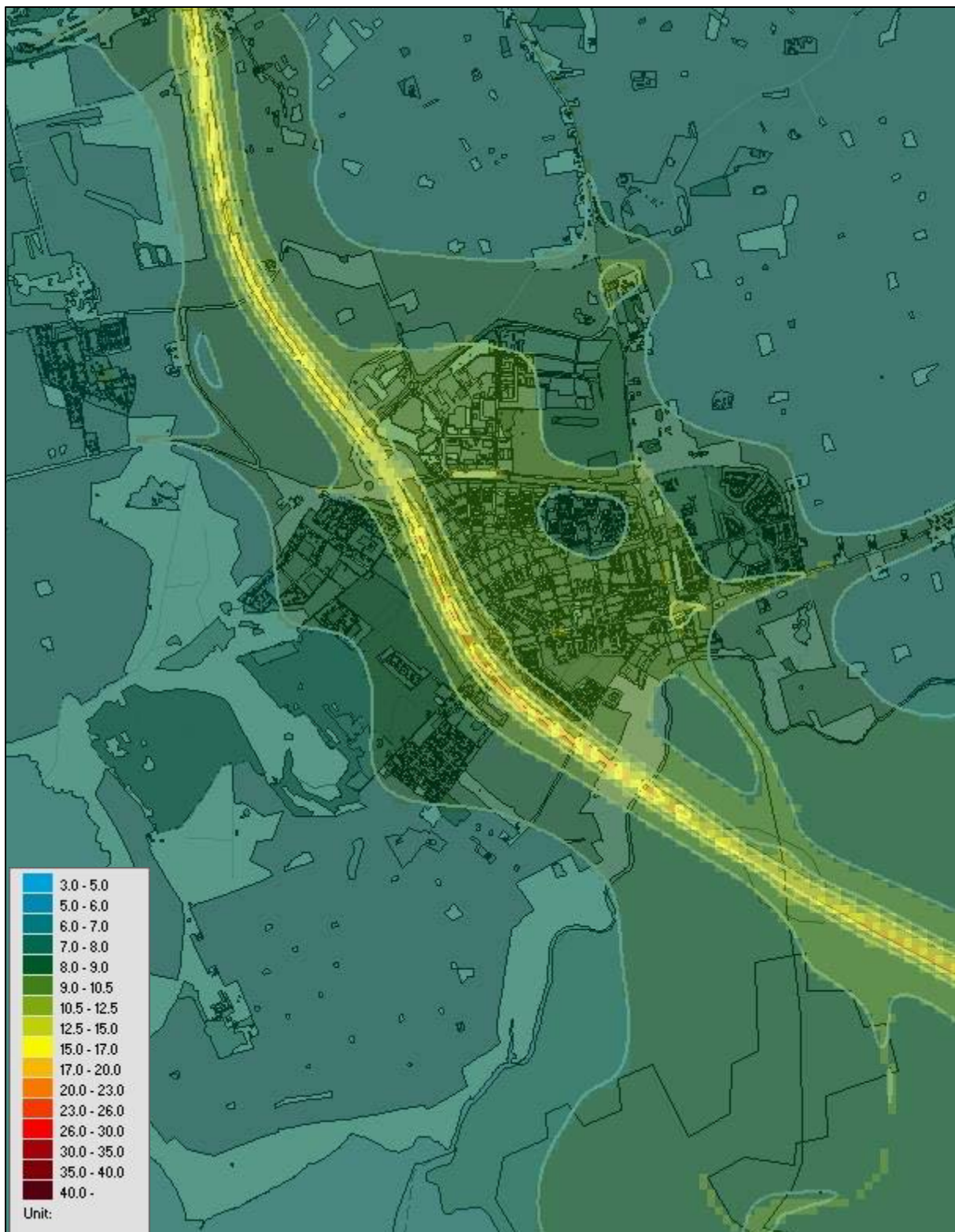
Figur 5. Beräknade årsmedelvärden av kvävedioxid i tätorten Löddeköpinge ( \mu\text{g}/\text{m}^3 ).
