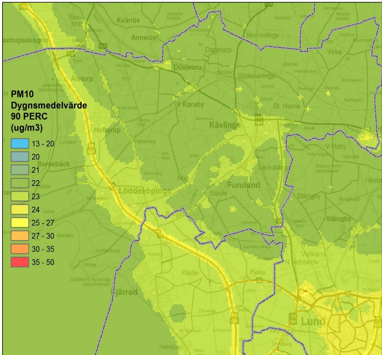
Figur 14. Beräknade dygnsmedelvärden av partiklar PM 10 inom kommunen (µg/m 3 ).
