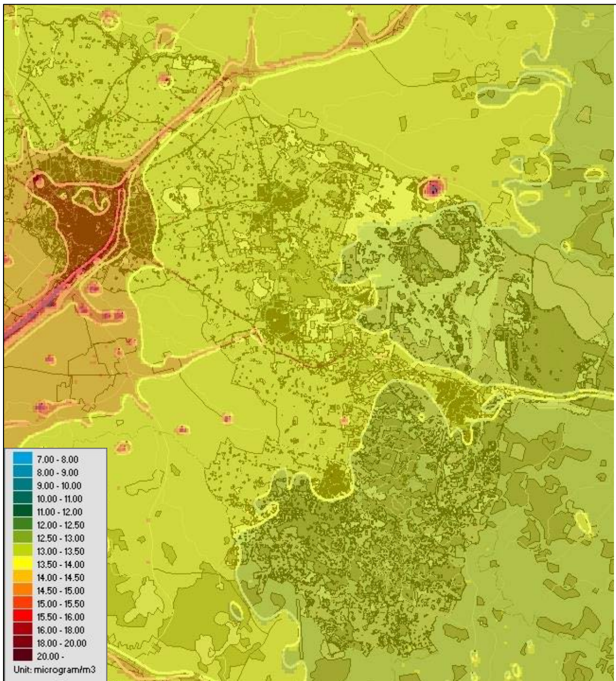
Figur 13. Beräknade årsmedelvärden av partiklar PM_{10} inom kommunen ( \mu\text{g}/\text{m}^3 ).
