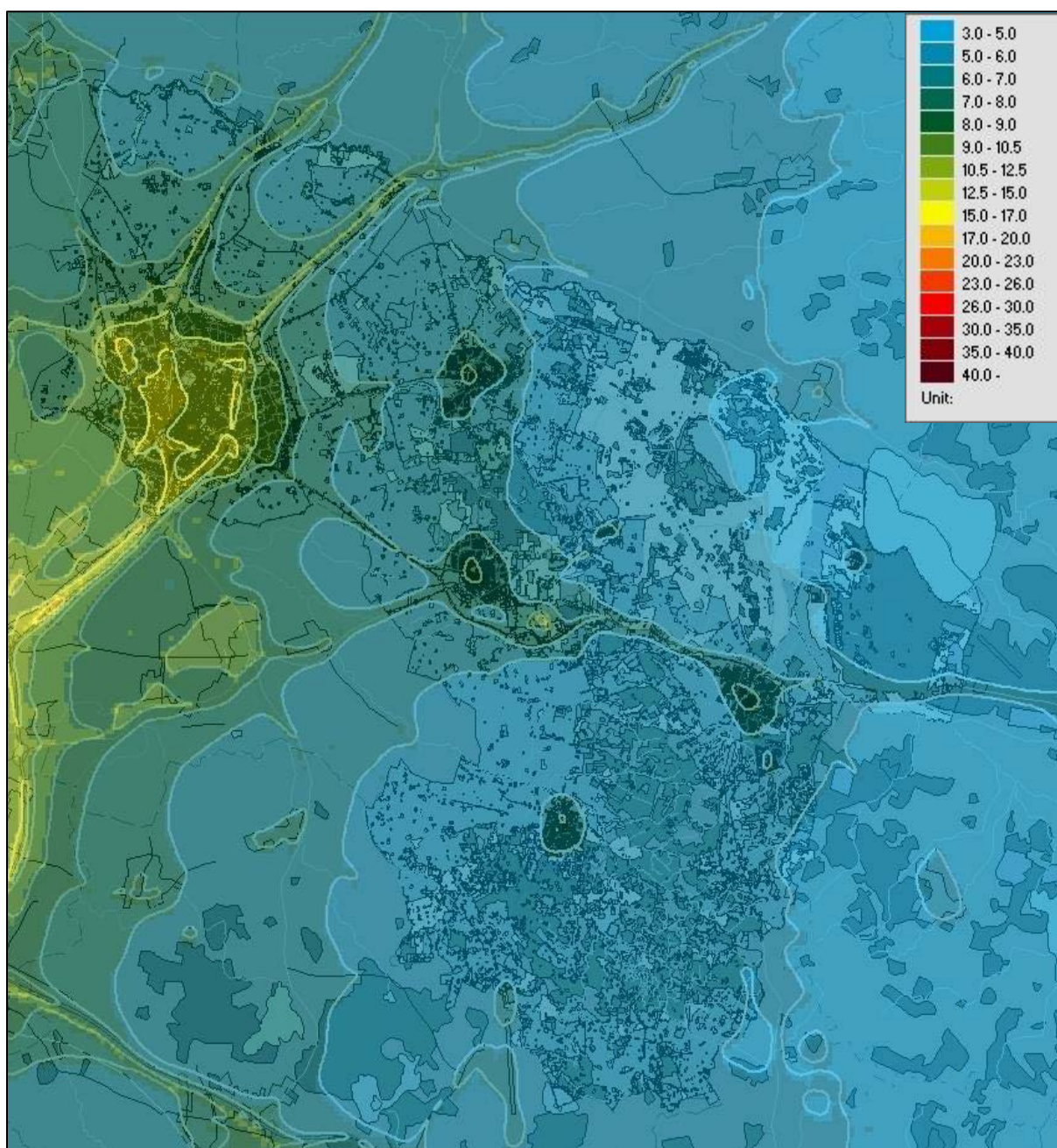
Figur 5. Beräknade årsmedelvärden av kvävedioxid inom kommunen (µg/m 3 ).
