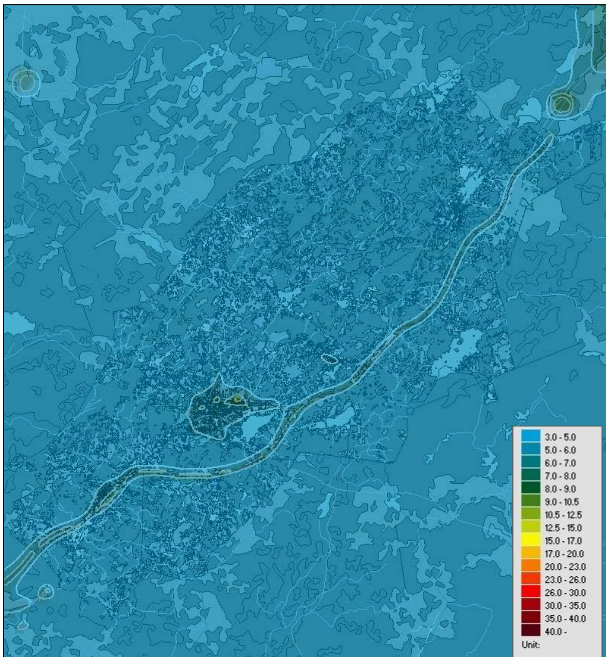
Figur 4. Beräknade årsmedelvärden av kvävedioxid inom kommunen ( \mu\text{g}/\text{m}^3 ).
