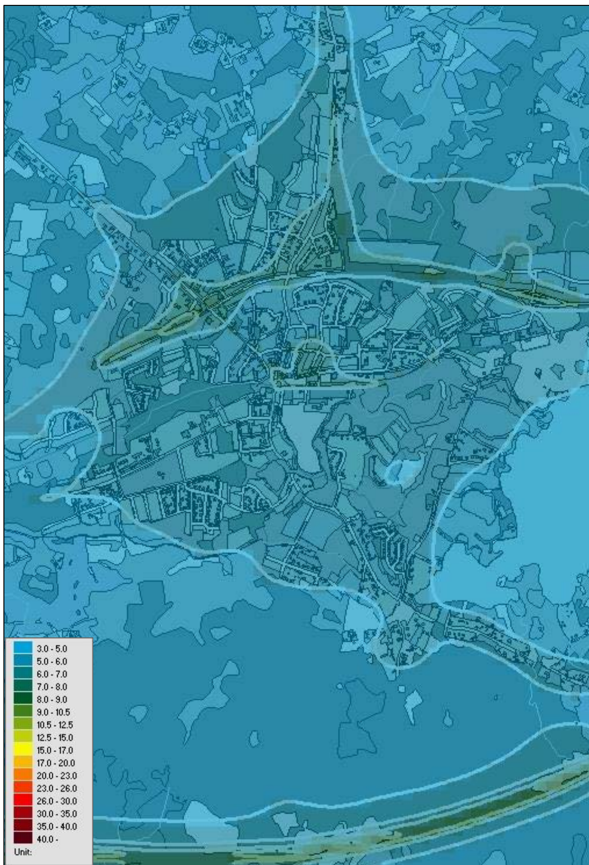
Figur 5. Beräknade årsmedelvärden av kvävedioxid i tätorten (µg/m 3 ).
