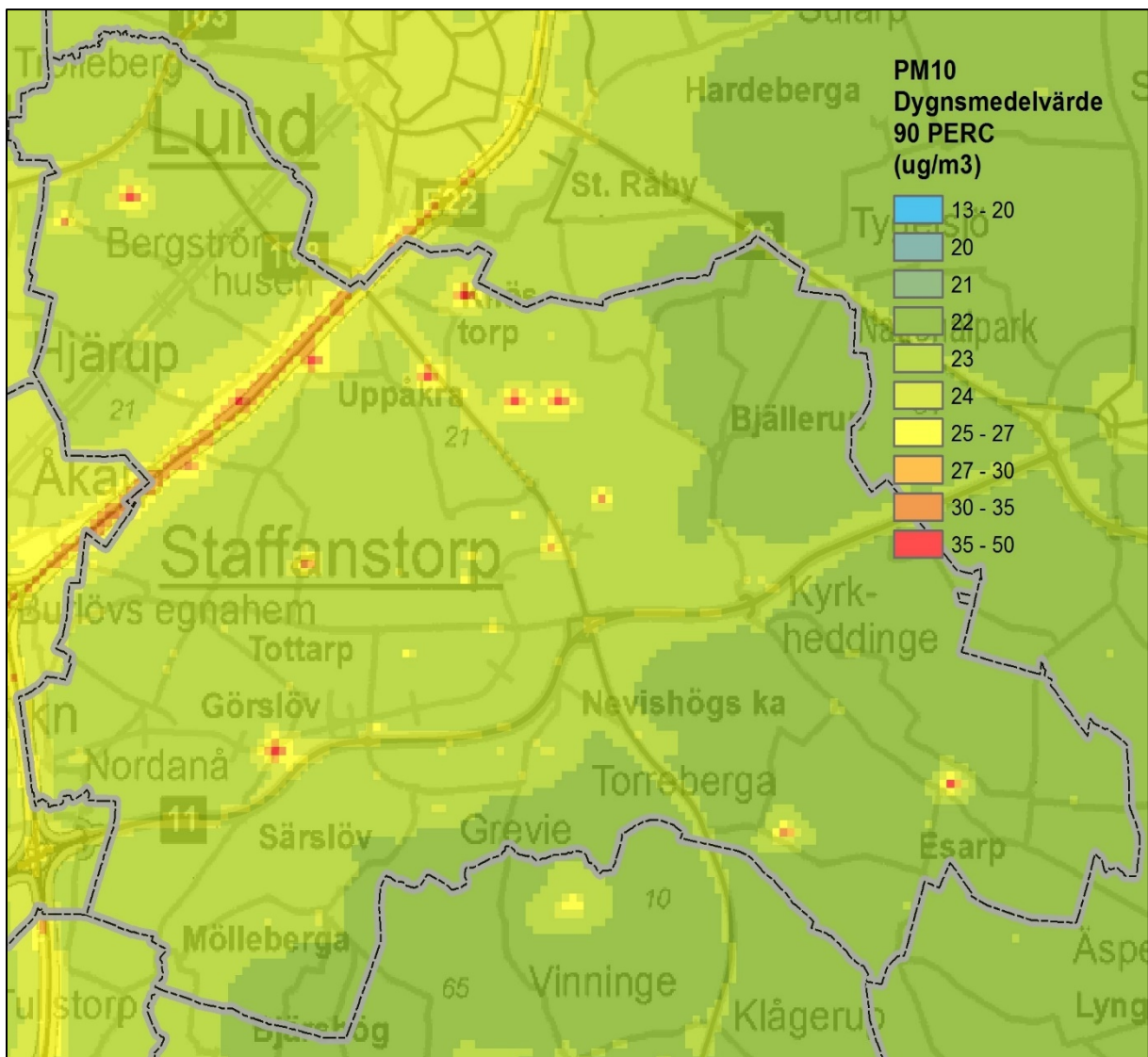
Figur 14. Beräknade dygnsmedelvärden av partiklar PM_{10} inom kommunen ( \mu\text{g}/\text{m}^3 ).
