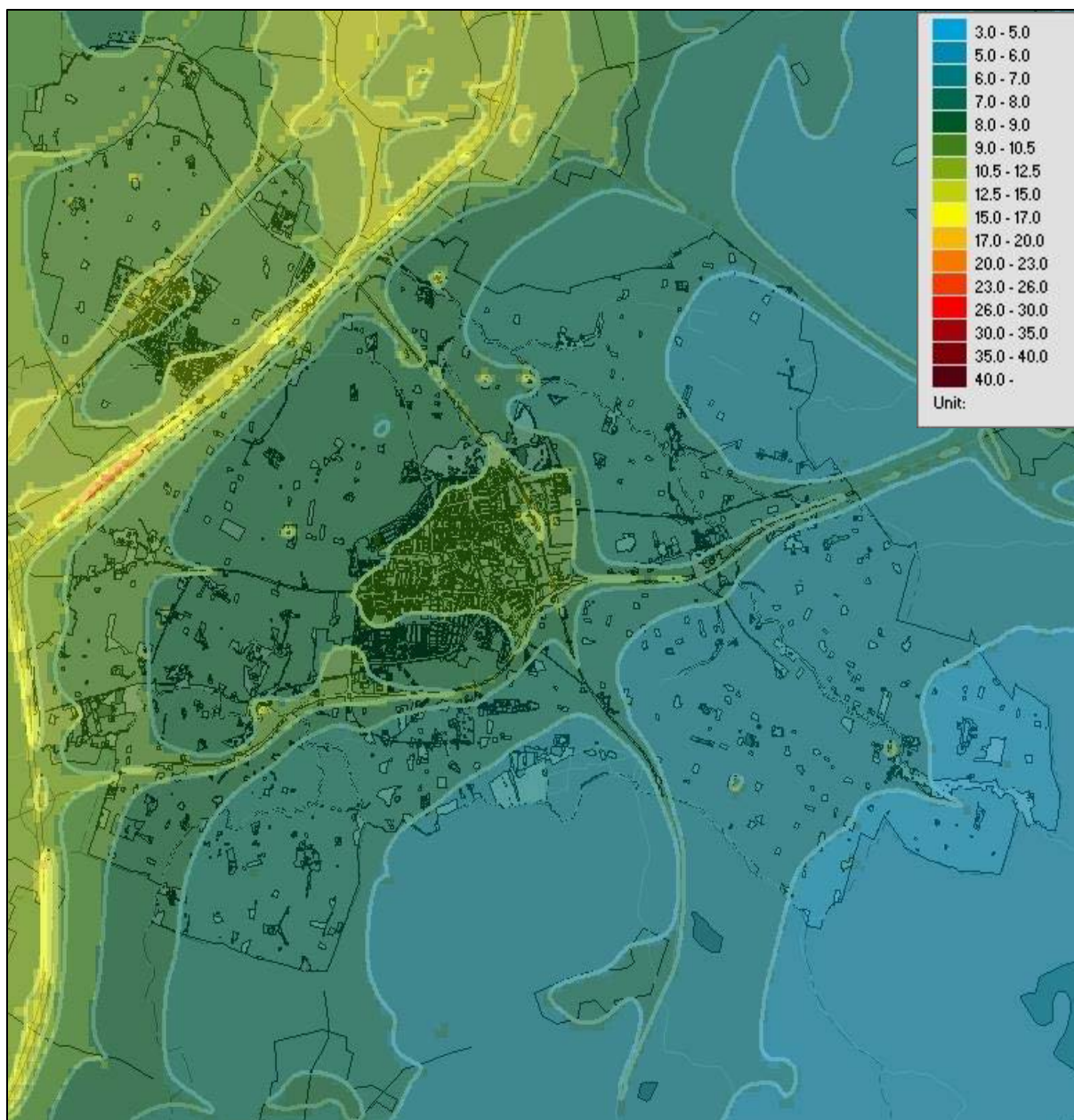
Figur 5. Beräknade årsmedelvärden av kvävedioxid inom kommunen (µg/m 3 ).
