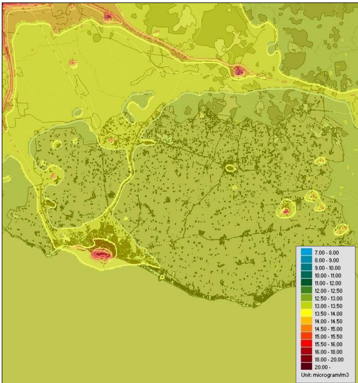
Figur 13. Beräknade årsmedelvärden av partiklar PM 10 inom kommunen (µg/m 3 ).
