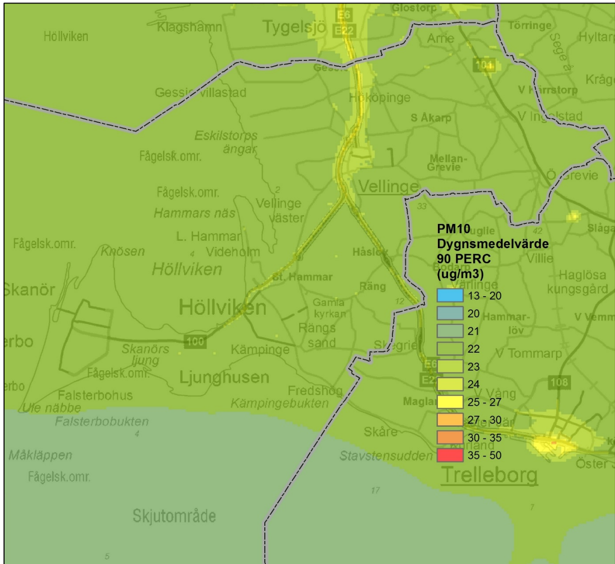
Figur 14. Beräknade dygnsmedelvärden av partiklar PM 10 inom kommunen (µg/m 3 ).
