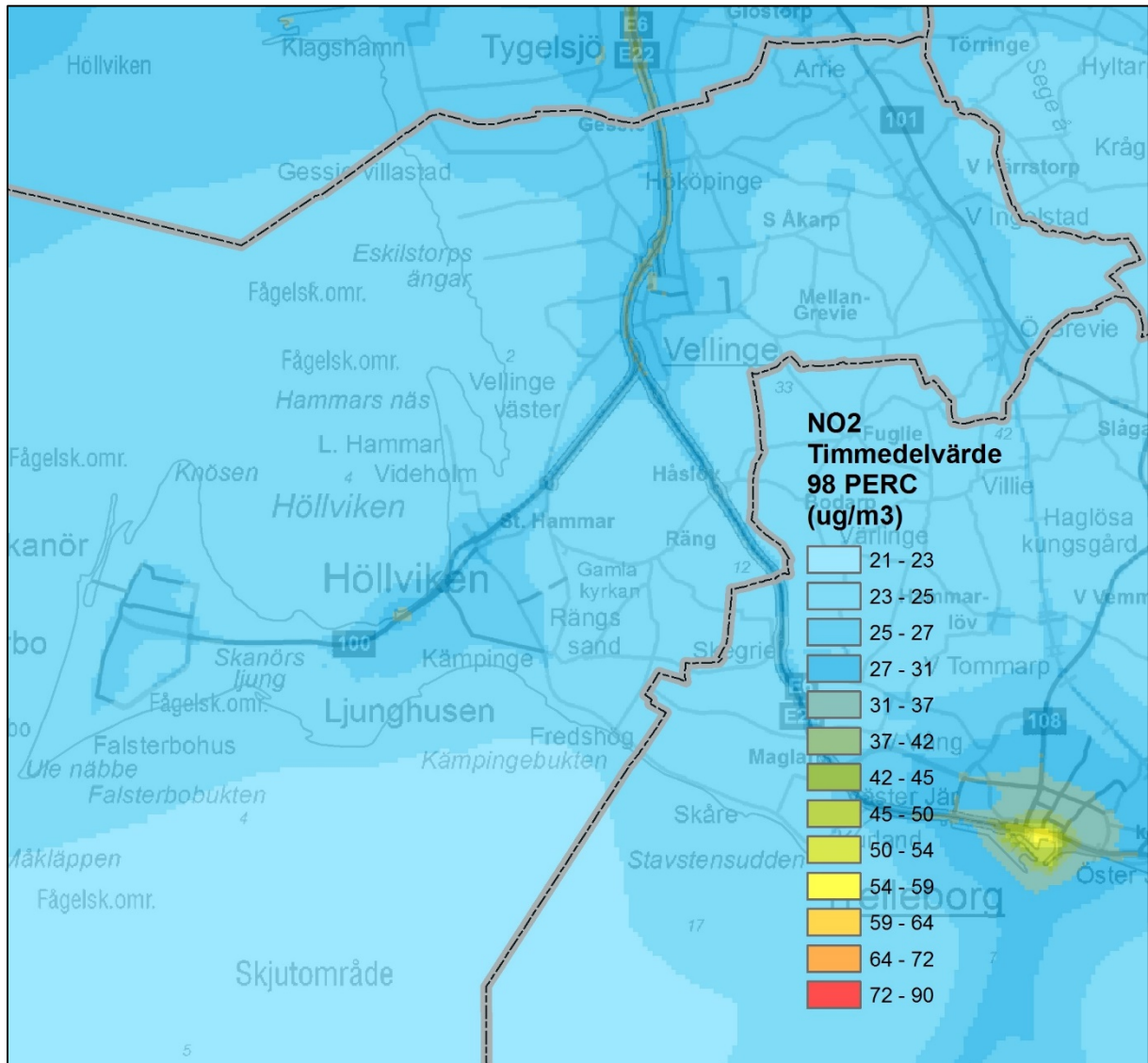
Figur 8. Beräknade timmedelvärderna av kvävedioxid inom kommunen ( \mu\text{g}/\text{m}^3 ).
