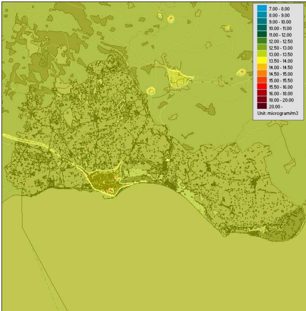
Figur 13. Beräknade årsmedelvärden av partiklar PM 10 inom kommunen (µg/m 3 ).
