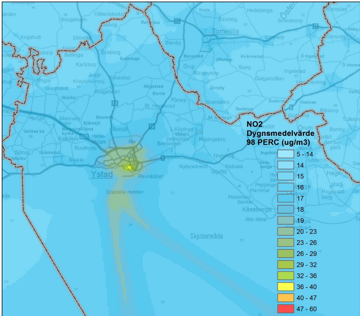
Figur 6. Beräknade dygnsmedelvärden av kvävedioxid inom kommunen ( \mu\text{g}/\text{m}^3 ).
