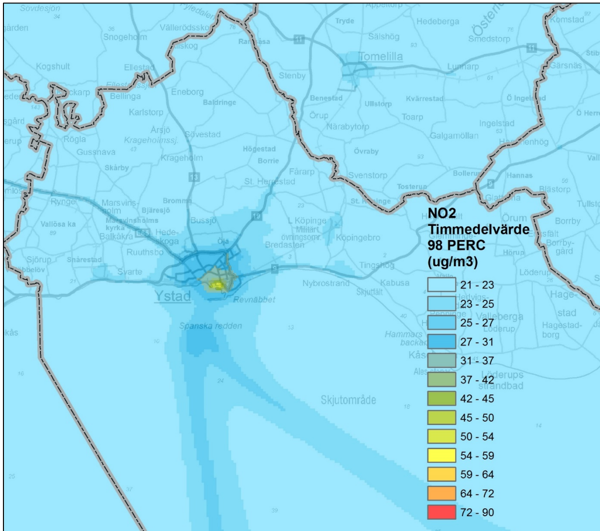
Figur 8. Beräknade timmedelvärden av kvävedioxid inom kommunen ( \mu\text{g}/\text{m}^3 ).
