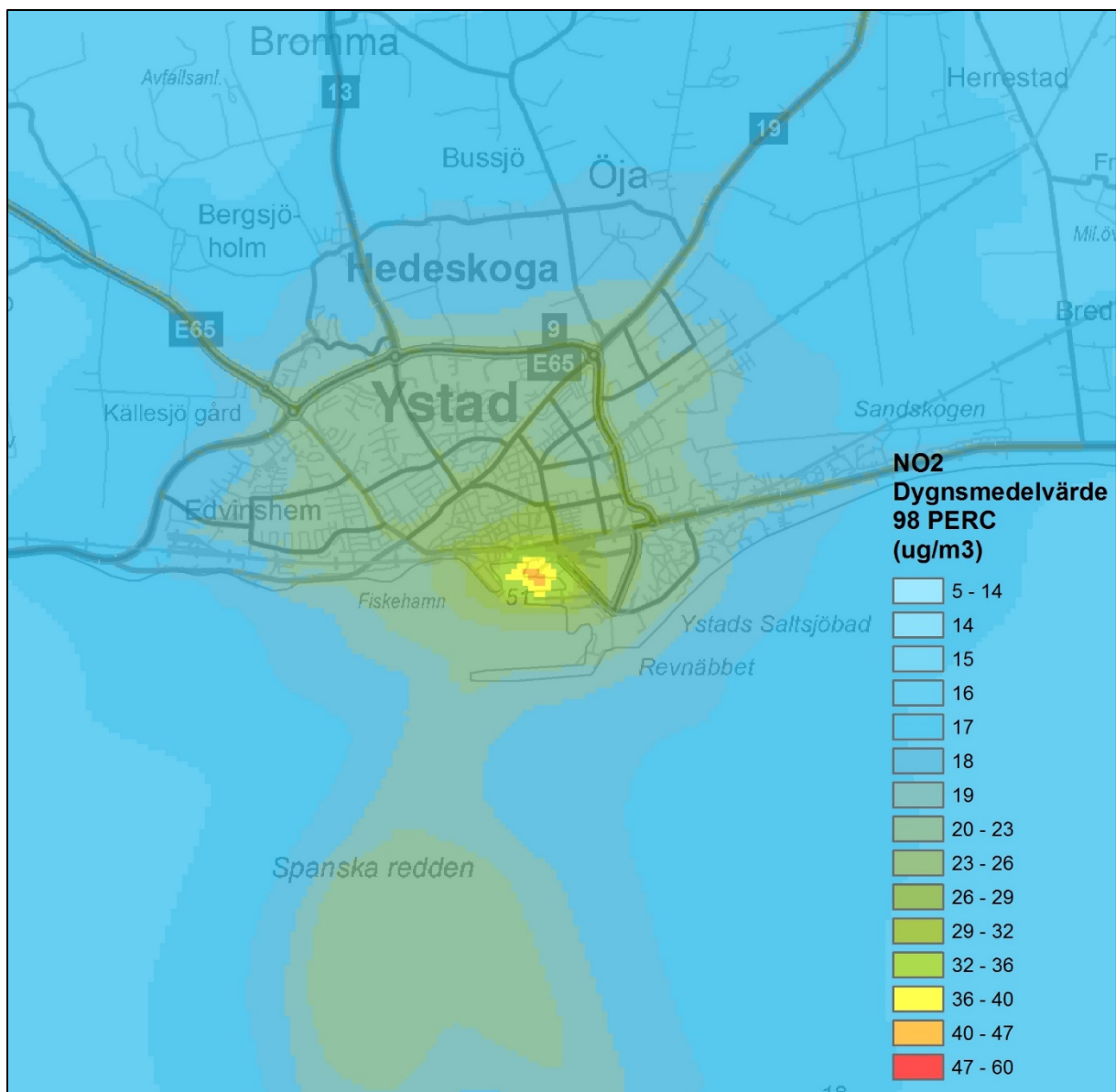
Figur 7. Beräknade dygnsnivåer av kvävedioxid i tätorten ( \mu\text{g}/\text{m}^3 ).
