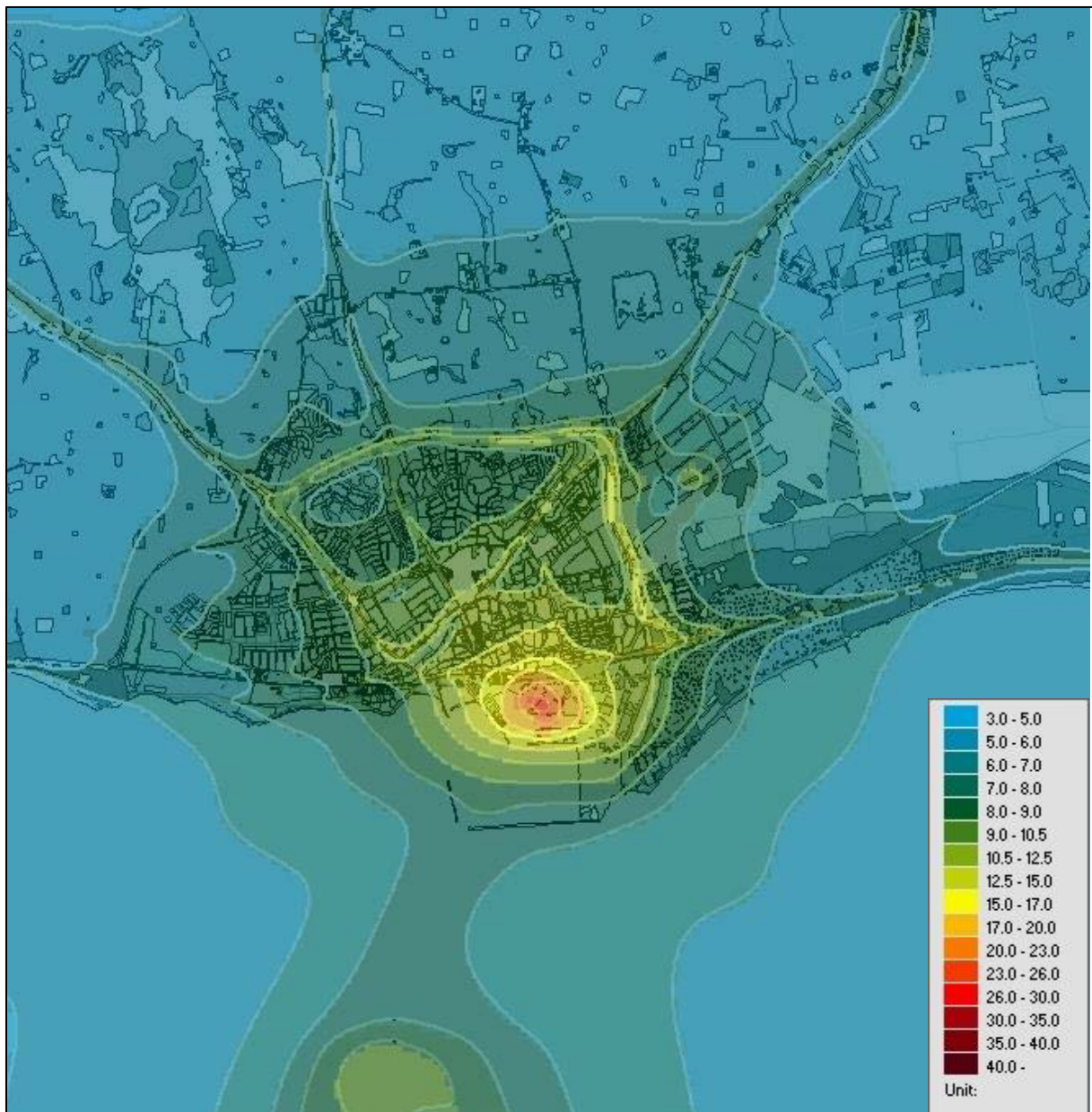
Figur 4. Beräknade årsmedelvärden av kvävedioxid i tätorten ( \mu\text{g}/\text{m}^3 ).
