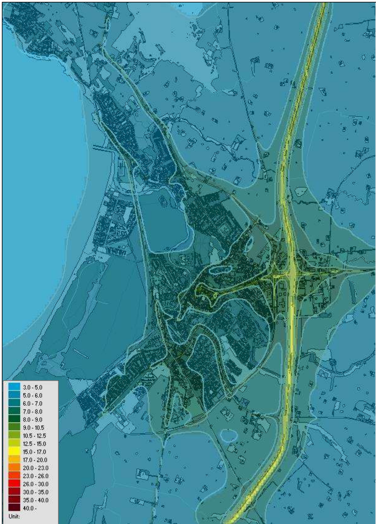
Figur 5. Beräknade årsmedelvärden av kvävedioxid i tätorten ( \mu\text{g}/\text{m}^3 ).
