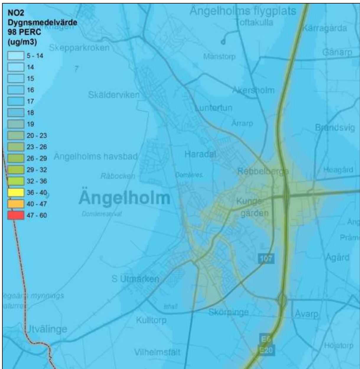
Figur 7. Beräknade dygnsnedelvärden av kvävedioxid i tätorten ( \mu\text{g}/\text{m}^3 ).
