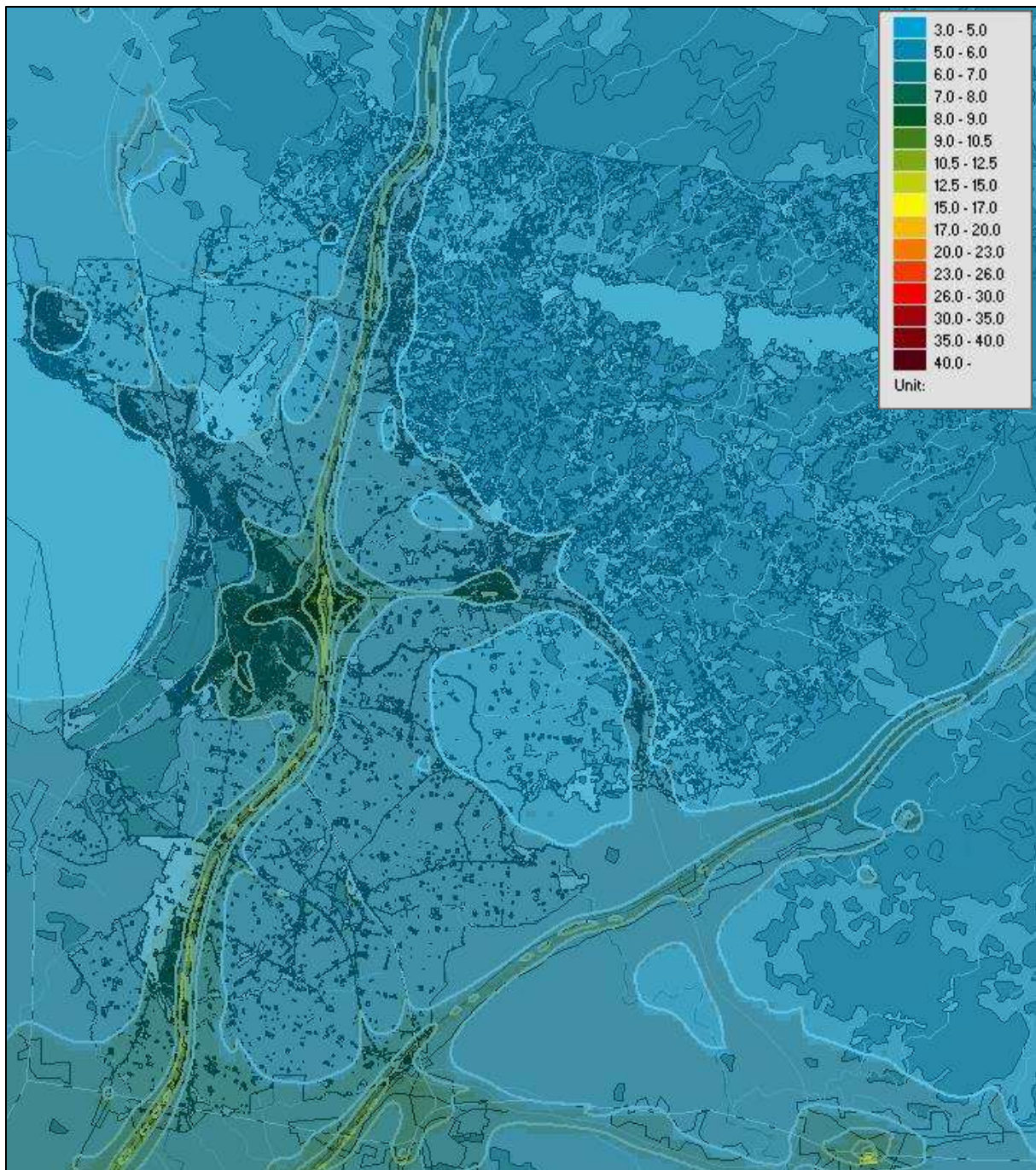
Figur 4. Beräknade årsmedelvärden av kvävedioxid inom kommunen ( \mu\text{g}/\text{m}^3 ).
