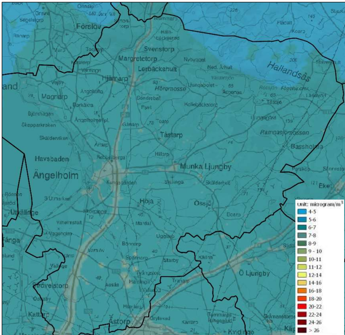
Figur 19. Beräknade årsmedelvärden av partiklar PM 2,5 inom kommunen (µg/m 3 ).
