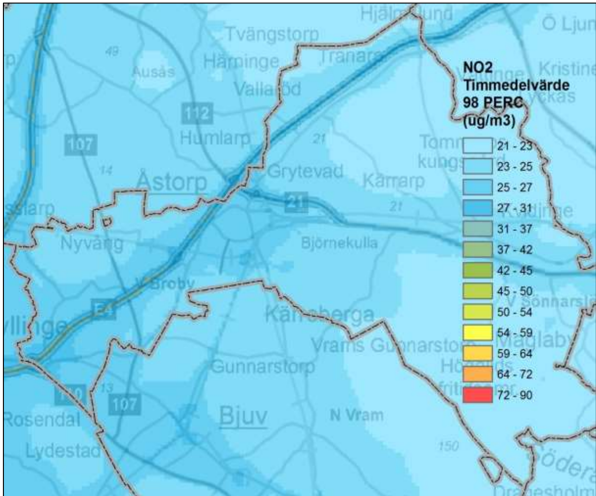
Figur 8. Beräknade timmedelvärden av kvävedioxid inom kommunen ( \mu\text{g}/\text{m}^3 ).
