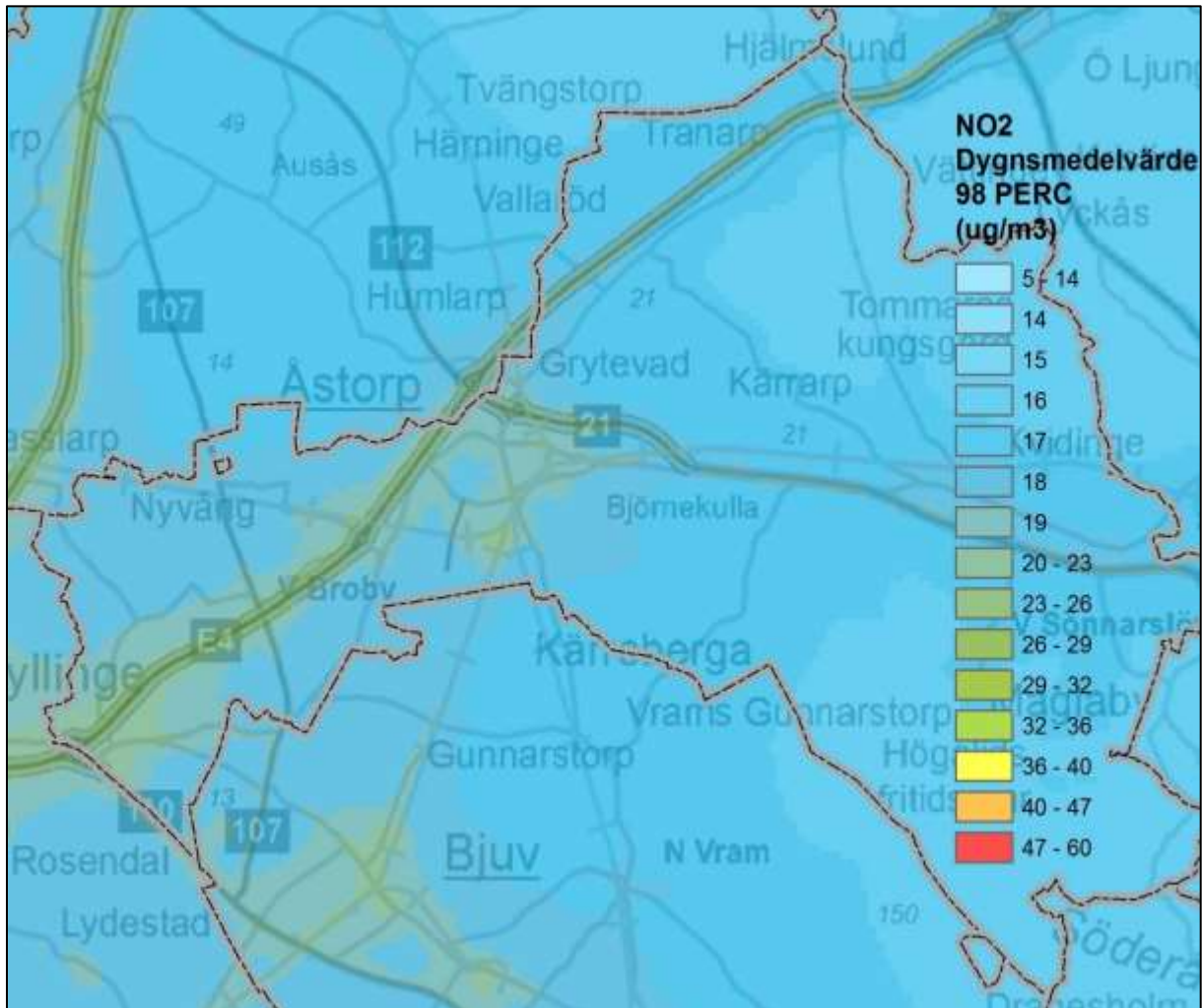
Figur 6. Beräknade dygnsmedelvärden av kvävedioxid inom kommunen ( \mu\text{g}/\text{m}^3 ).
