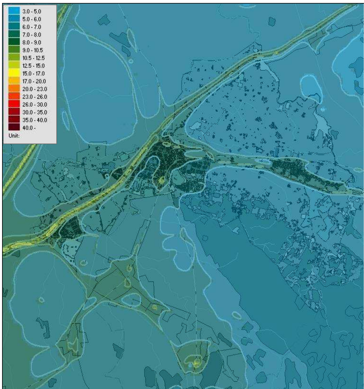
Figur 5. Beräknade årsmedelvärden av kvävedioxid inom kommunen ( \mu\text{g}/\text{m}^3 ).
