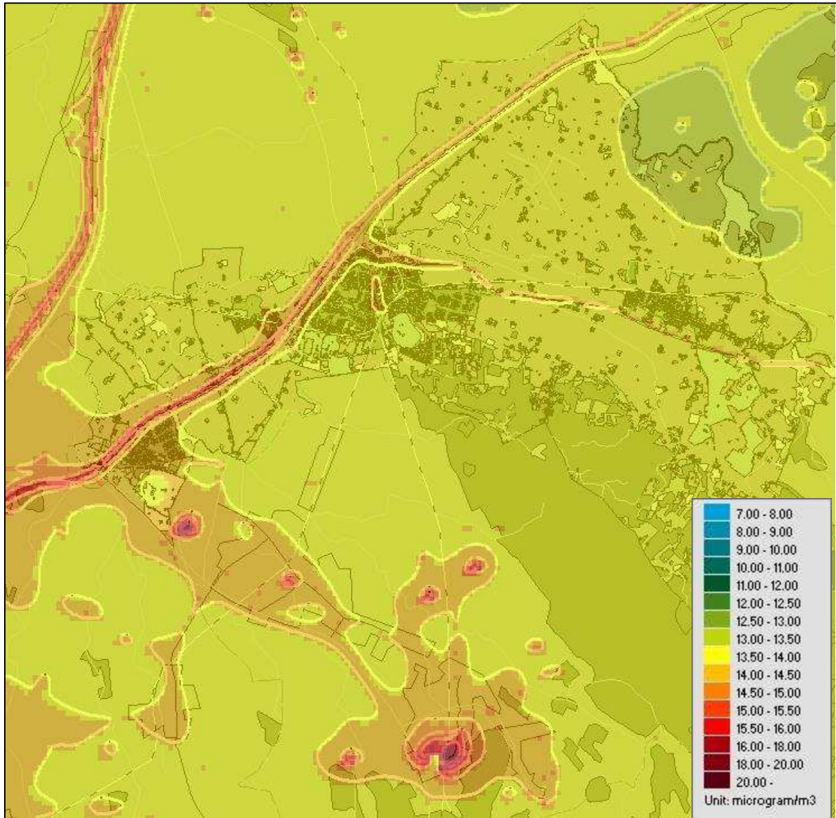
Figur 14. Beräknade årsmedelvärden av partiklar PM 10 inom kommunen (µg/m 3 ).
