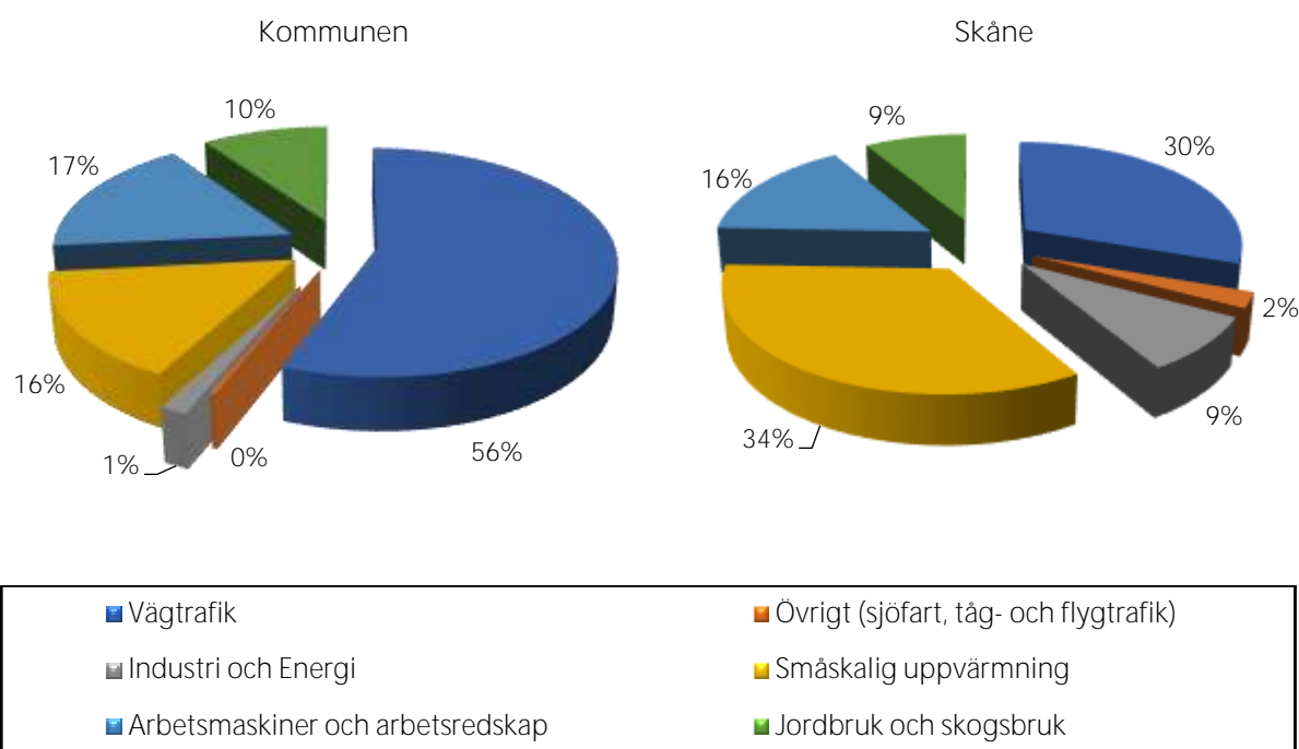
Figur 20. Procentuell fördelning av utsläppskällor för partiklar (PM 2,5 ) i kommunen jämfört med Skåne.
