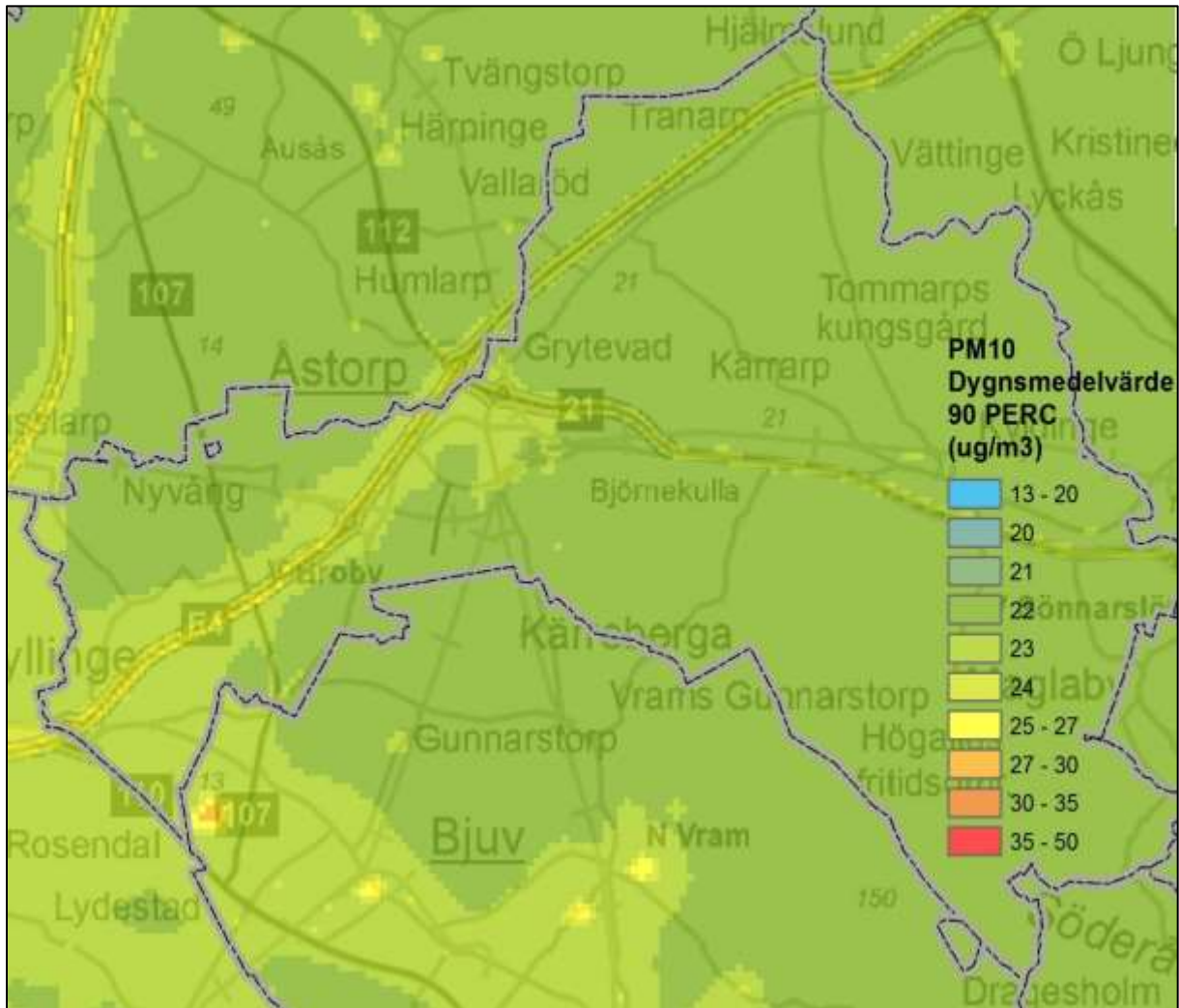
Figur 15. Beräknade dygnsmedelvärden av partiklar PM_{10} inom kommunen ( \mu\text{g}/\text{m}^3 ).
