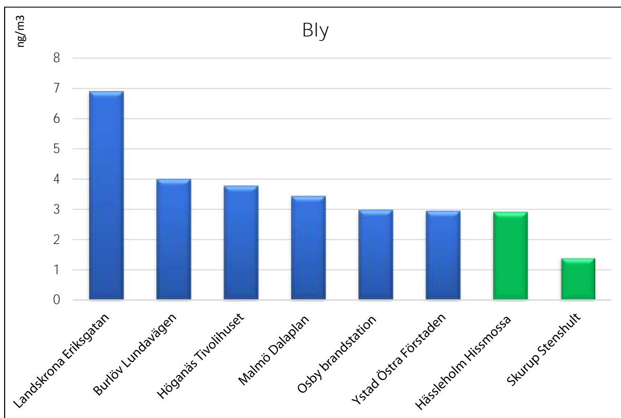
Figur 27. Medelvärdet för Bly (Pb) under mätperioden inom samverkansområdet Skåne.
