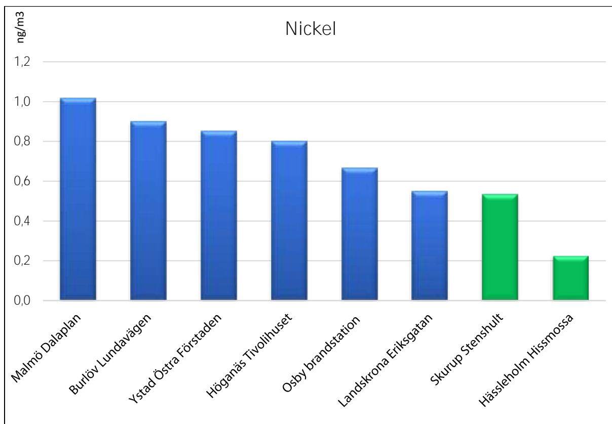
Figur 26. Medelvärdet för Nickel (Ni) under mätperioden inom samverkansområdet Skåne.
