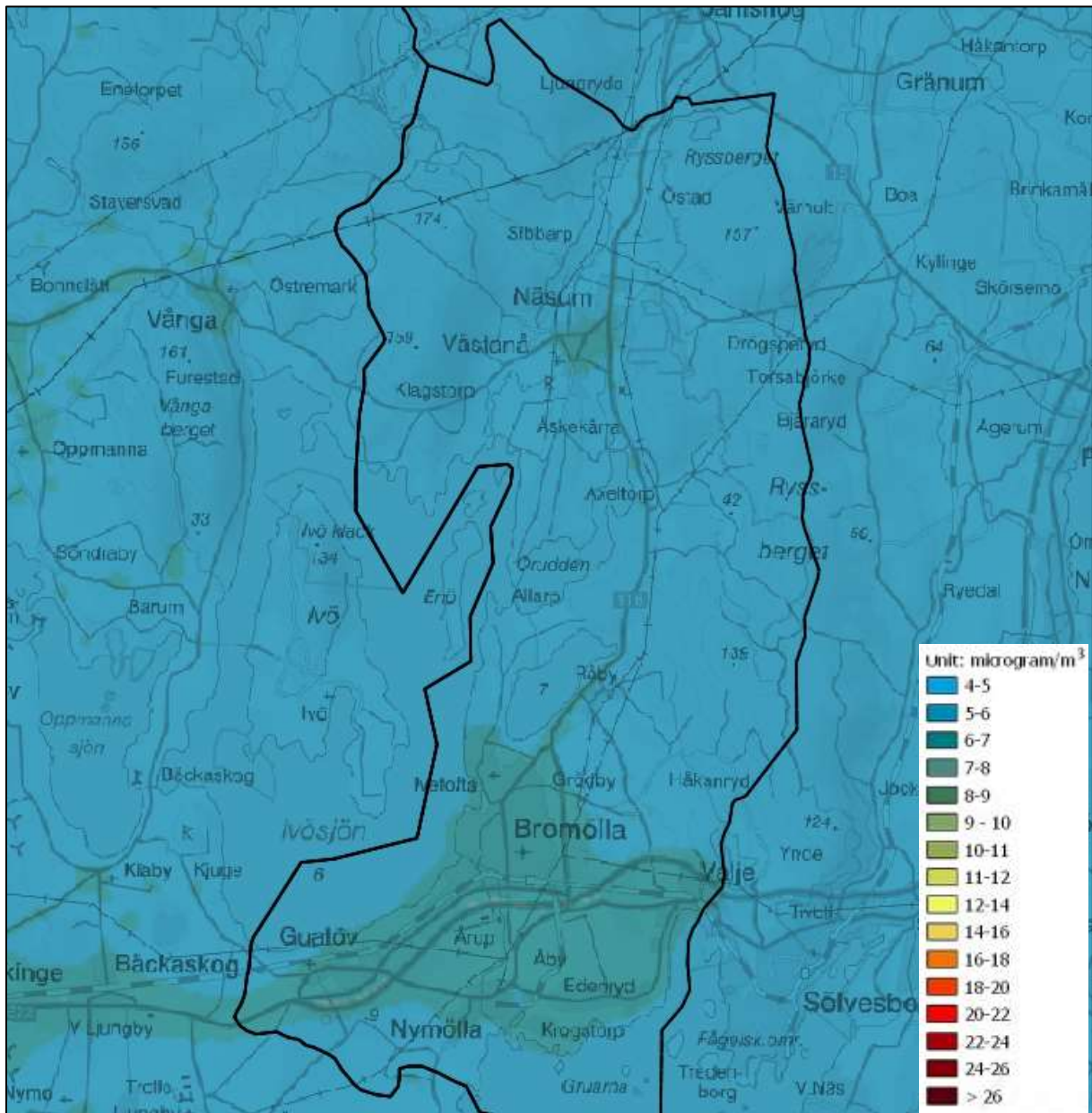
Figur 19. Beräknade årsmedelvärden av partiklar PM 2,5 inom kommunen (µg/m 3 ).
