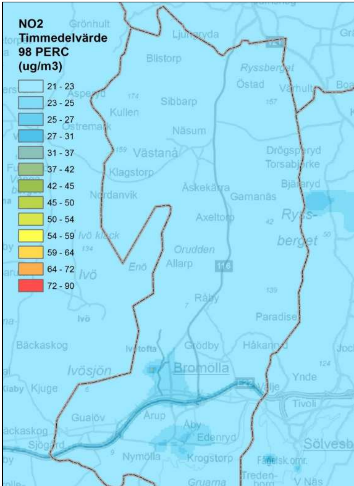
Figur 8. Beräknade timmedelvärden av kvävedioxid inom kommunen ( \mu\text{g}/\text{m}^3 ).
