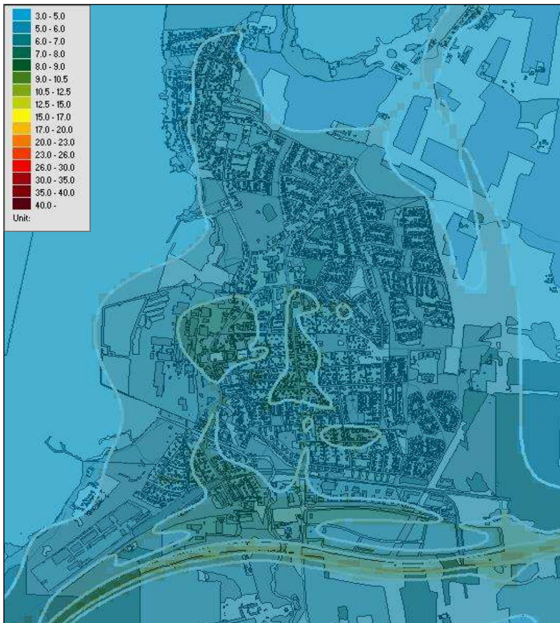
Figur 4. Beräknade årsmedelvärden av kvävedioxid i tätorten ( \mu\text{g}/\text{m}^3 ).
