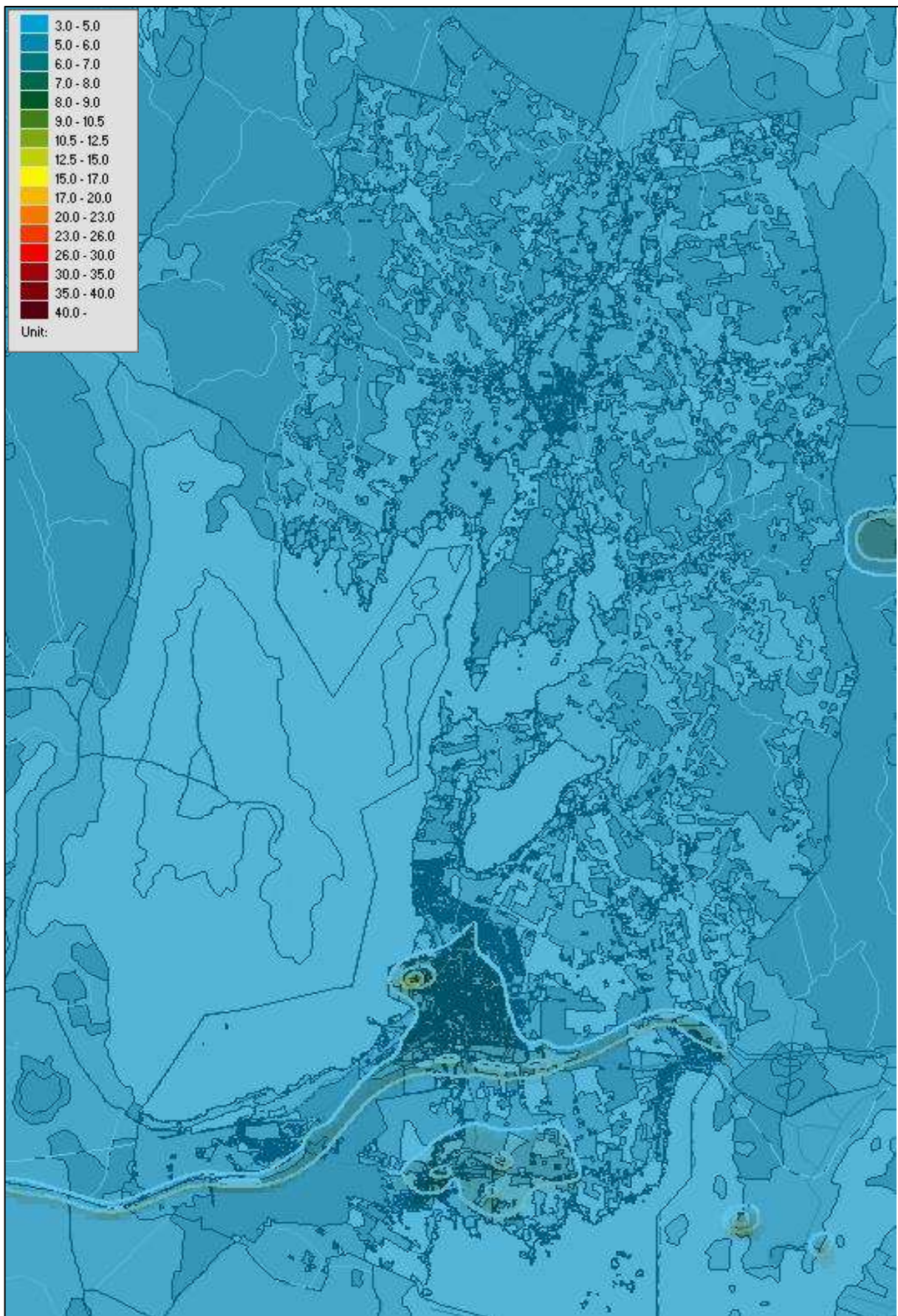
Figur 5. Beräknade årsmedelvärden av kvävedioxid inom kommunen ( \mu\text{g}/\text{m}^3 ).
