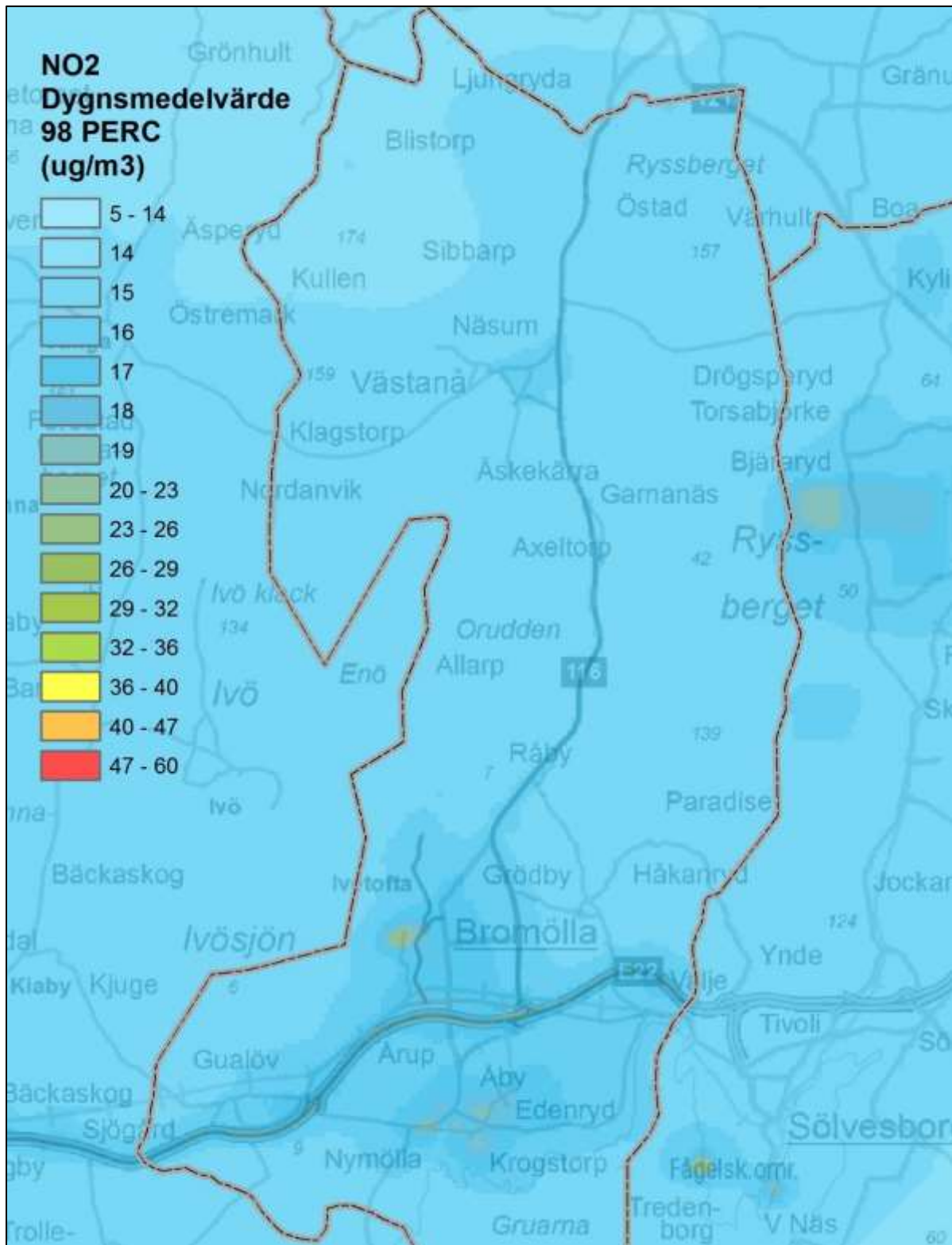
Figur 6. Beräknade dygnsmedelvärden av kvävedioxid inom kommunen ( \mu\text{g}/\text{m}^3 ).
