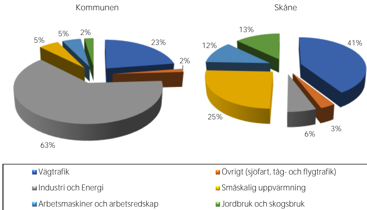
Figur 16. Procentuell fördelning av utsläppskällor för partiklar (PM 10 ) i kommunen jämfört med Skåne.
