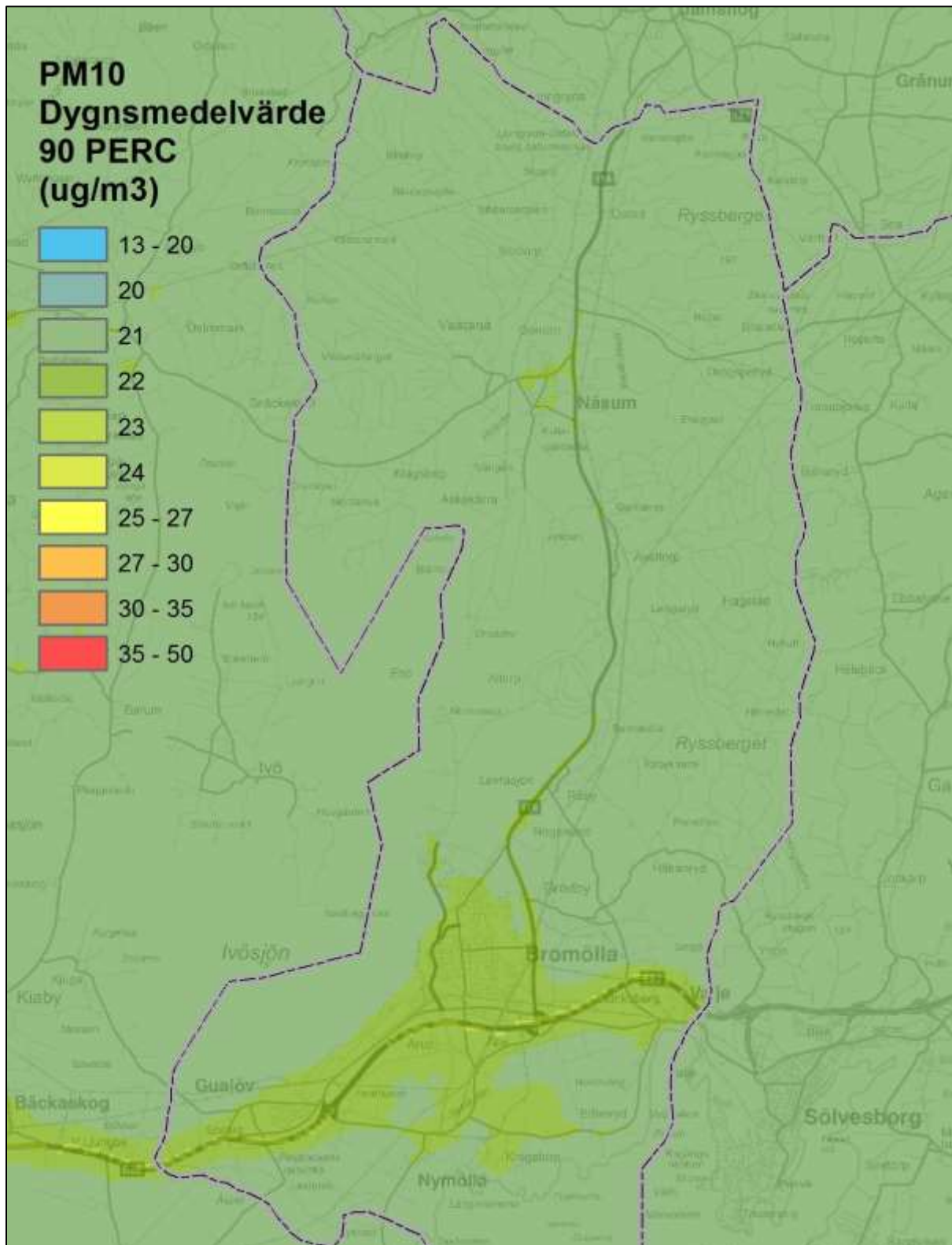
Figur 15. Beräknade dygnsmedelvärden av partiklar PM 10 inom kommunen (µg/m 3 ).
