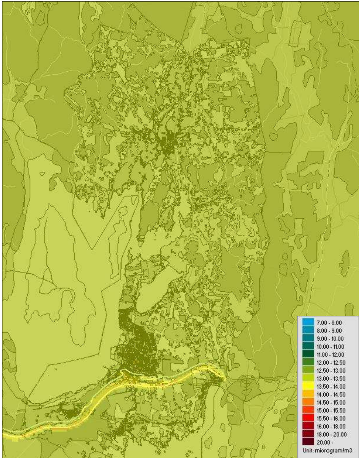
Figur 14. Beräknade årsmedelvärden av partiklar PM 10 inom kommunen (µg/m 3 ).
