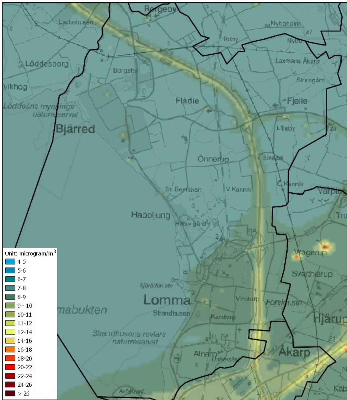
Figur 19. Beräknade årsmedelvärden av partiklar PM_{2,5} inom kommunen ( \mu\text{g}/\text{m}^3 ).
