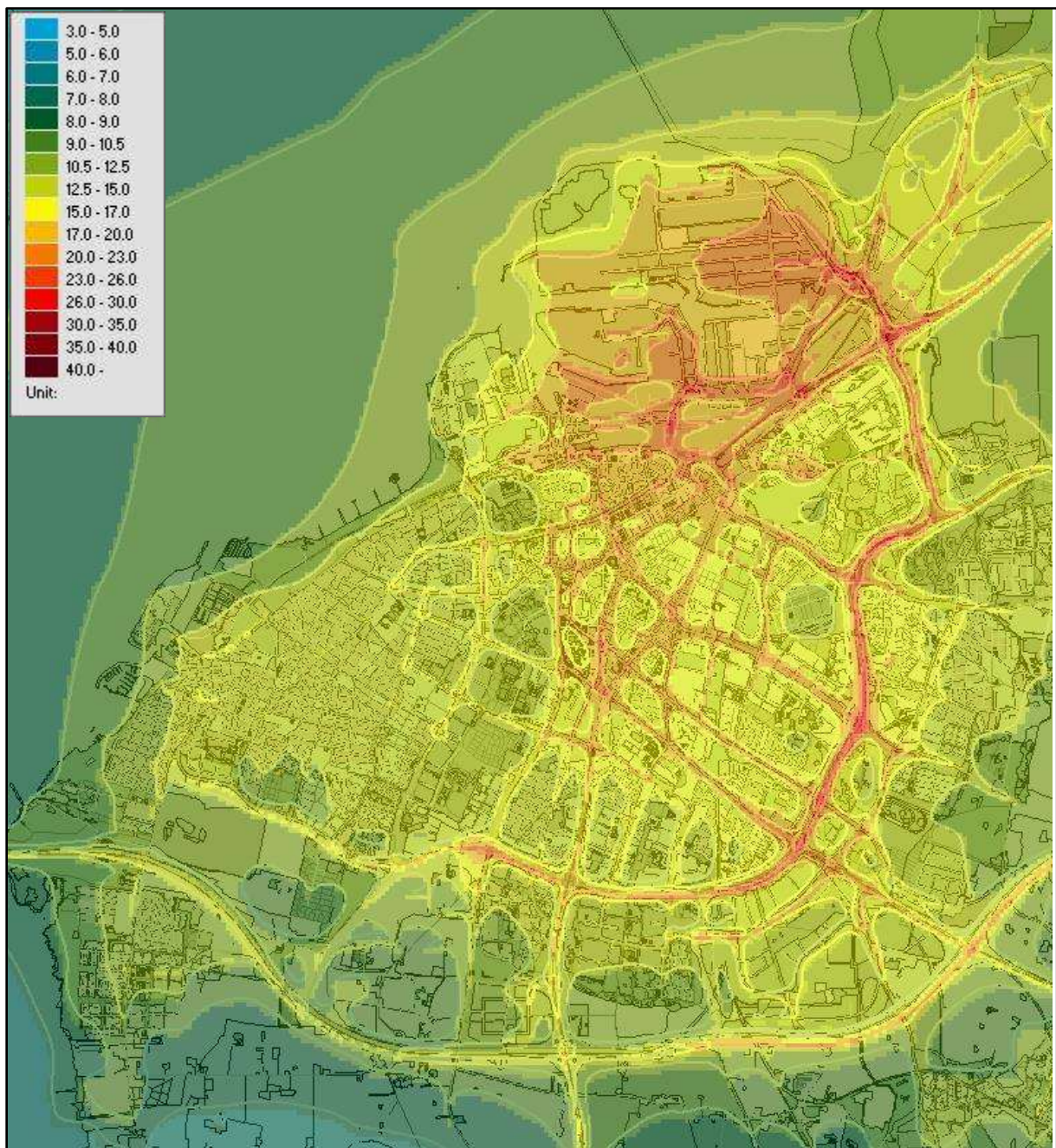
Figur 4. Beräknade årsmedelvärden av kvävedioxid i tätorten Malmö ( \mu\text{g}/\text{m}^3 ).
