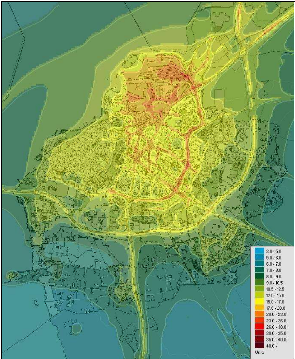
Figur 5. Beräknade årsmedelvärden av kvävedioxid inom kommunen (µg/m 3 ).
