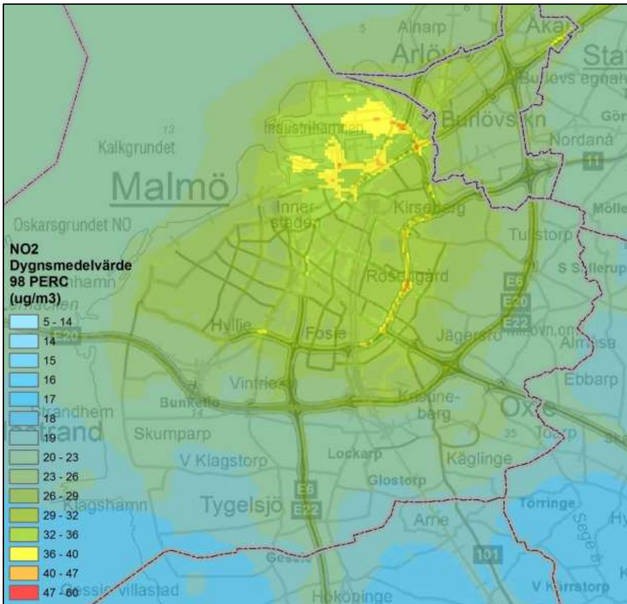
Figur 6. Beräknade dygnsmedelvärden av kvävedioxid inom kommunen ( \mu\text{g}/\text{m}^3 ).
