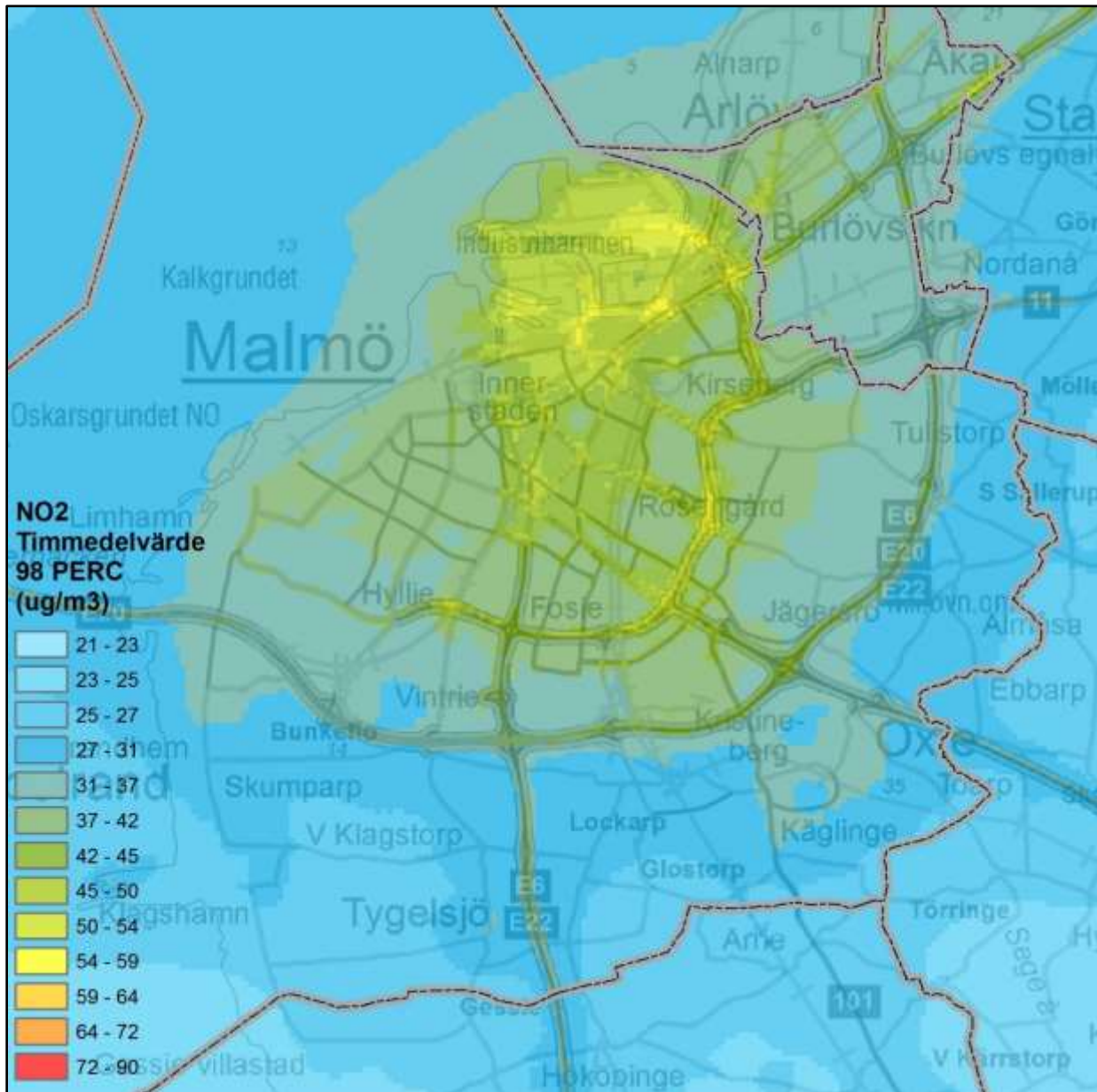
Figur 8. Beräknade timmedelvärden av kvävedioxid inom kommunen ( \mu\text{g}/\text{m}^3 ).
