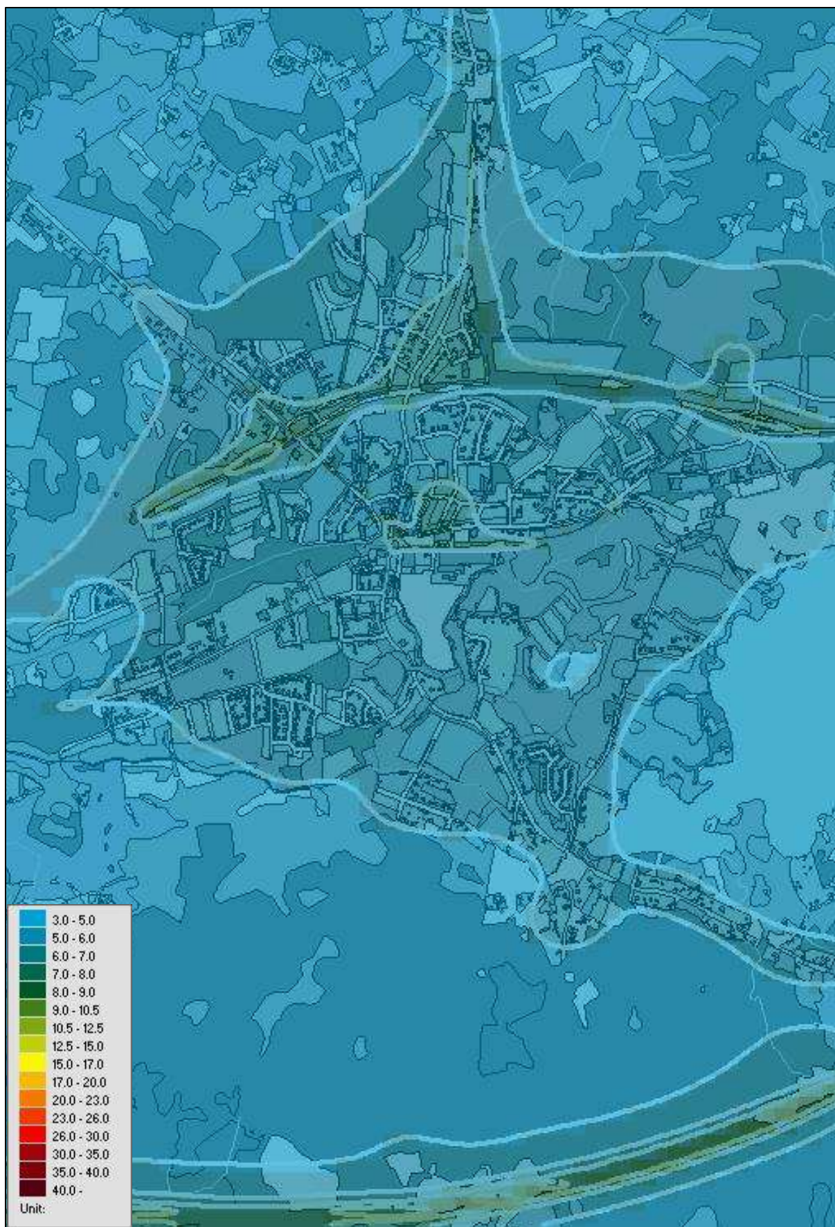
Figur 5. Beräknade årsmedelvärden av kvävedioxid i tätorten ( \mu\text{g}/\text{m}^3 ).
