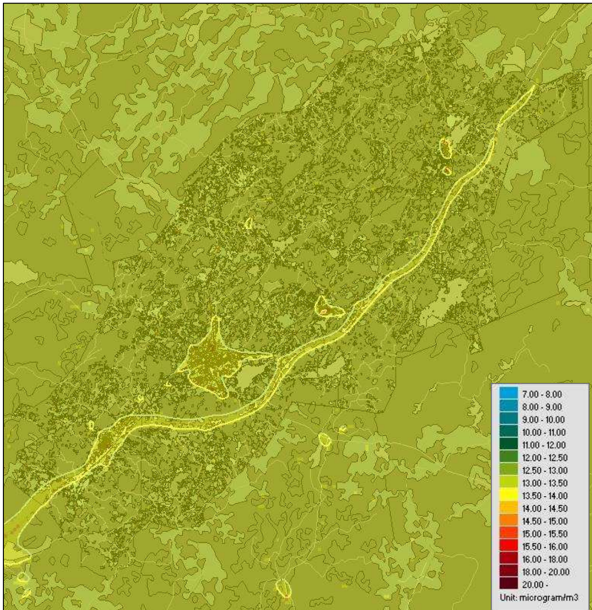
Figur 14. Beräknade årsmedelvärden av partiklar PM 10 inom kommunen (µg/m 3 ).
