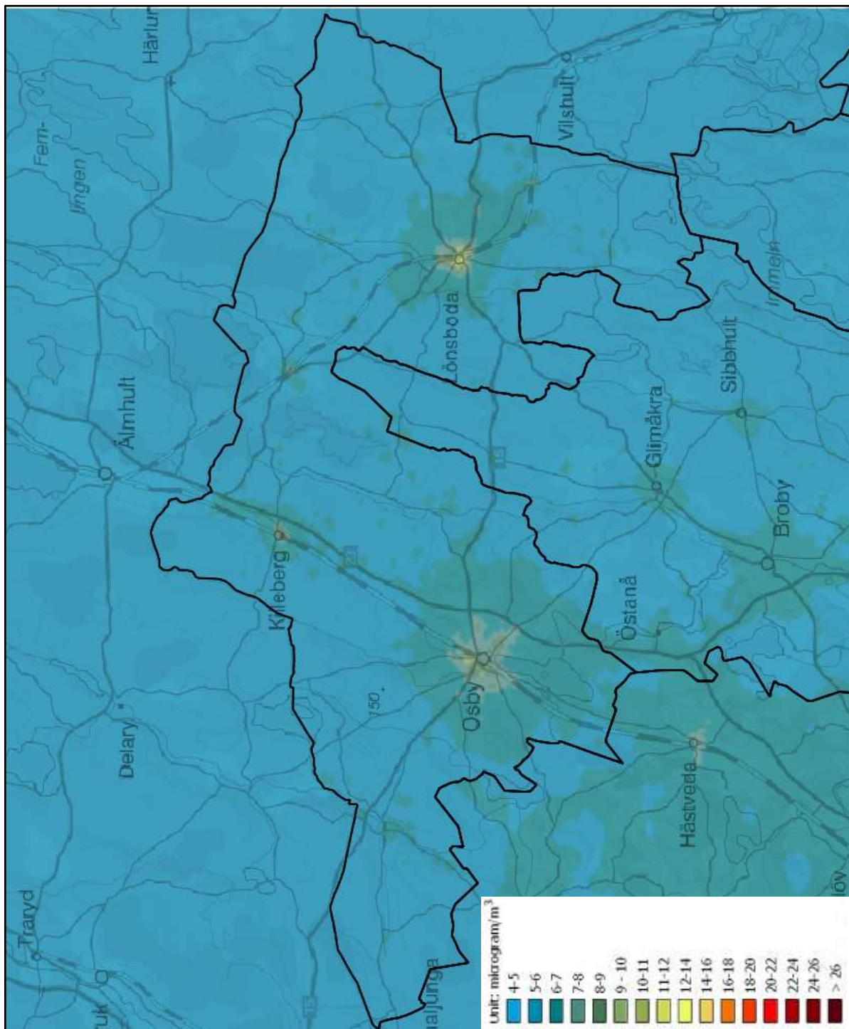
Figur 19. Beräknade årsmedelvärden av partiklar PM 2,5 inom kommunen (µg/m 3 ).
