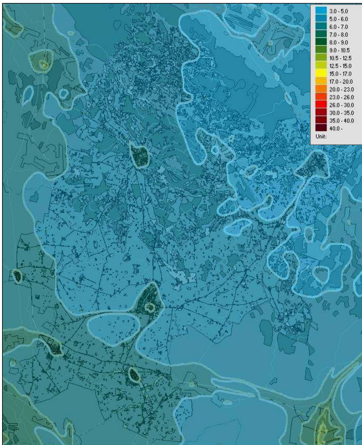
Figur 5. Beräknade årsmedelvärden av kvävedioxid inom kommunen ( \mu\text{g}/\text{m}^3 ).
