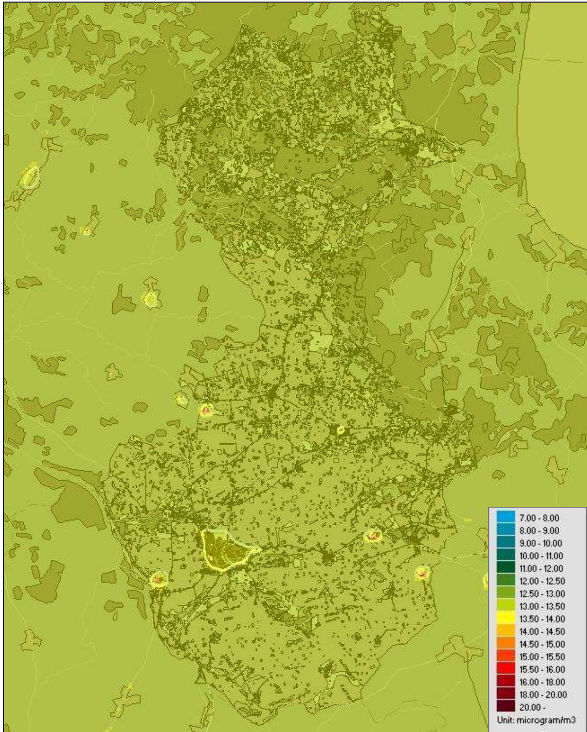
Figur 14. Beräknade årsmedelvärden av partiklar PM_{10} inom kommunen ( \mu\text{g}/\text{m}^3 ).
