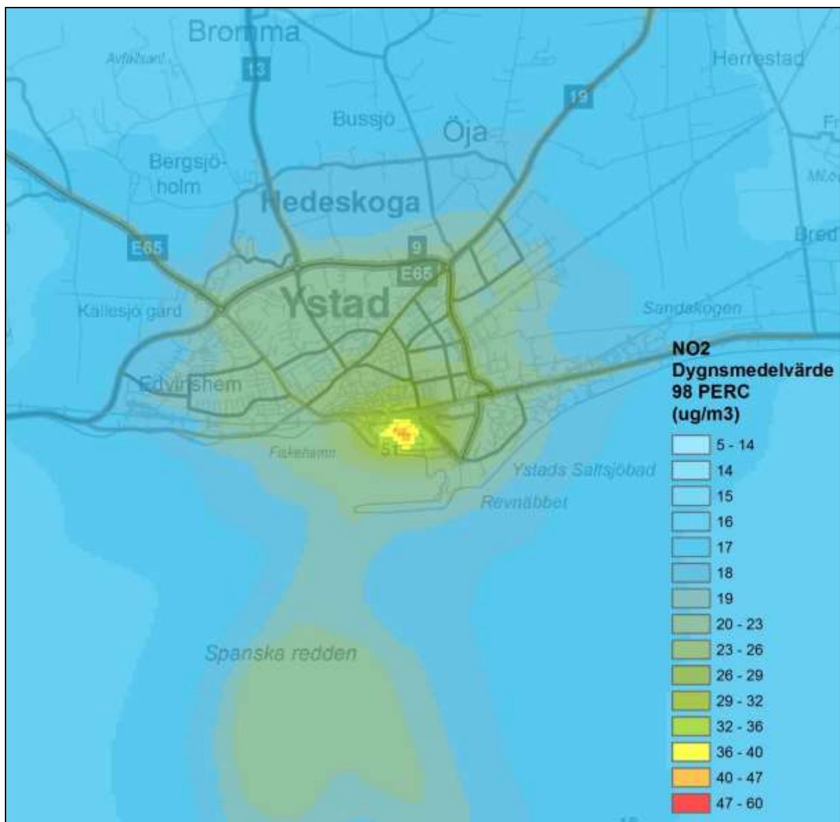
Figur 7. Beräknade dygnsmedelvärden av kvävedioxid i tätorten ( \mu\text{g}/\text{m}^3 ).
