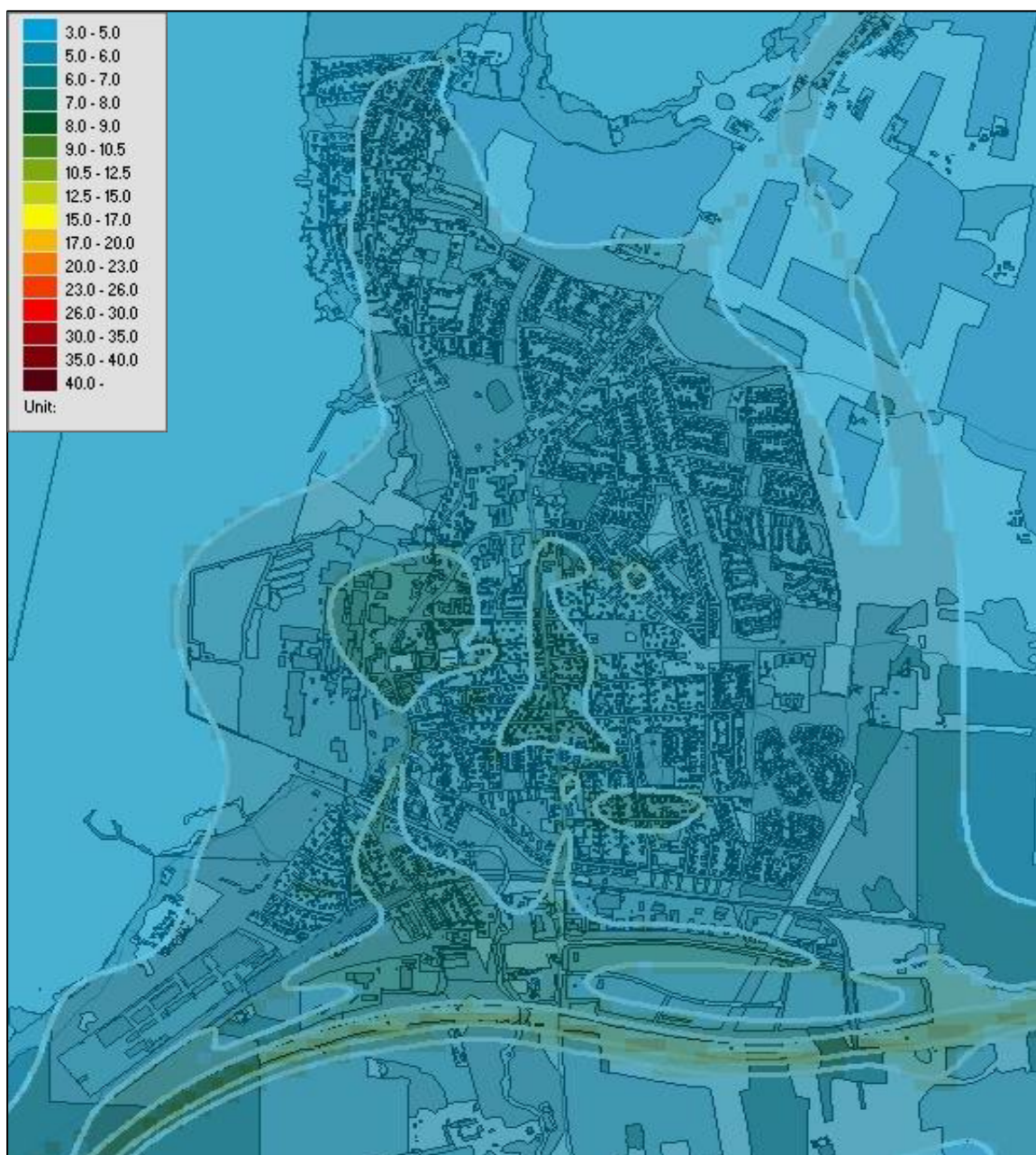
Figur 6. Beräknade årsmedelvärden av kvävedioxid i tätorten ( \mu\text{g}/\text{m}^3 ).
