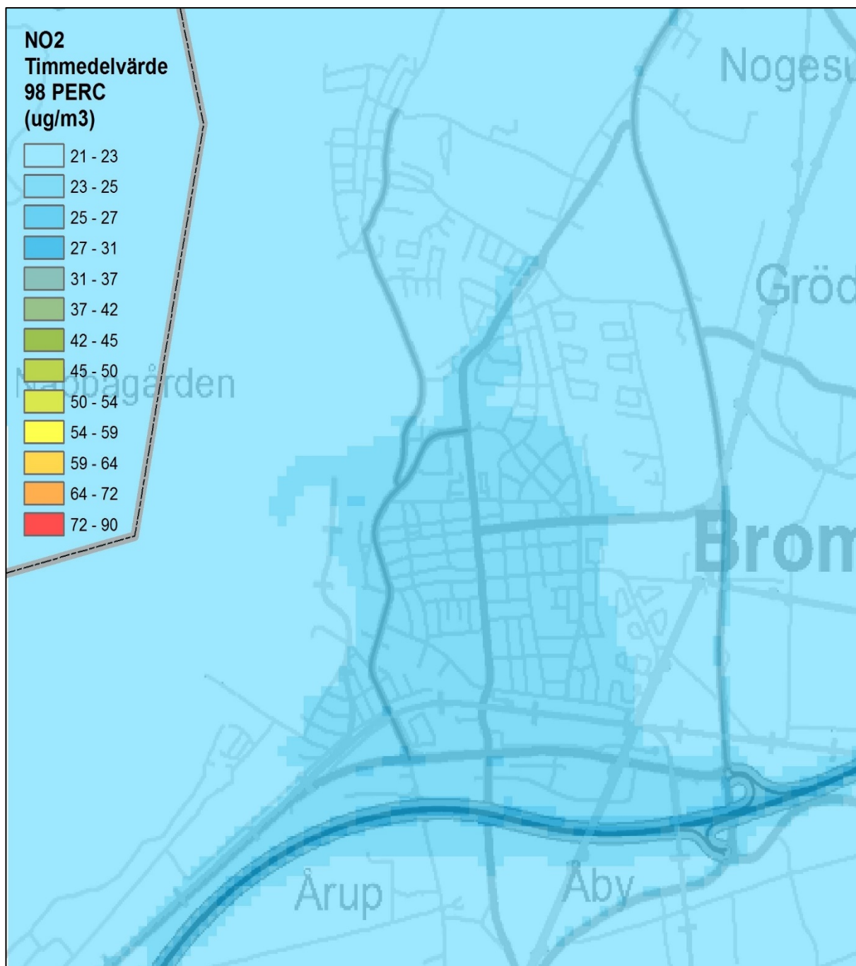
Figur 11. Beräknade timmedelvärden av kvävedioxid i tätorten ( \mu\text{g}/\text{m}^3 ).
