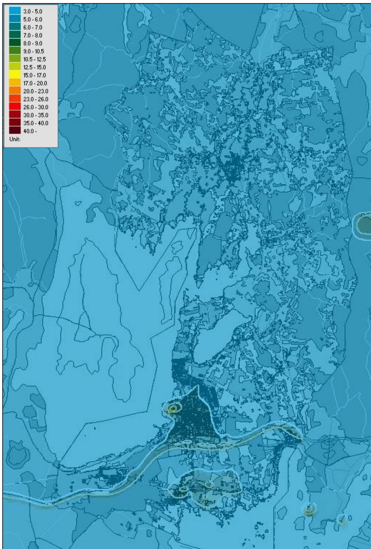
Figur 7. Beräknade årsmedelvärden av kvävedioxid inom kommunen ( \mu\text{g}/\text{m}^3 ).
