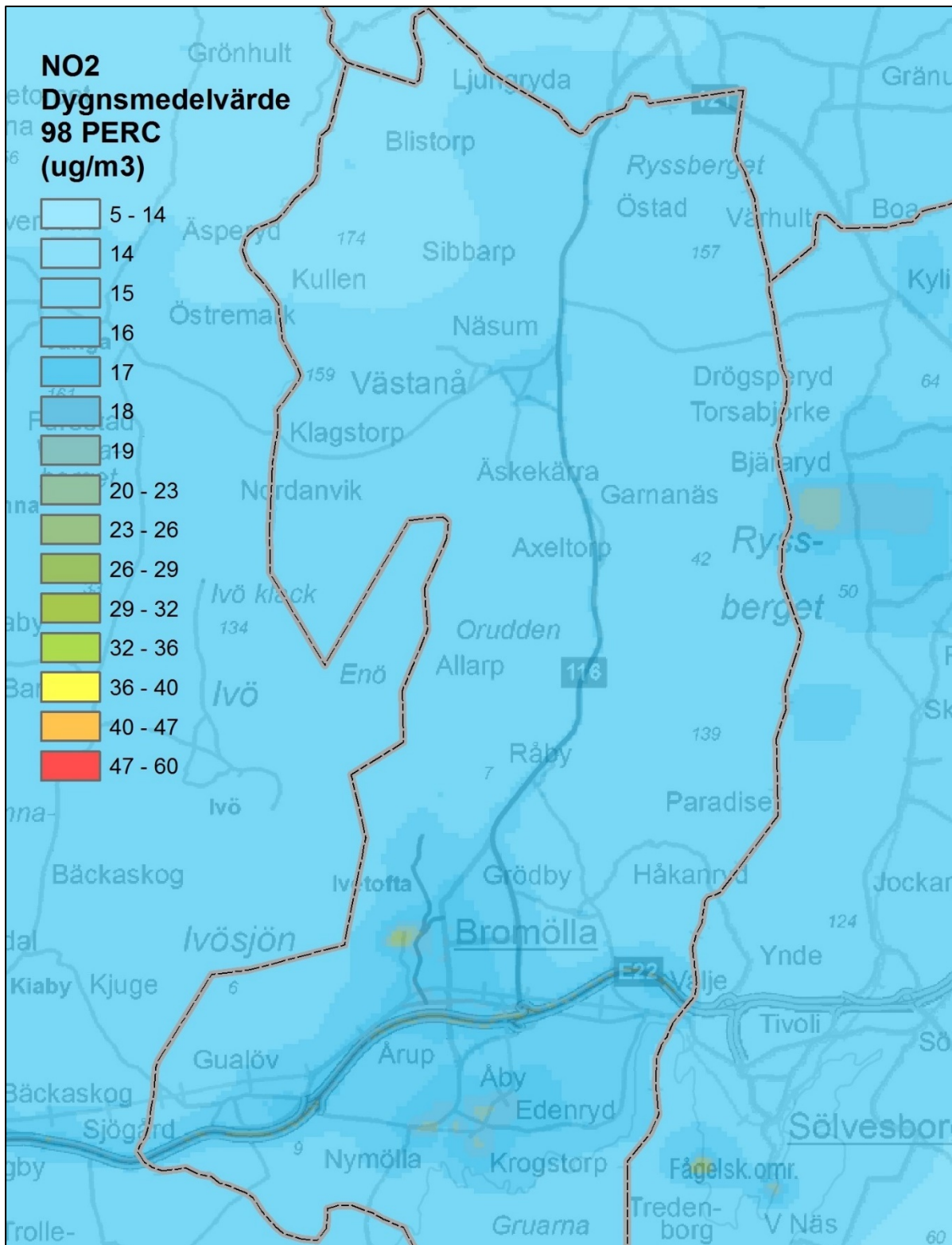
Figur 8. Beräknade dygnsmedelvärden av kvävedioxid inom kommunen ( \mu\text{g}/\text{m}^3 ).
