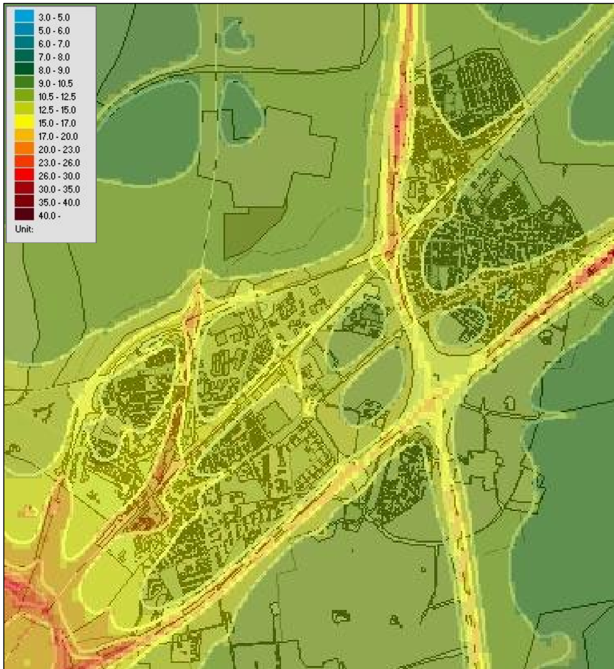
Figur 6. Beräknade årsmedelvärden av kvävedioxid i tätorten ( \mu\text{g}/\text{m}^3 ).
