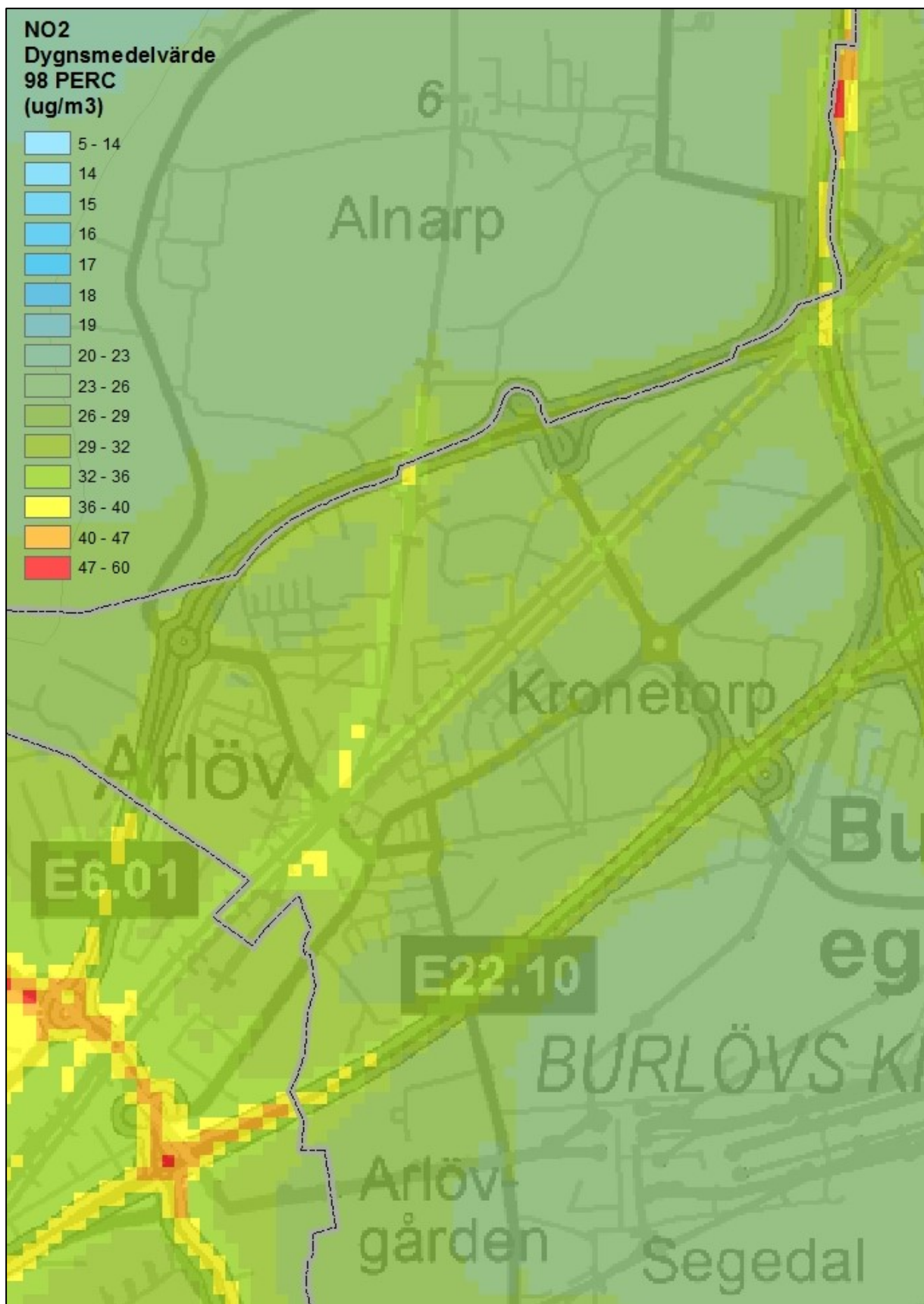
Figur 9. Beräknade dygnsmedelvärden av kvävedioxid i tätorten ( \mu\text{g}/\text{m}^3 ).
