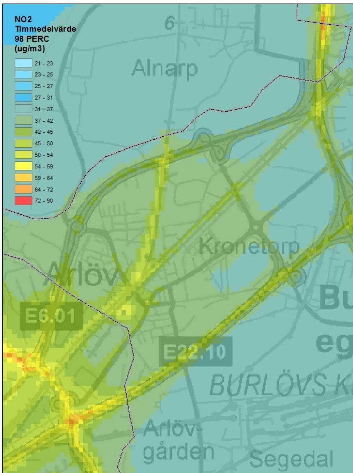
Figur 11. Beräknade timmedelvärden av kvävedioxid i tätorten ( \mu\text{g}/\text{m}^3 ).
