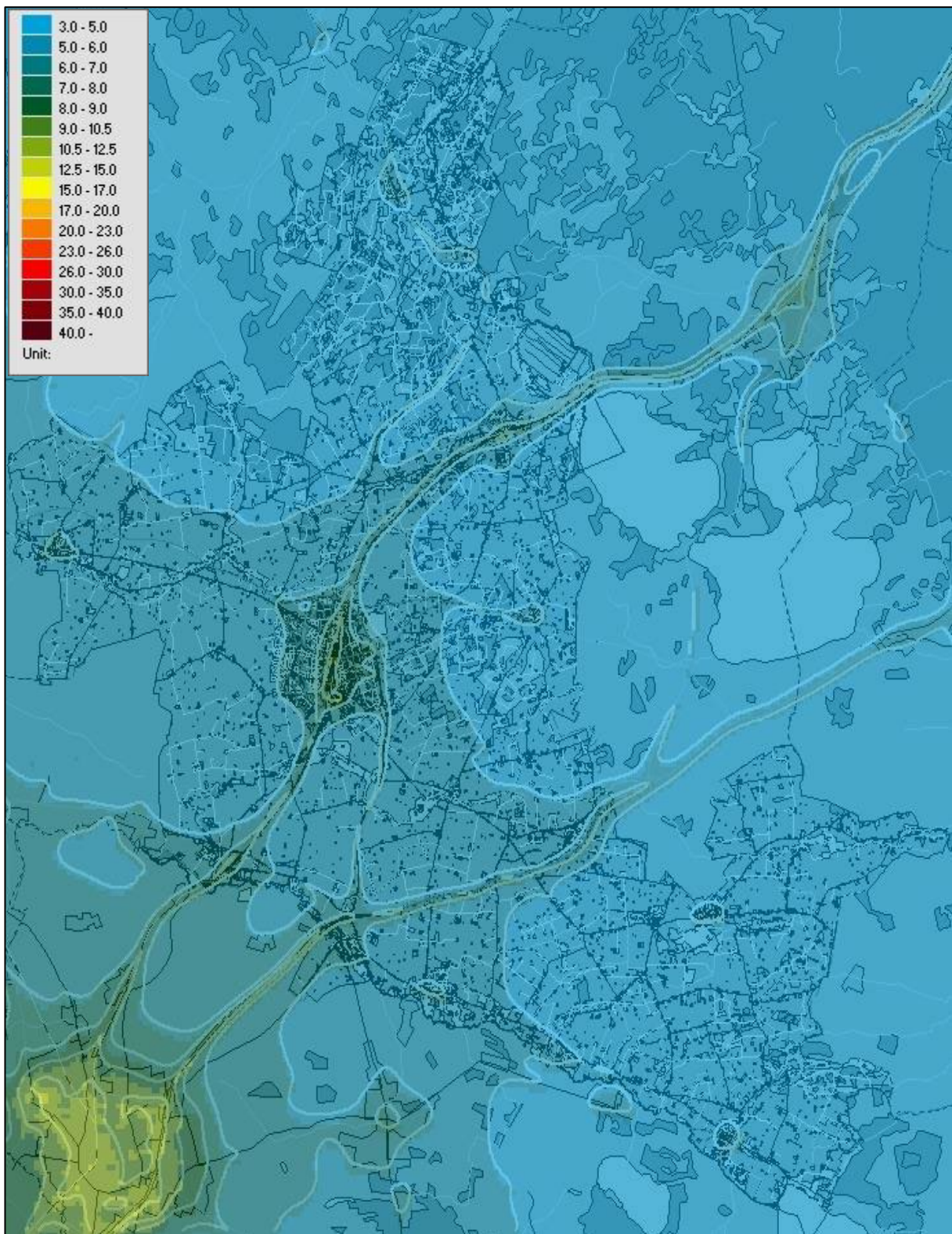
Figur 7. Beräknade årsmedelvärden av kvävedioxid inom kommunen ( \mu\text{g}/\text{m}^3 ).
