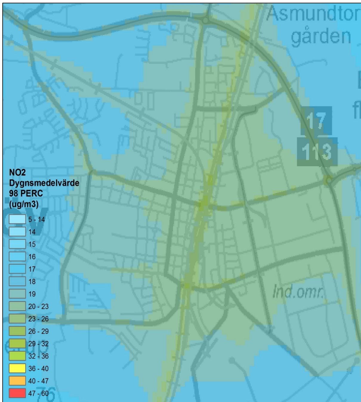
Figur 9. Beräknade dygnsmedelvärden av kvävedioxid i tätorten ( \mu\text{g}/\text{m}^3 ).
