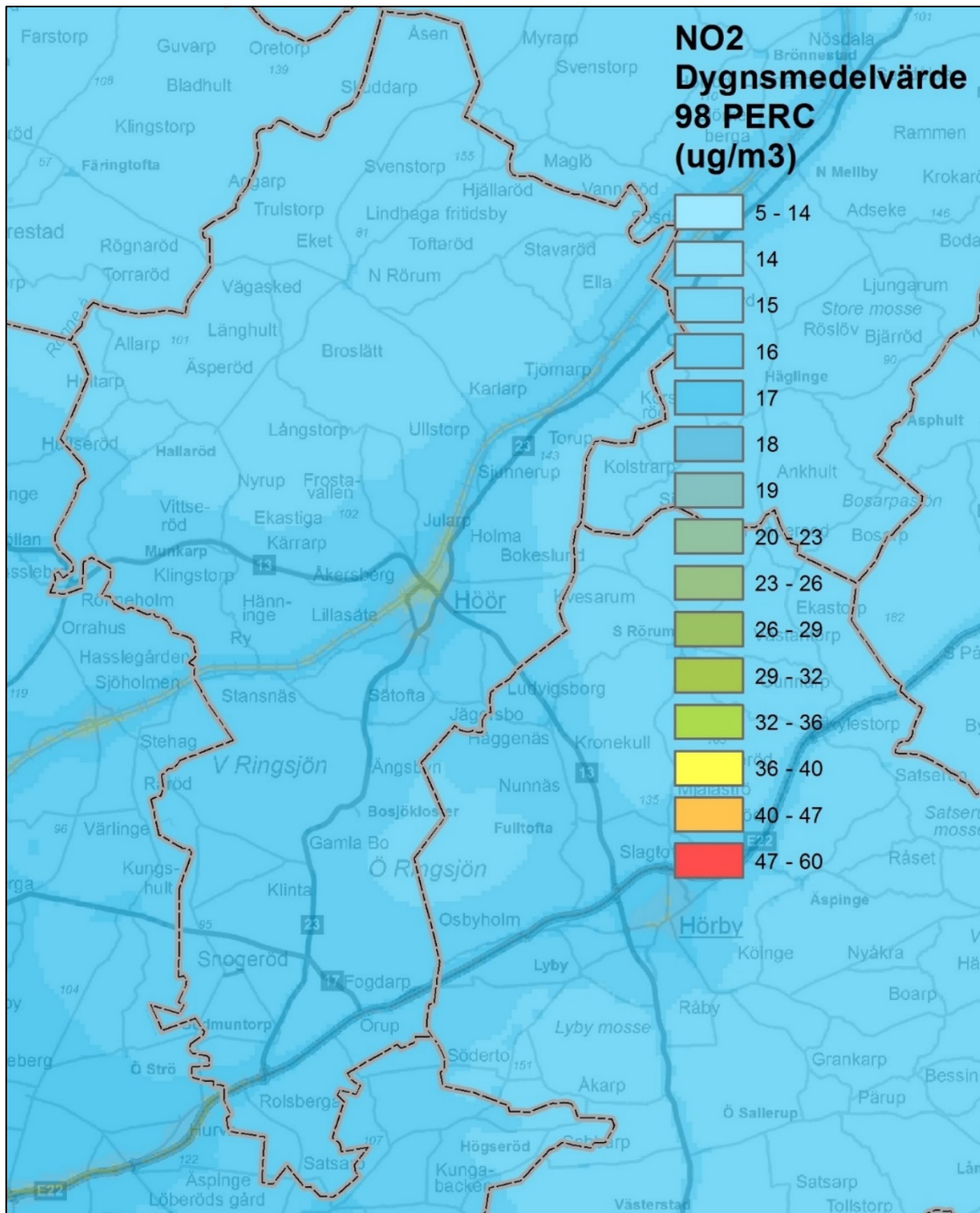
Figur 8. Beräknade dygnsmedelvärden av kvävedioxid inom kommunen ( \mu\text{g}/\text{m}^3 ).
