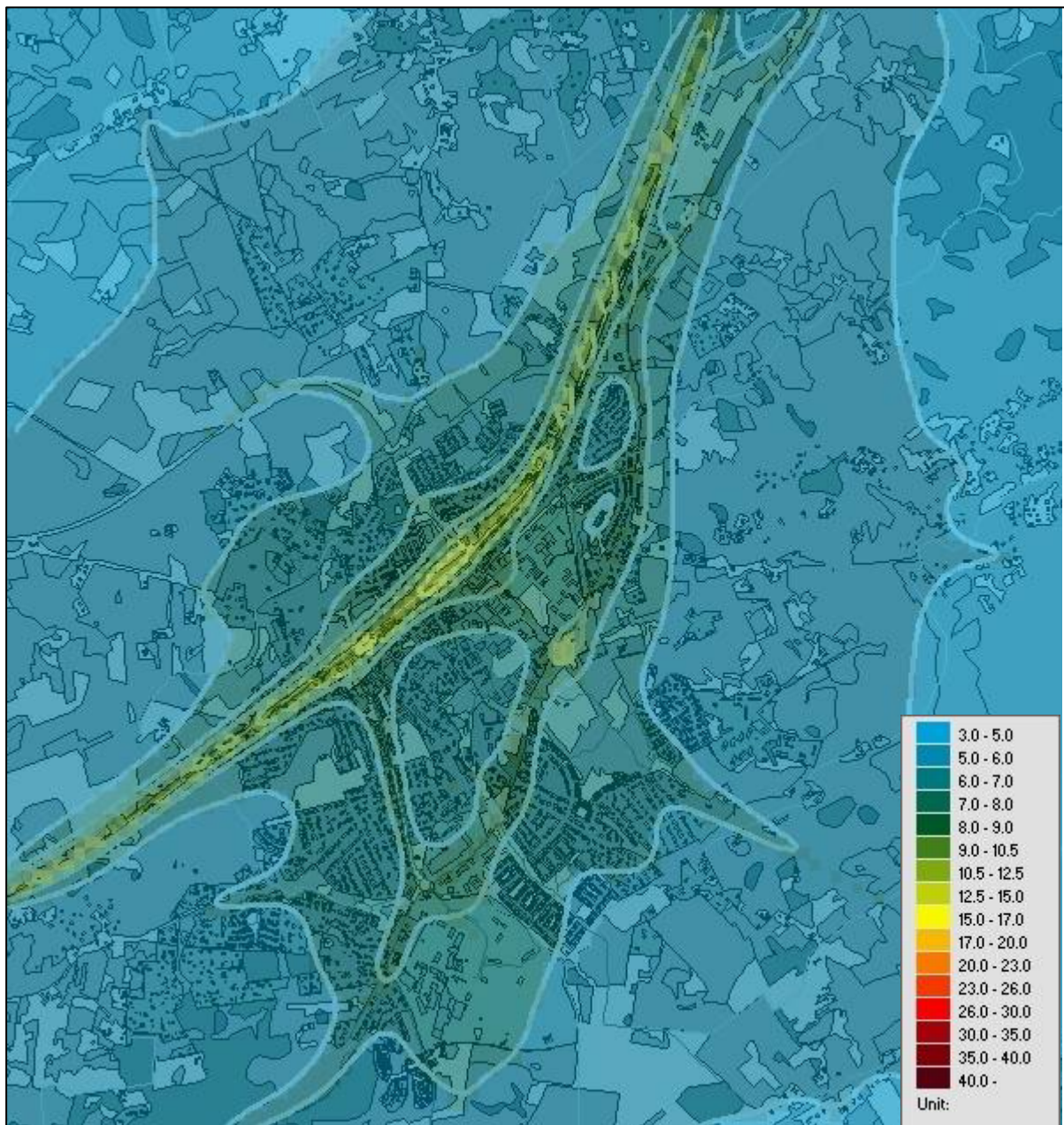
Figur 6. Beräknade årsmedelvärden av kvävedioxid i tätorten (µg/m 3 ).
