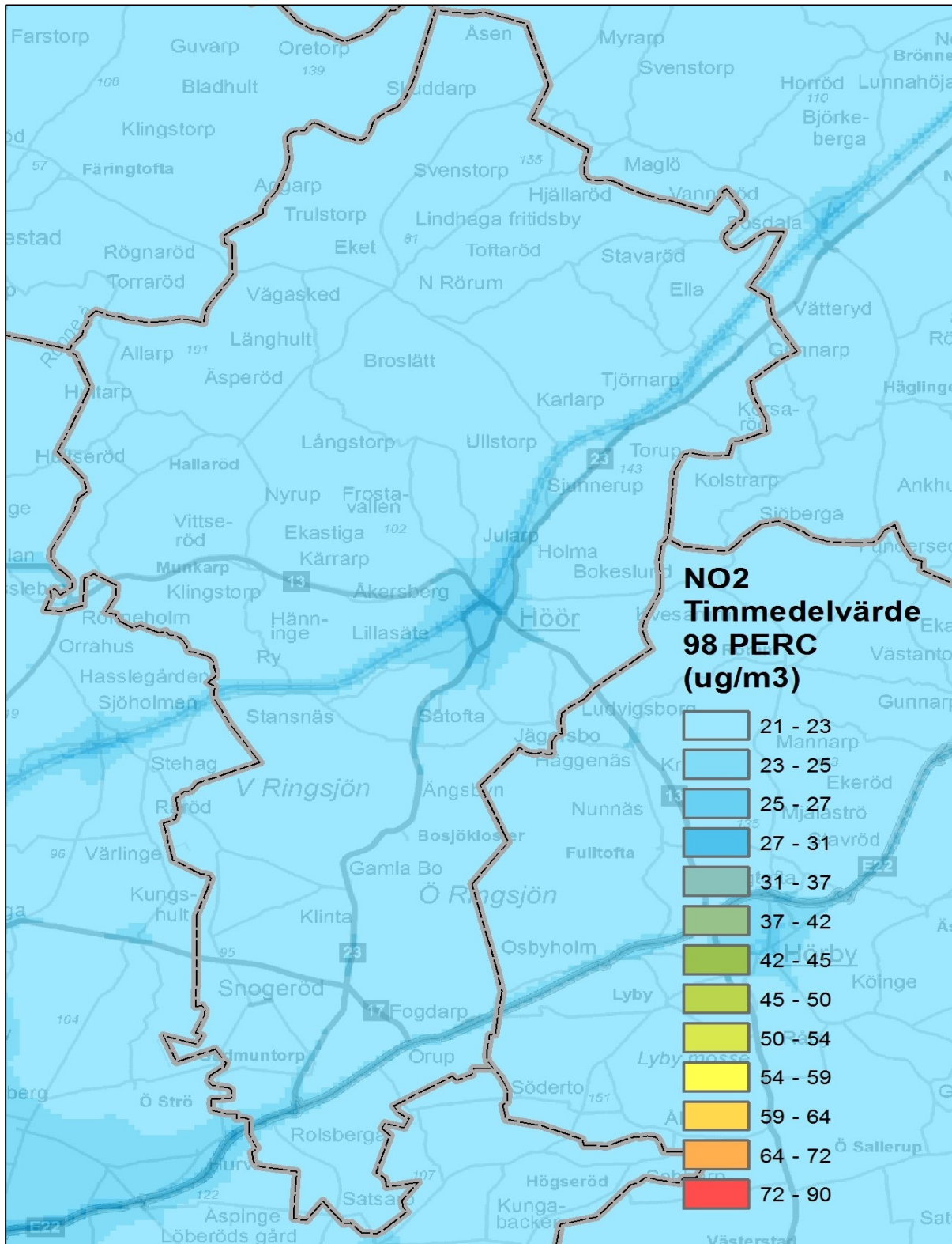
Figur 10. Beräknade timmedelvärden av kvävedioxid inom kommunen ( \mu\text{g}/\text{m}^3 ).
