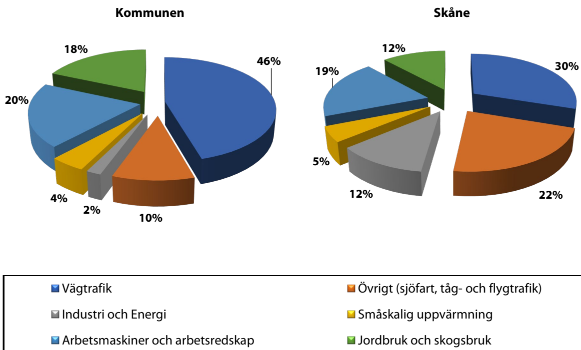
Figur 12. Procentuell fördelning av utsläppskällor för kväveoxider i kommunen jämfört med Skåne.
