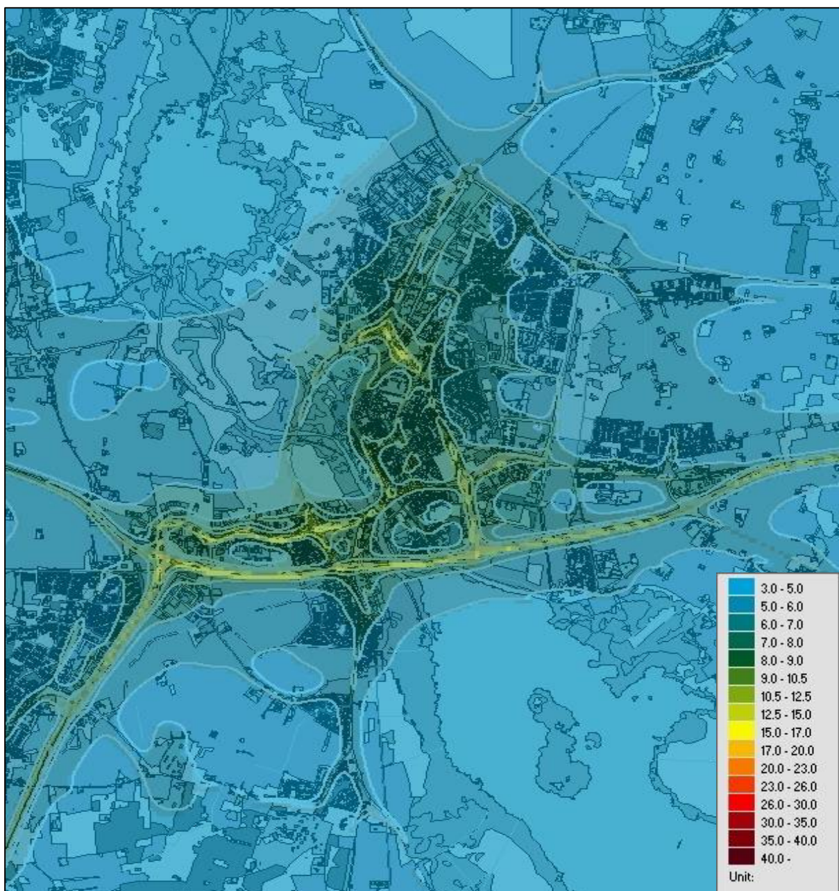
Figur 6. Beräknade årsmedelvärden av kvävedioxid i tätorten Kristianstad (µg/m 3 ).
