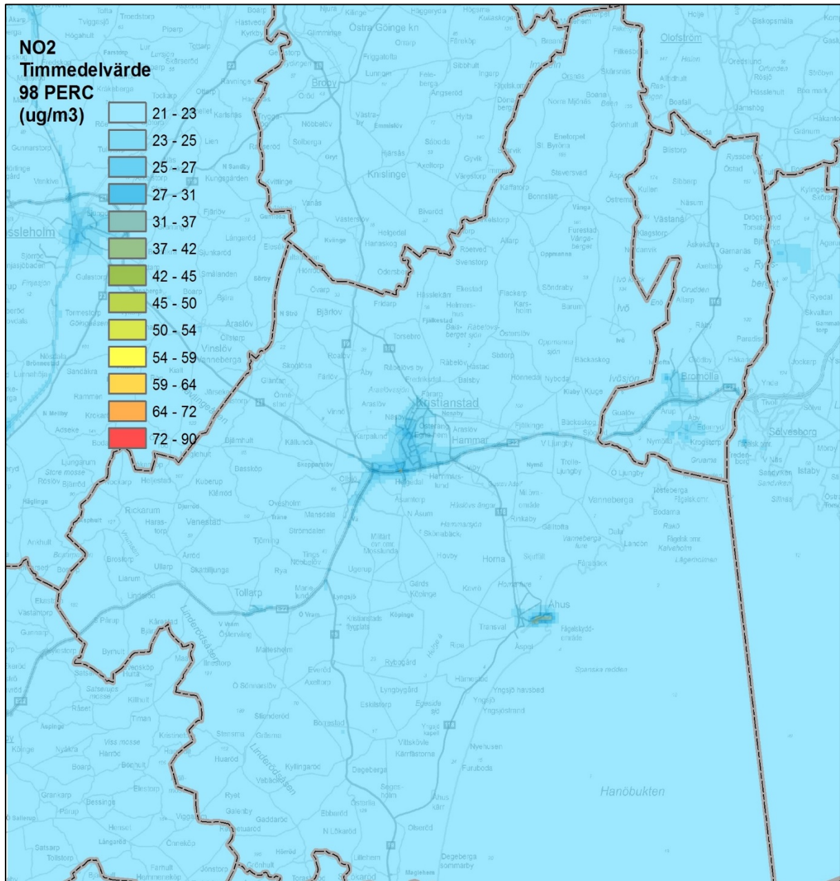
Figur 10. Beräknade timmedelvärderna av kvävedioxid inom kommunen ( \mu\text{g}/\text{m}^3 ).
