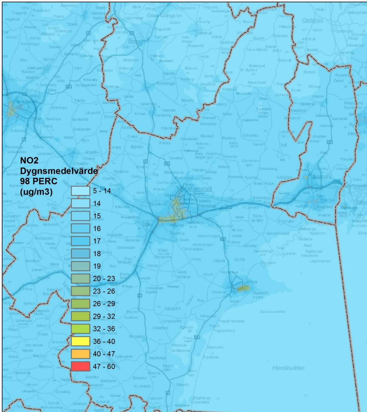
Figur 8. Beräknade dygnsnedelvärderna av kvävedioxid inom kommunen ( \mu\text{g}/\text{m}^3 ).
