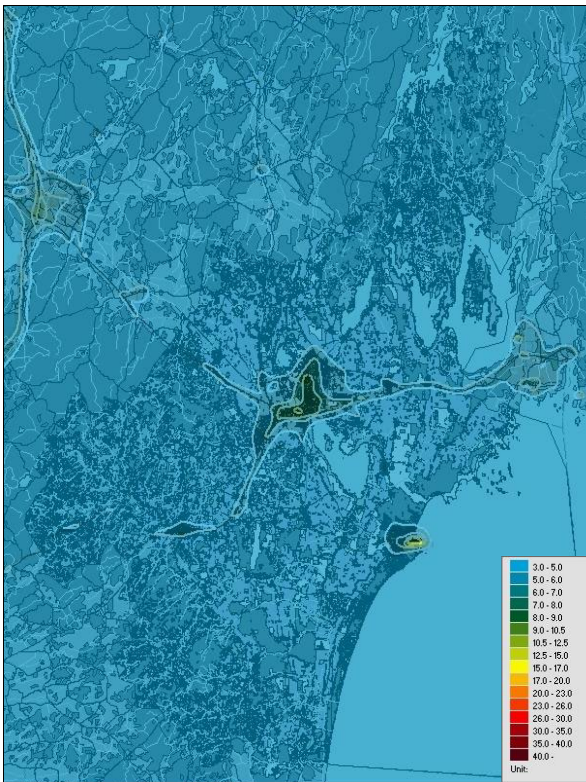
Figur 7. Beräknade årsmedelvärden av kvävedioxid inom kommunen ( \mu\text{g}/\text{m}^3 ).
