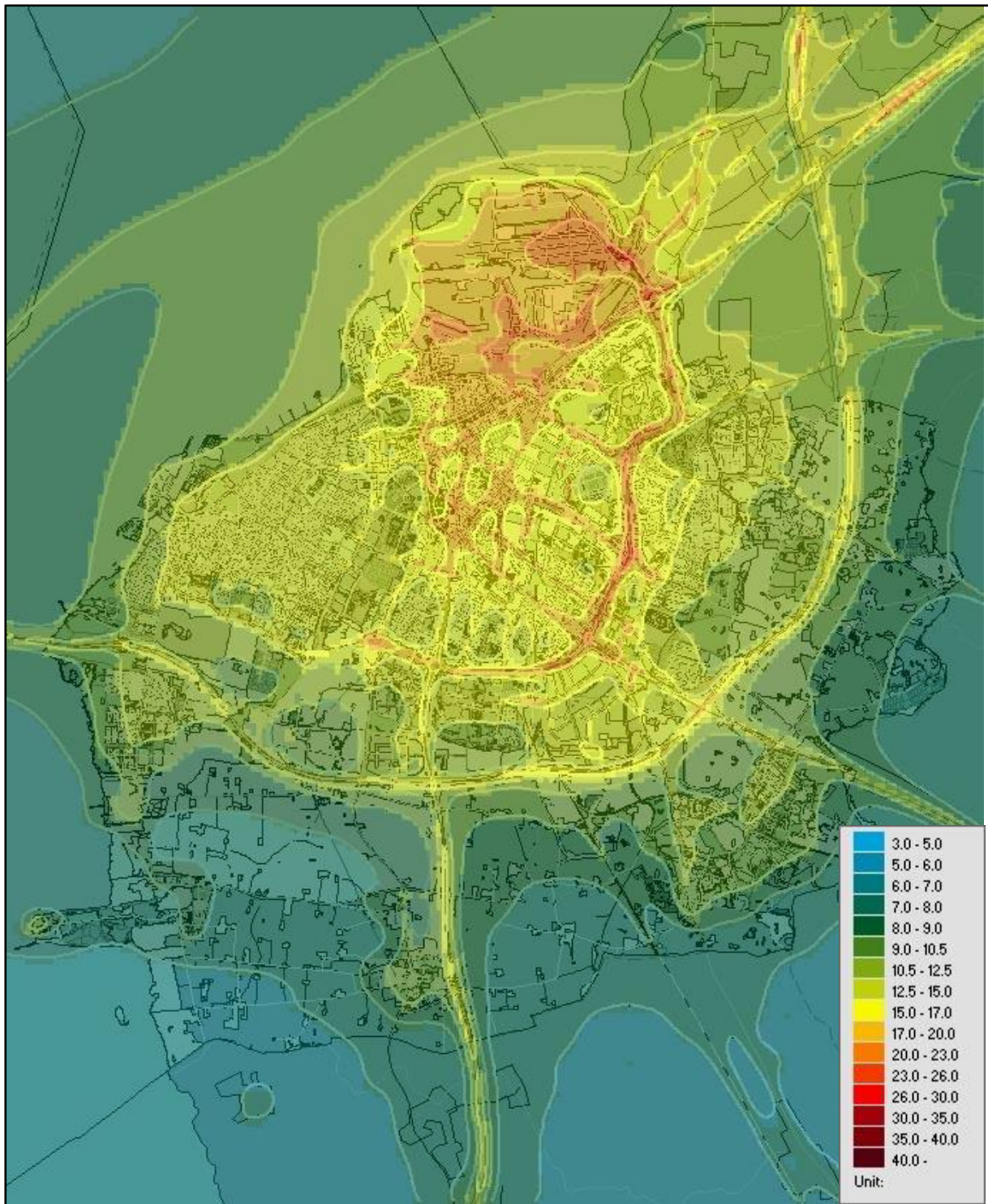
Figur 7. Beräknade årsmedelvärden av kvävedioxid inom kommunen (µg/m 3 ).
