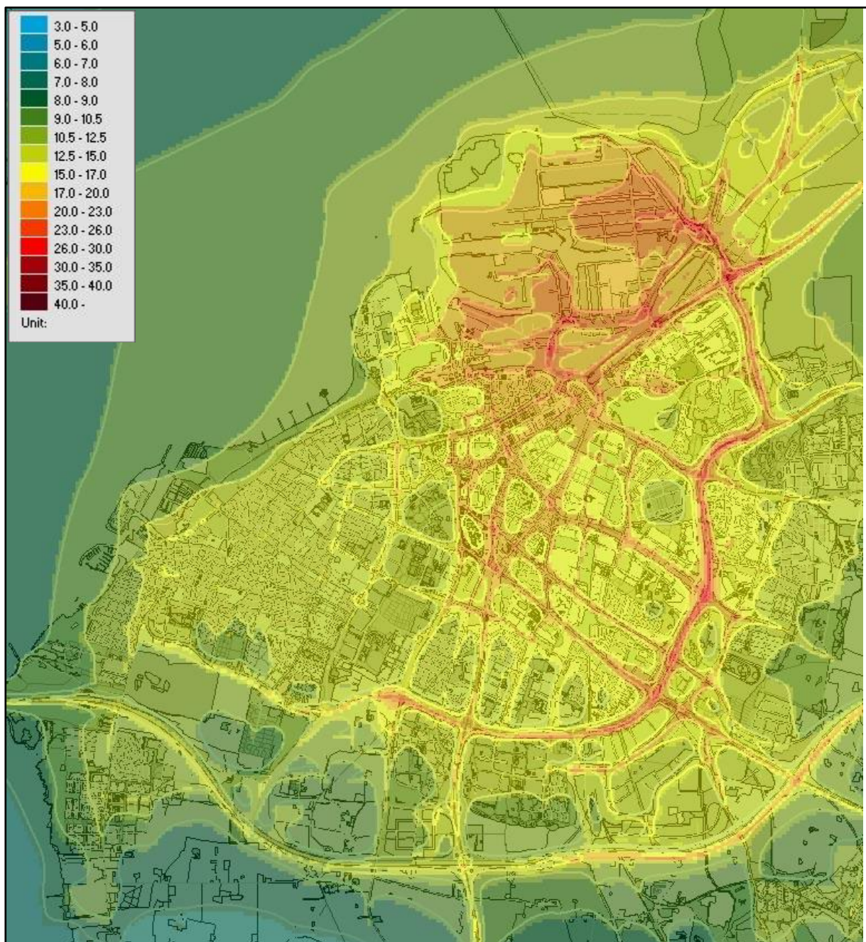
Figur 6. Beräknade årsmedelvärden av kvävedioxid i tätorten Malmö (µg/m 3 ).
