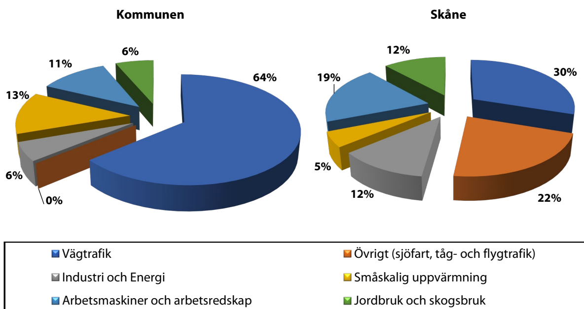
Figur 12. Procentuell fördelning av utsläppskällor för kväveoxider i kommunen jämfört med Skåne.
