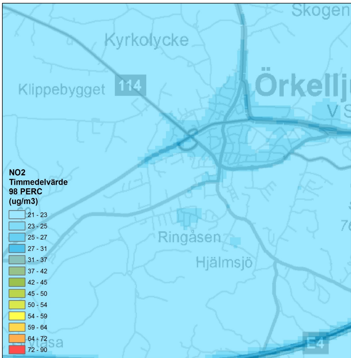
Figur 11. Beräknade timmedelvärden av kvävedioxid i tätorten (µg/m³).
