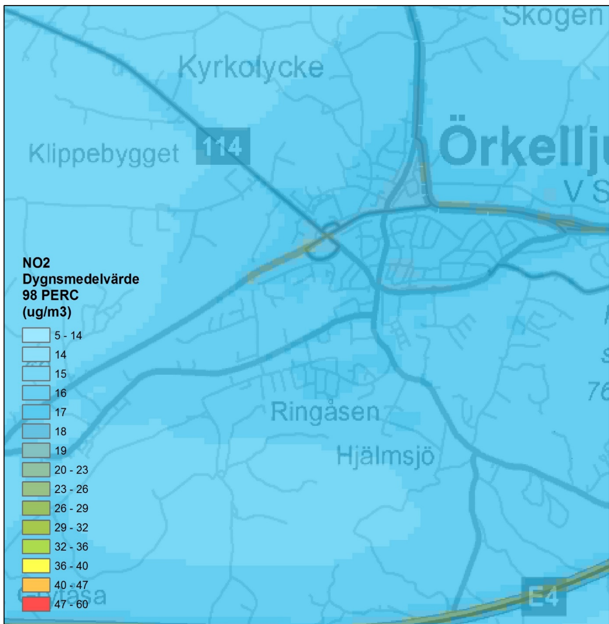
Figur 9. Beräknade dygnsnivåer av kvävedioxid i tätorten ( \mu\text{g}/\text{m}^3 ).
