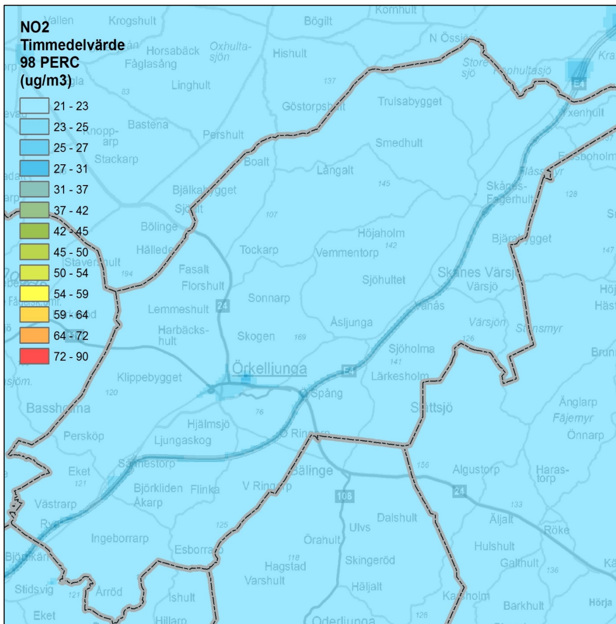
Figur 10. Beräknade timmedelvärden av kvävedioxid inom kommunen ( \mu\text{g}/\text{m}^3 ).
