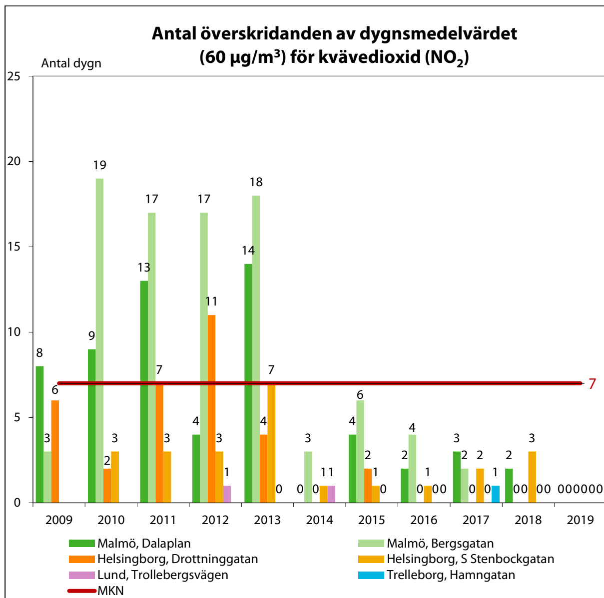
Figur 3. Antal överskridanden av dygnsmedelvärdet för kvävedioxid (NO 2 ) under tio år inom samverkansområdet Skåne.
