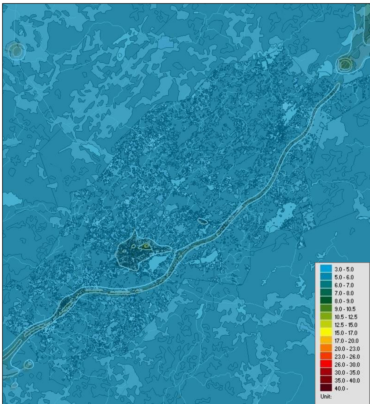
Figur 6. Beräknade årsmedelvärden av kvävedioxid inom kommunen (µg/m 3 ).
