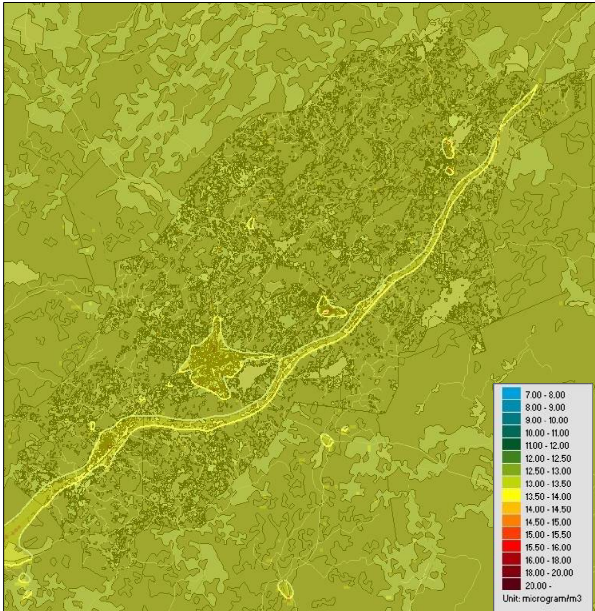
Figur 17. Beräknade årsmedelvärden av partiklar PM 10 inom kommunen (µg/m 3 ).
