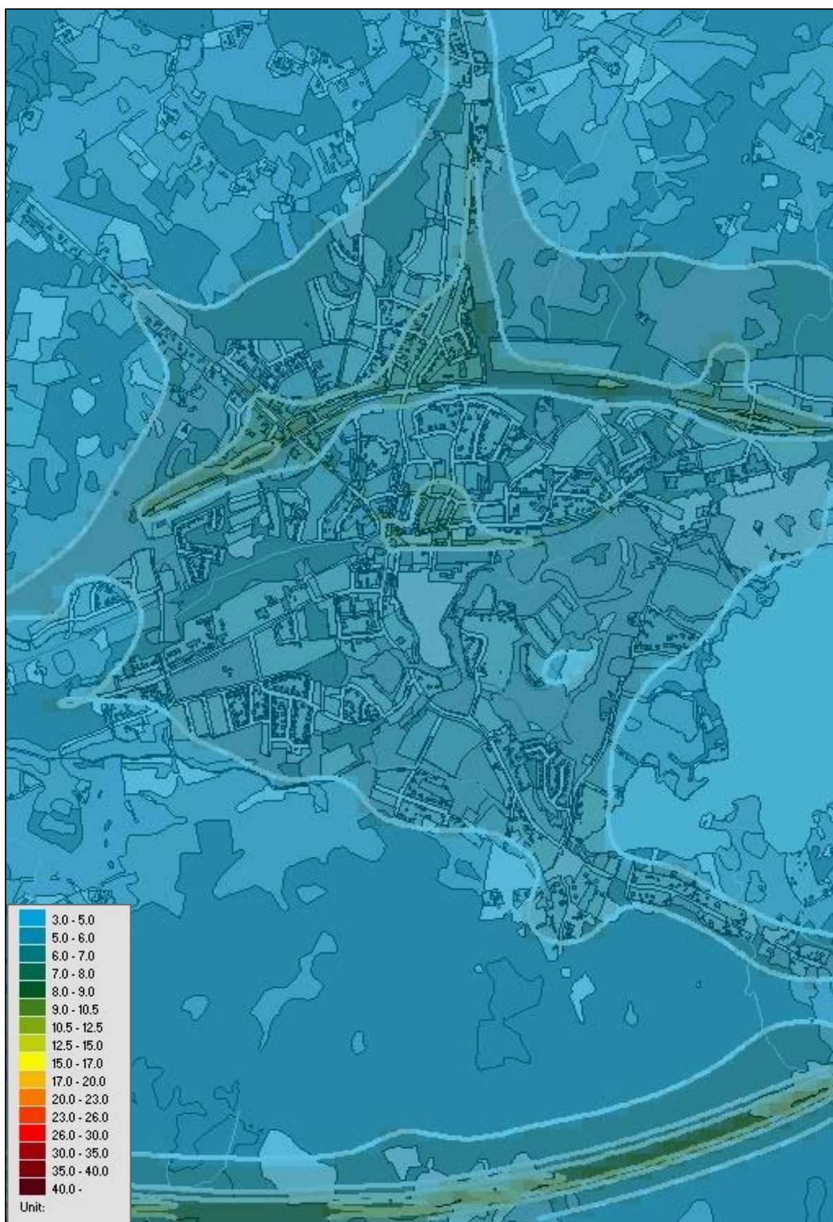
Figur 7. Beräknade årsmedelvärden av kvävedioxid i tätorten ( \mu\text{g}/\text{m}^3 ).
