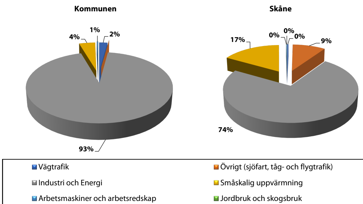
Figur 27. Procentuell fördelning av utsläppskällor för svaveldioxid (SO 2 ) i kommunen jämfört med Skåne.
