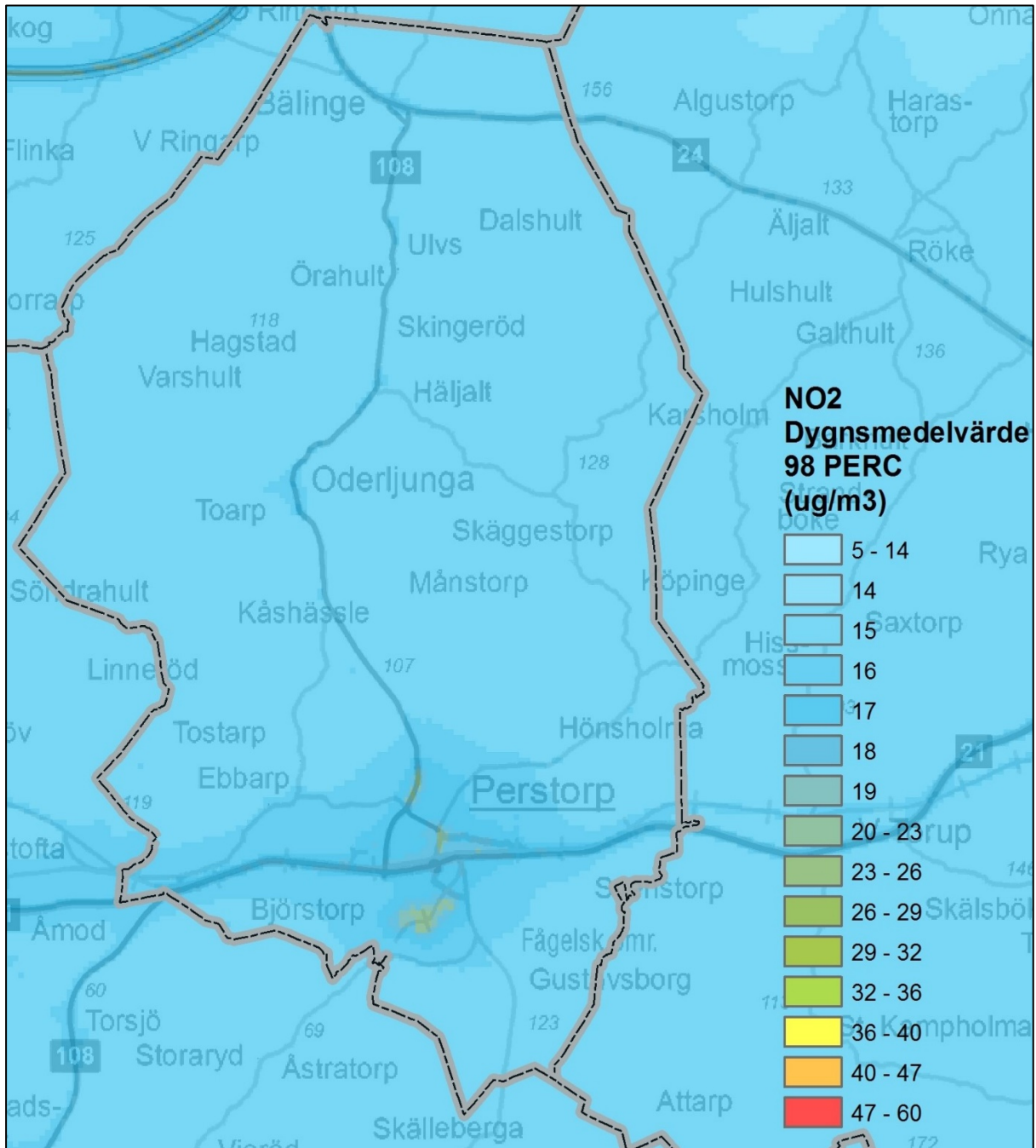
Figur 8. Beräknade dygnsmedelvärden av kvävedioxid inom kommunen ( \mu\text{g}/\text{m}^3 ).
