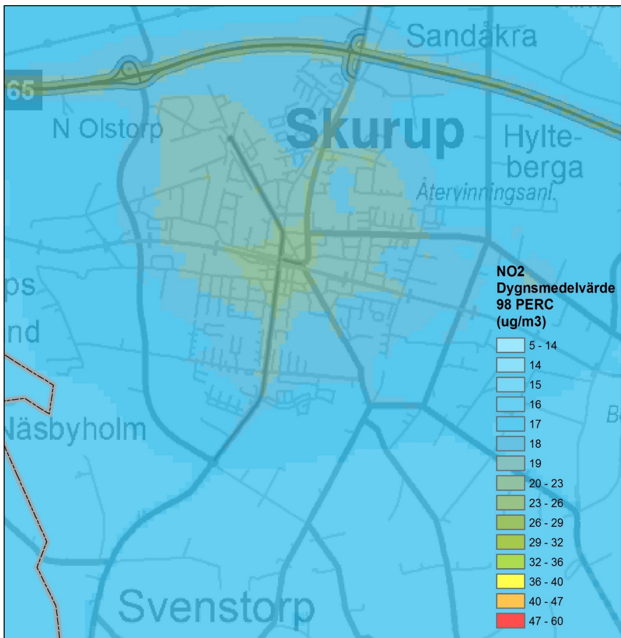
Figur 9. Beräknade dygnsmedelvärden av kvävedioxid i tätorten ( \mu\text{g}/\text{m}^3 ).
