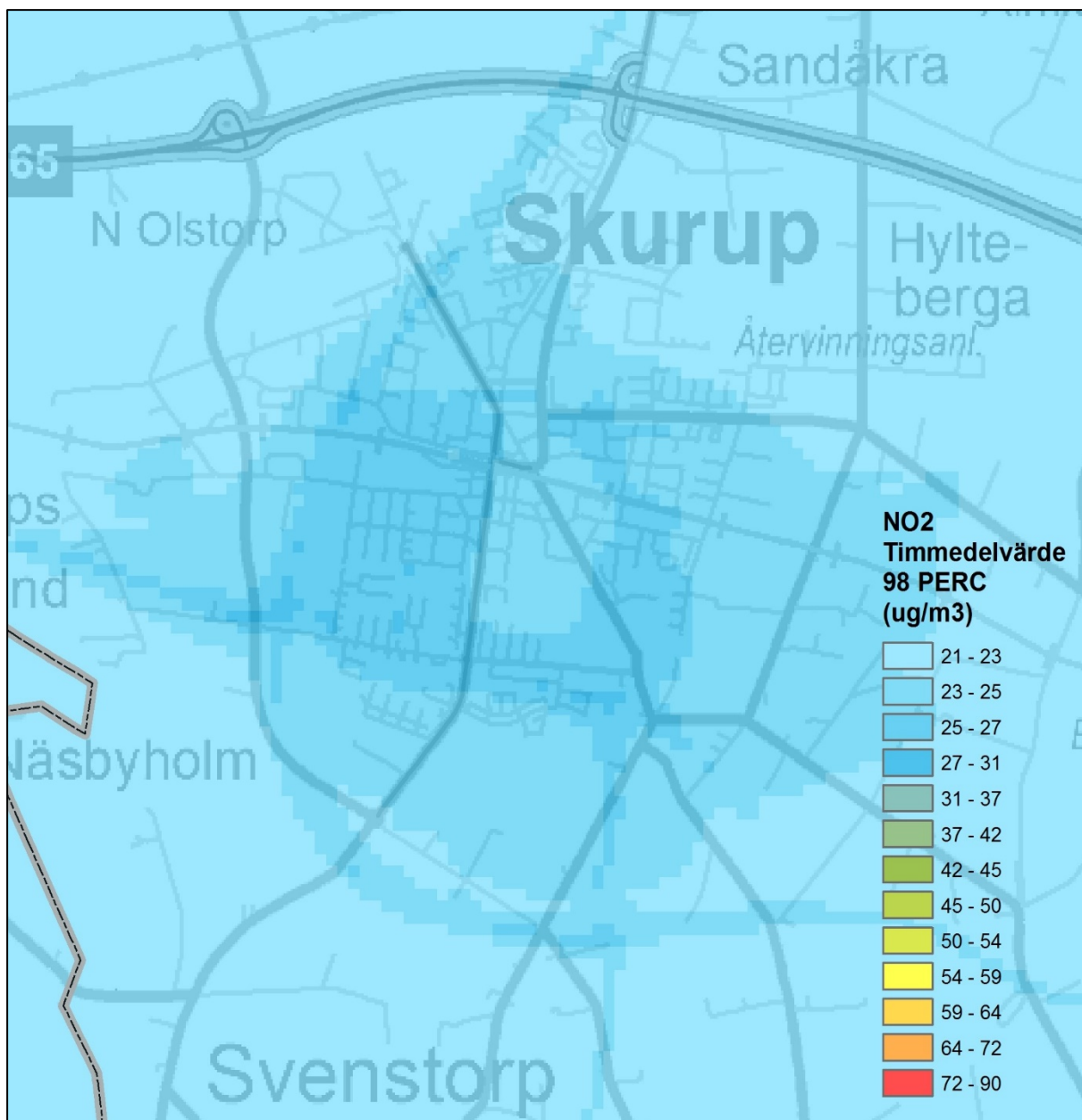
Figur 11. Beräknade timmedelvärden av kvävedioxid i tätorten (µg/m 3 ).
