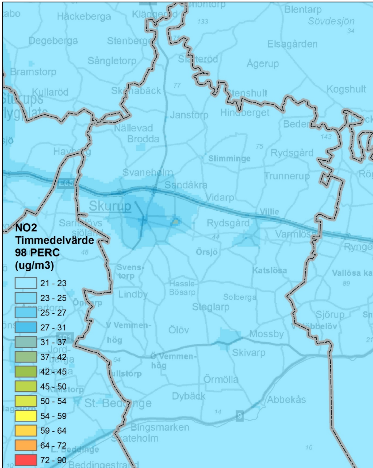
Figur 10. Beräknade timmedelvärden av kvävedioxid inom kommunen ( \mu\text{g}/\text{m}^3 ).
