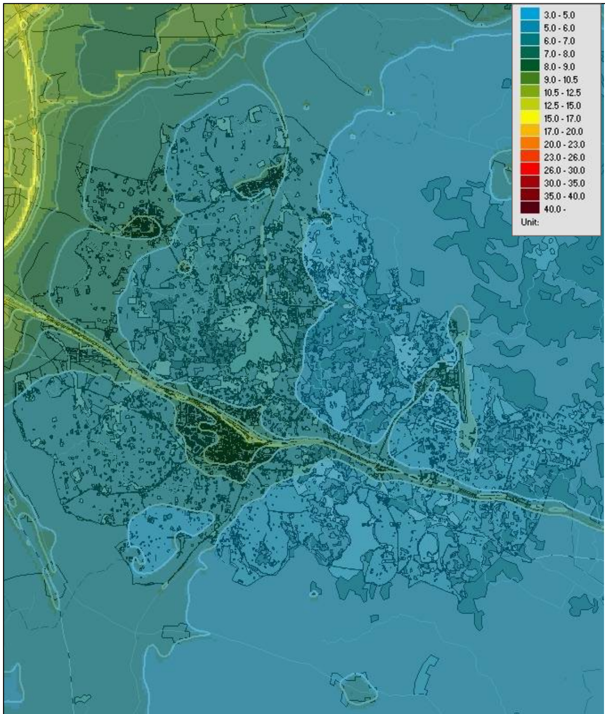
Figur 7. Beräknade årsmedelvärden av kvävedioxid inom kommunen ( \mu\text{g}/\text{m}^3 ).
