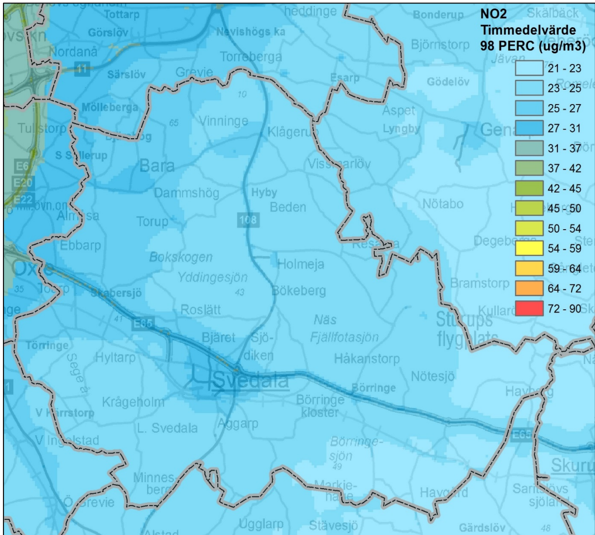
Figur 10. Beräknade timmedelvärden av kvävedioxid inom kommunen ( \mu\text{g}/\text{m}^3 ).
