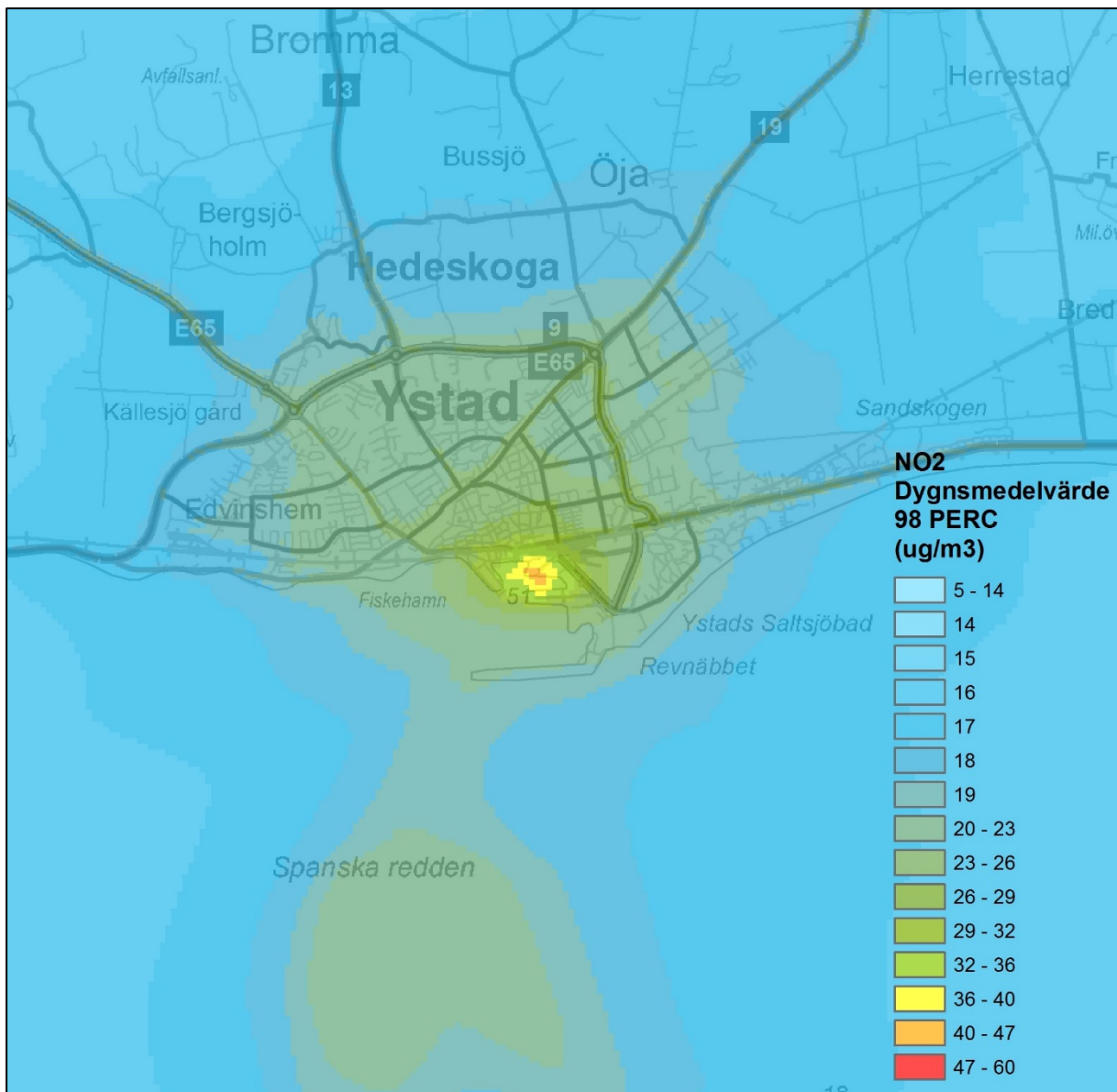
Figur 9. Beräknade dygnsmedelvärden av kvävedioxid i tätorten ( \mu\text{g}/\text{m}^3 ).
