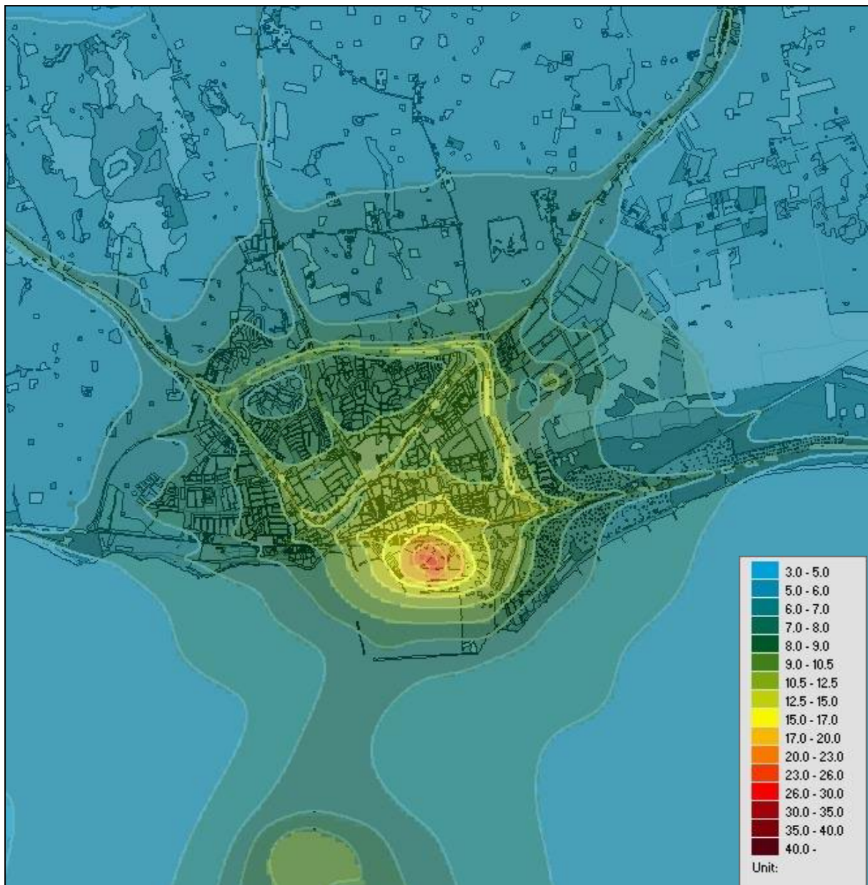
Figur 6. Beräknade årsmedelvärden av kvävedioxid i tätorten (µg/m 3 ).
