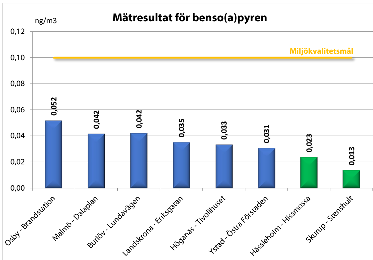
Figur 30. Medelvärdet för bens(a)pyren under mätperioden inom samverkansområdet Skåne.
