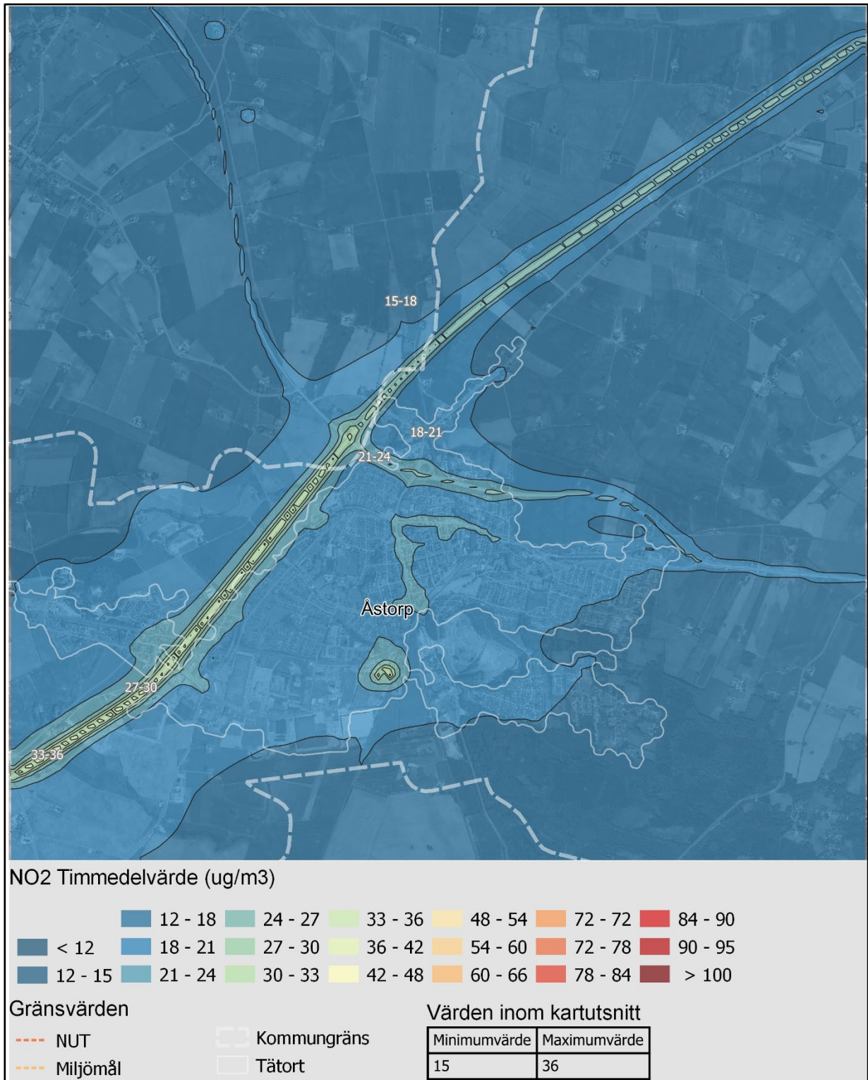
Figur 9. Beräknade timmedelvärden av kvävedioxid i tätorten ( \mu\text{g}/\text{m}^3 ).
