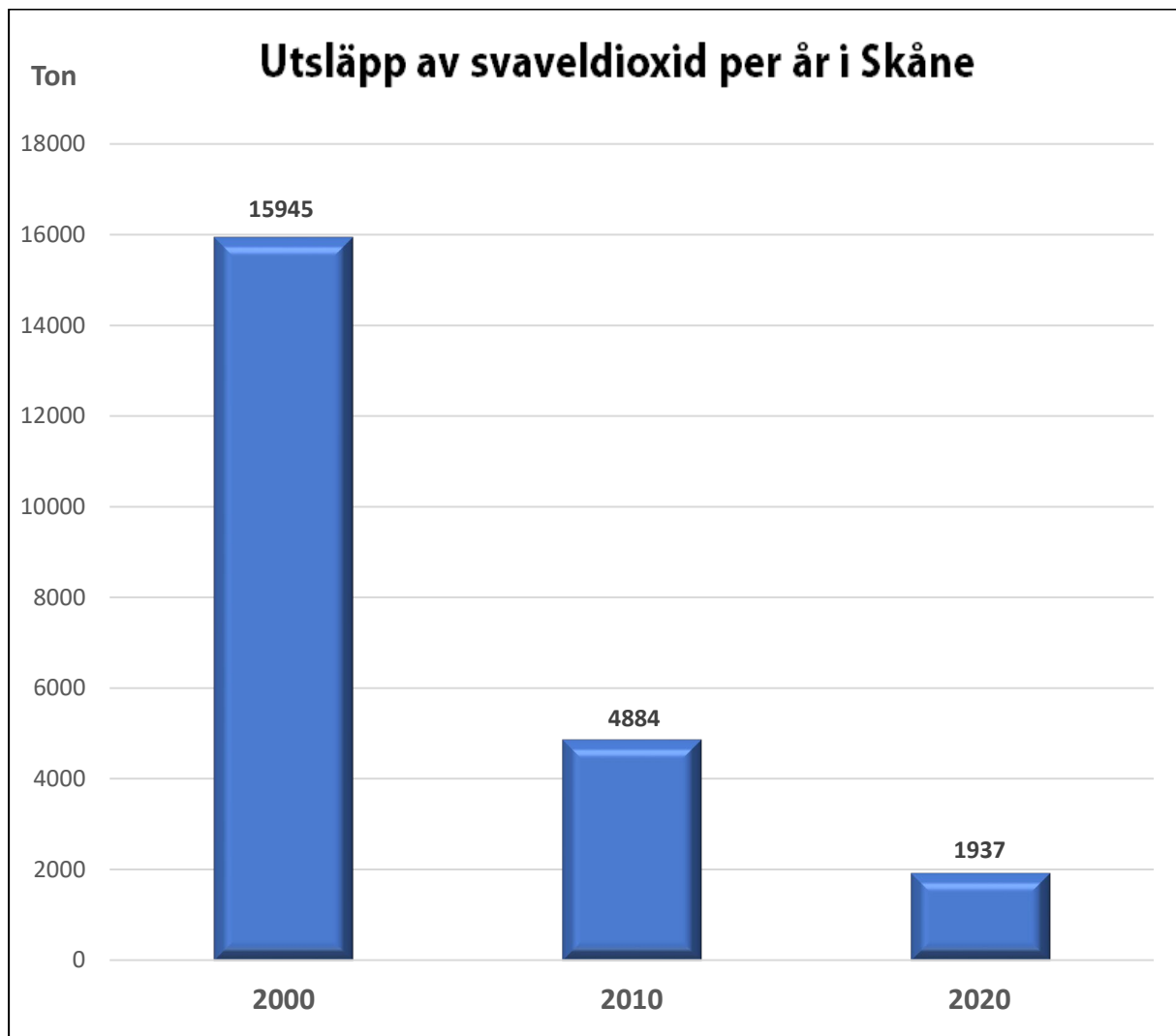
Figur 24. Beräknade utsläpp per år för svaveldioxid (SO 2 ) under de senaste två decennierna i Skåne.
