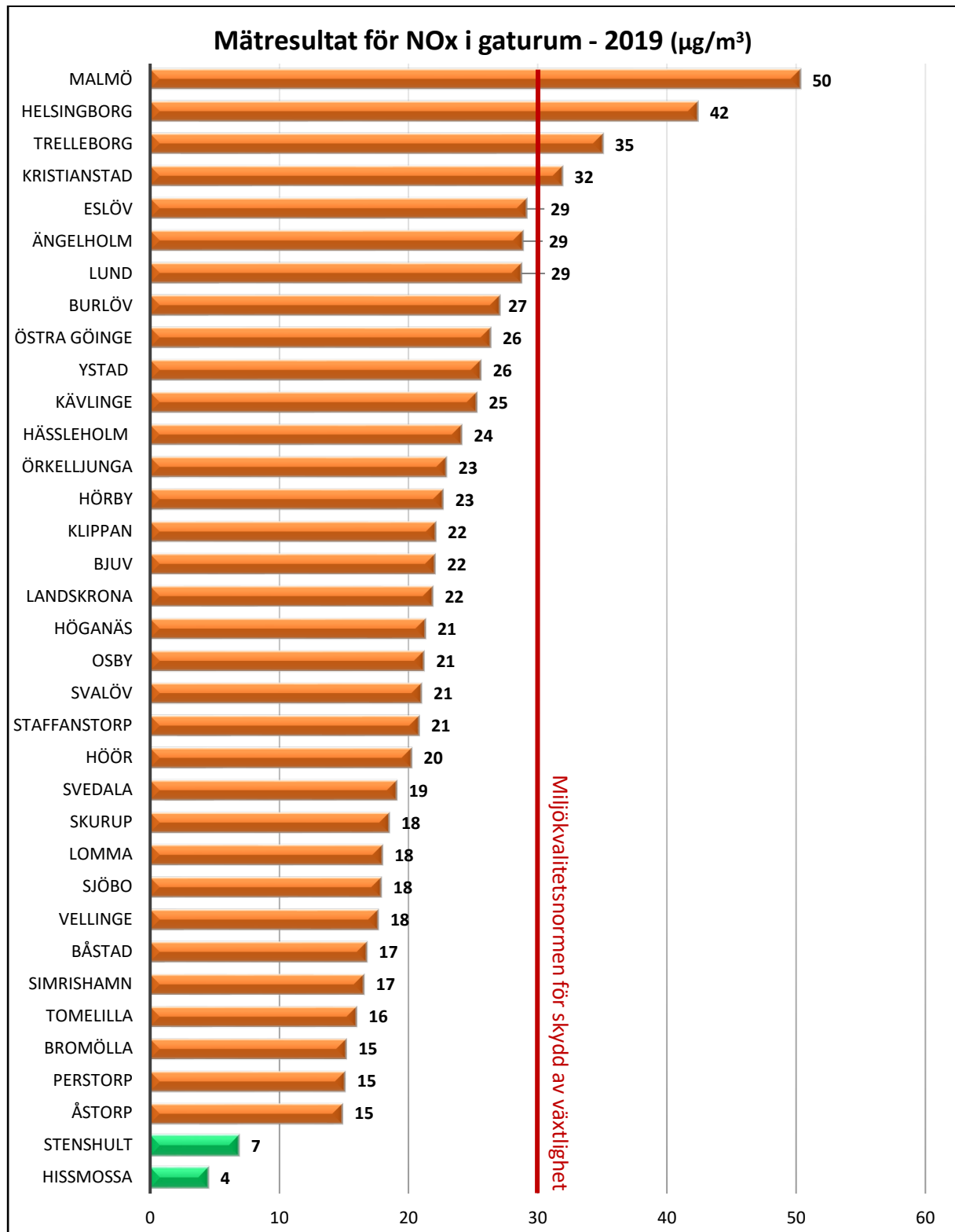
Figur 12. Uppmätta halter av kväveoxider (NO x ) under 2019 inom samverkansområdet Skåne.
