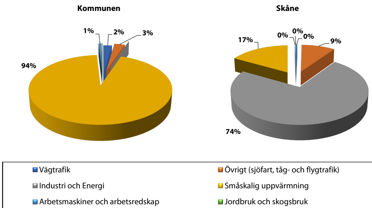
Figur 26. Procentuell fördelning av utsläppskällor för svaveldioxid (SO 2 ) i kommunen jämfört med Skåne.
