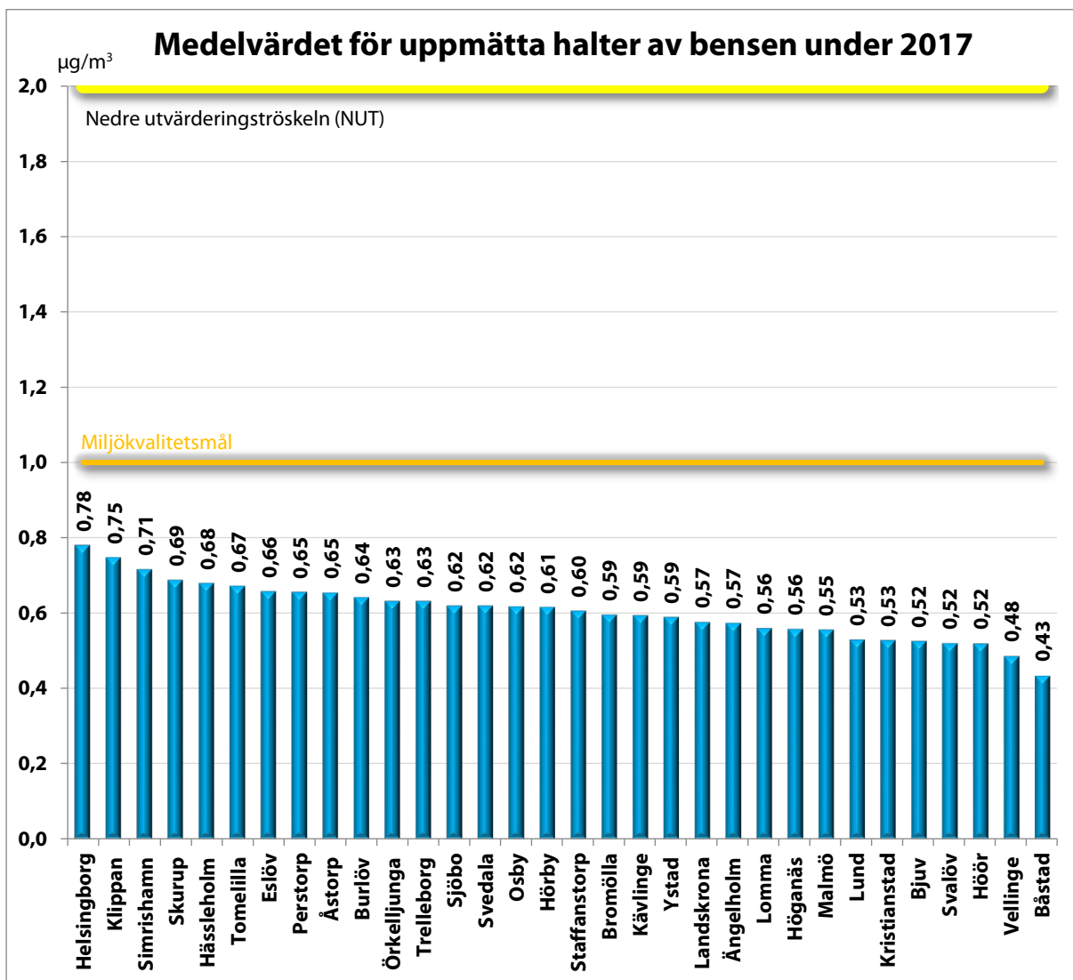
Figur 28. Uppmätta halter av bensen under 2017 i förhållande till Miljömålet och NUT.
