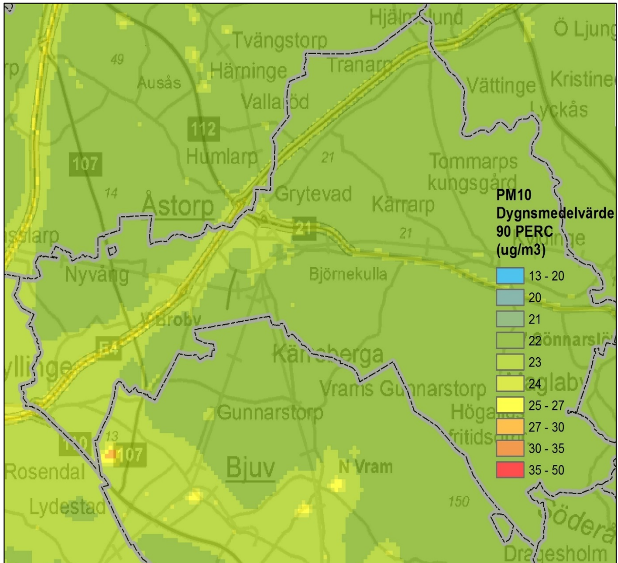
Figur 17. Beräknade dygnsmedelvärden av partiklar PM 10 inom kommunen (µg/m 3 ).
