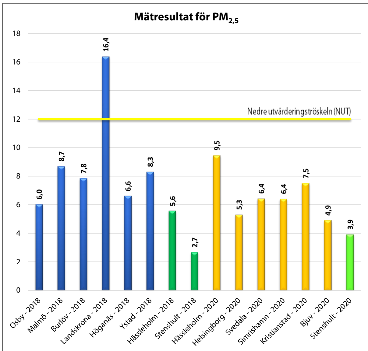
Figur 20. Uppmätta halter för partiklar (PM 2,5 ) under två mätperioder (2018 och 2020) inom samverkansområdet Skåne.
