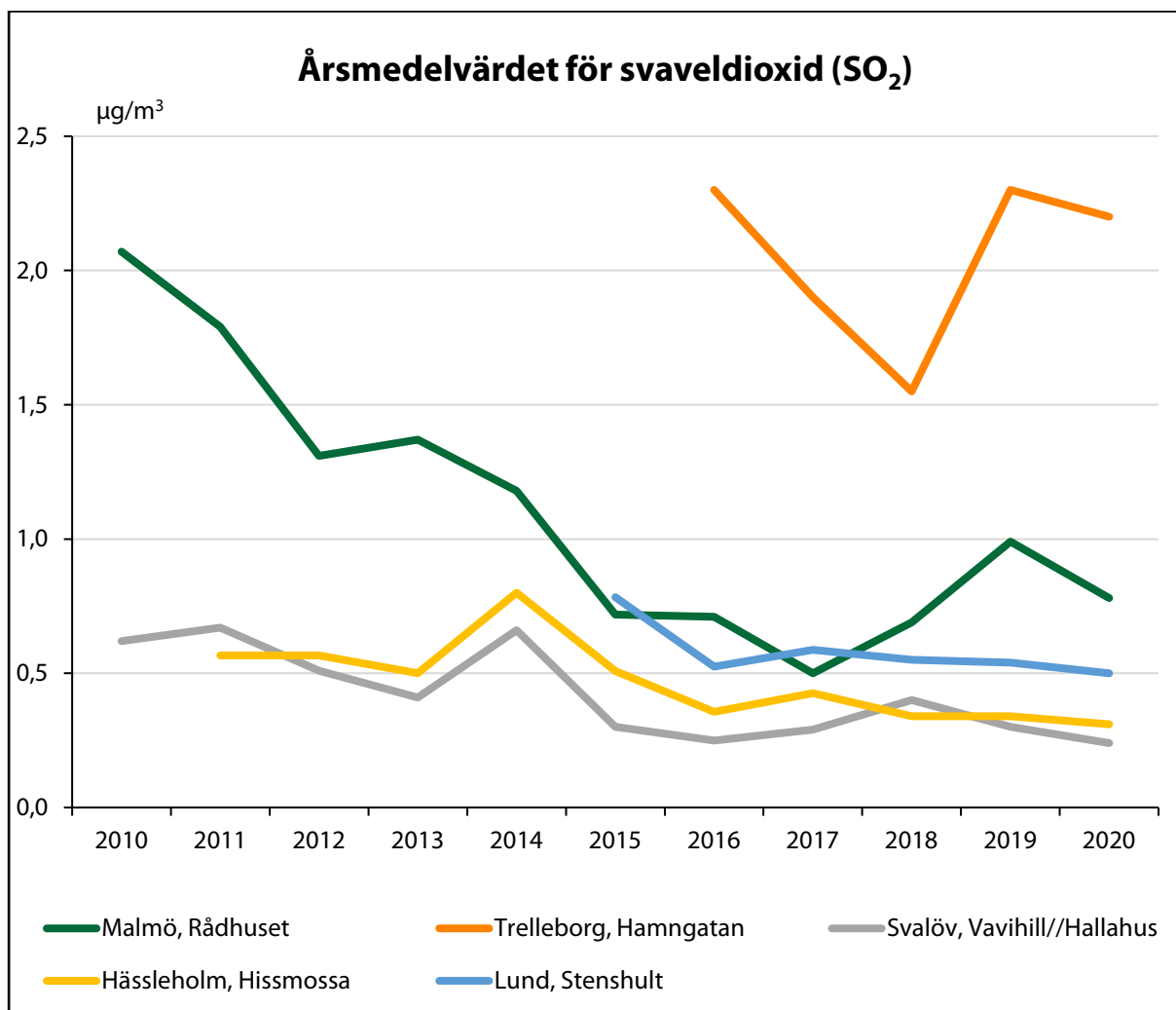
Figur 23. Årsmedelvärdet för svaveldioxid (SO 2 ) under tio år inom samverkansområdet Skåne.
