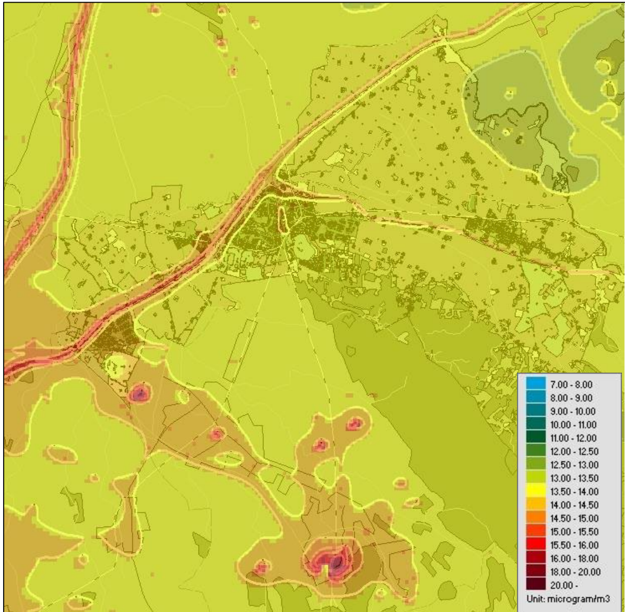
Figur 16. Beräknade årsmedelvärden av partiklar PM 10 inom kommunen (µg/m 3 ).
