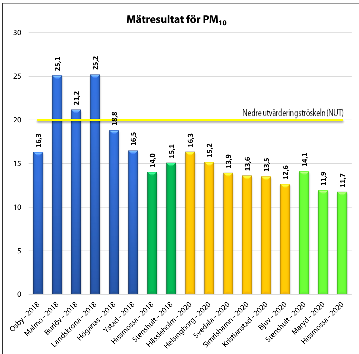
Figur 15. Uppmätta halter för partiklar (PM 10 ) under två mätperioder (2018 och 2020) inom samverkansområdet Skåne.
