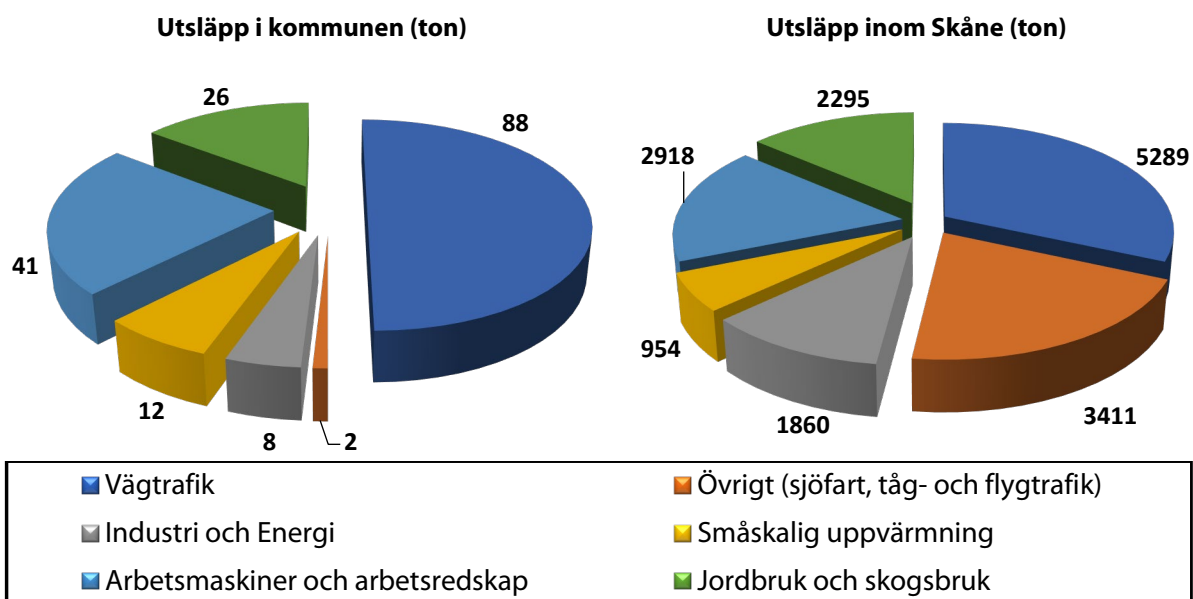
Figur 11. Fördelning av utsläppskällor för NO x i kommunen jämfört med hela samverkansområdet Skåne.
