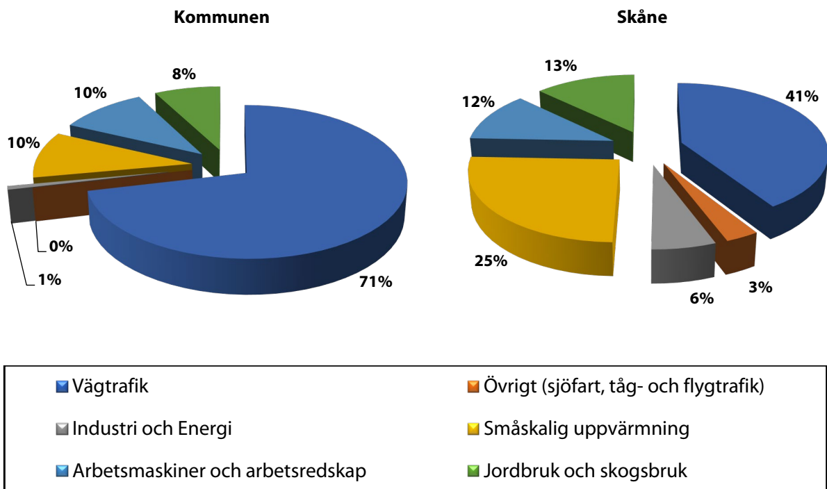
Figur 18. Procentuell fördelning av utsläppskällor för partiklar (PM 10 ) i kommunen jämfört med Skåne.
