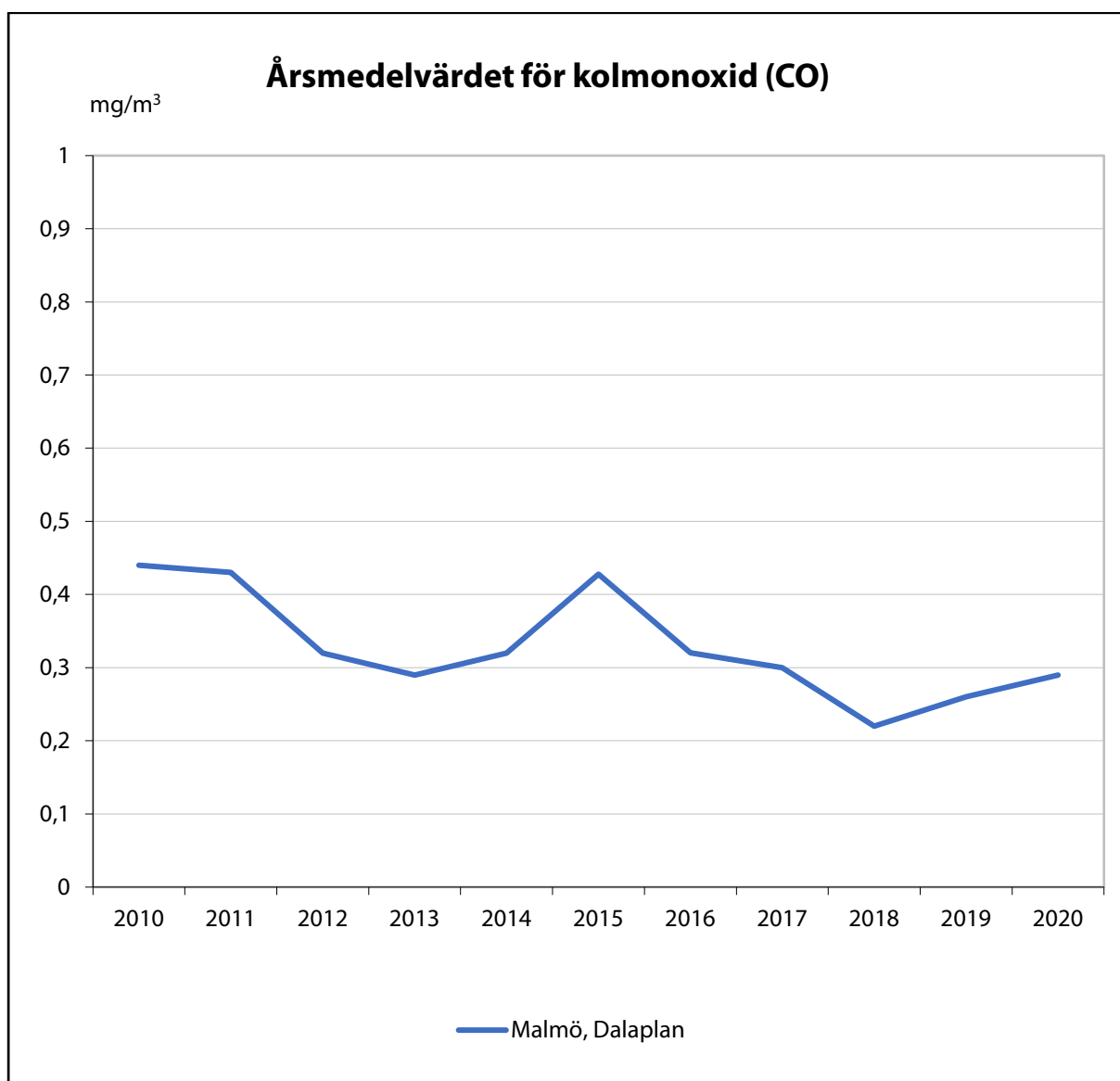
Figur 27. Årsmedelvärdet för kolmonoxid (CO) under tio år inom samverkansområdet Skåne.
