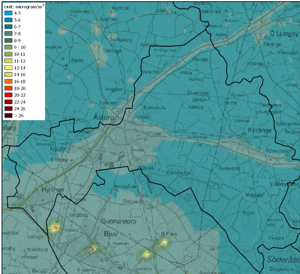
Figur 21. Beräknade årsmedelvärden av partiklar PM 2,5 inom kommunen (µg/m 3 ).
