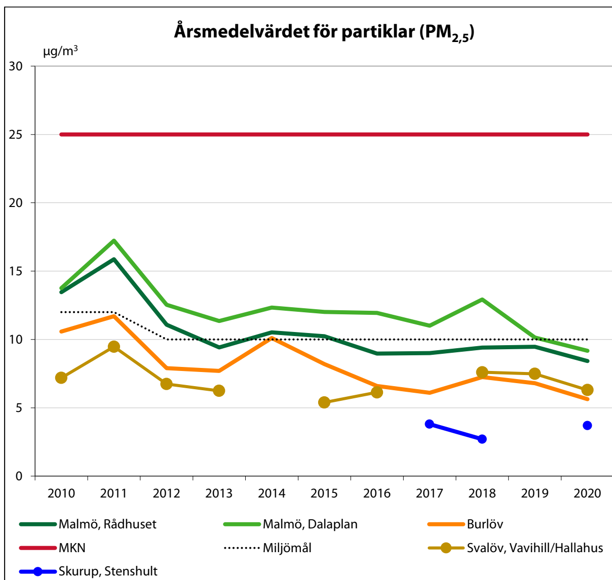
Figur 19. Årsmedelvärdet för partiklar (PM 2,5 ) under tio år inom samverkansområdet Skåne.
