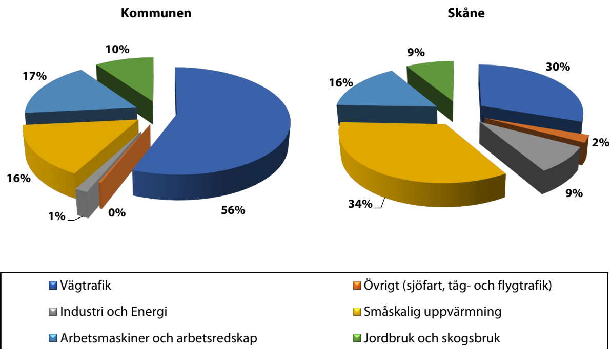
Figur 22. Procentuell fördelning av utsläppskällor för partiklar (PM 2,5 ) i kommunen jämfört med Skåne.
