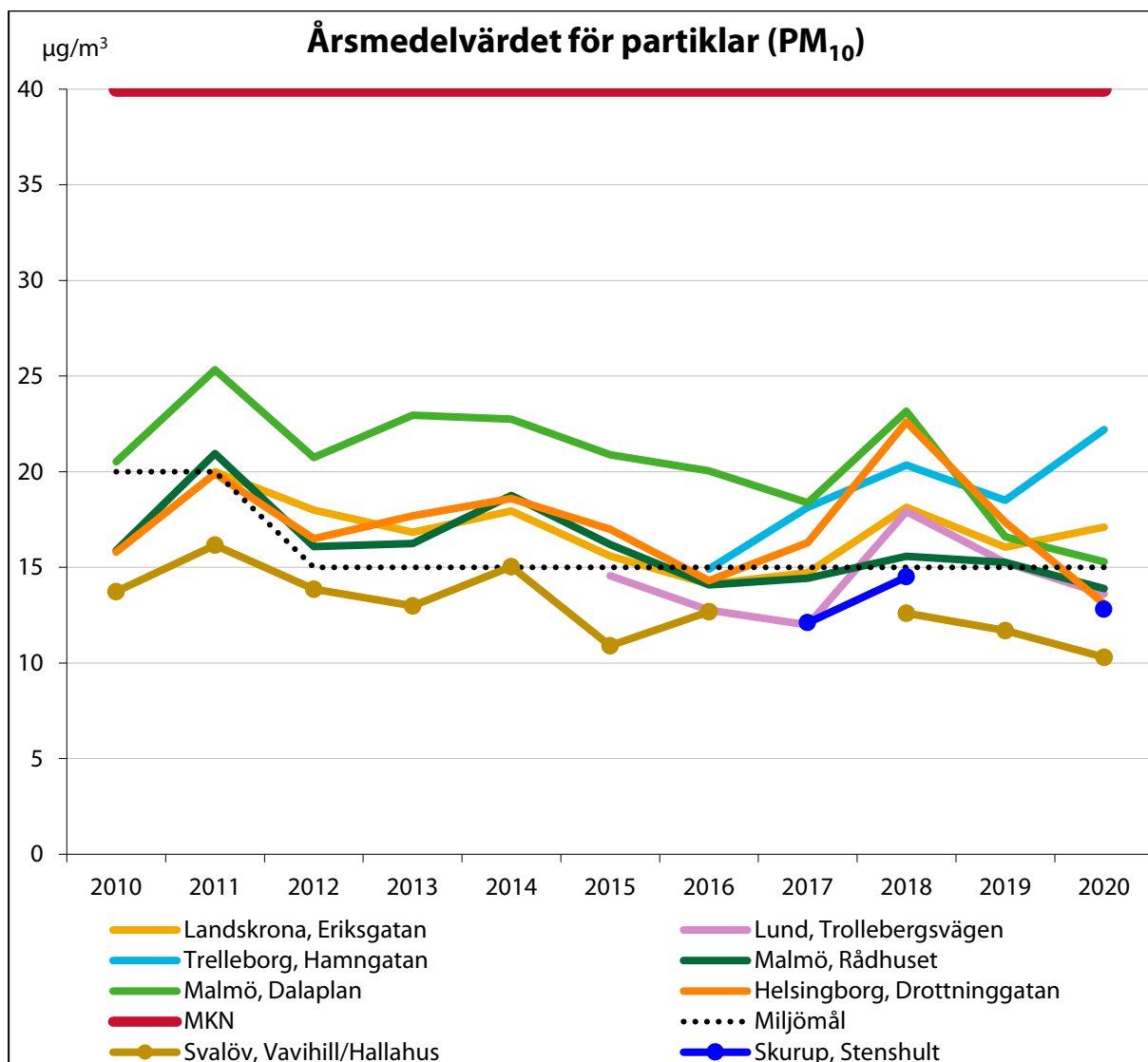
Figur 13. Årsmedelvärdet för partiklar (PM 10 ) under tio år inom samverkansområdet Skåne.
