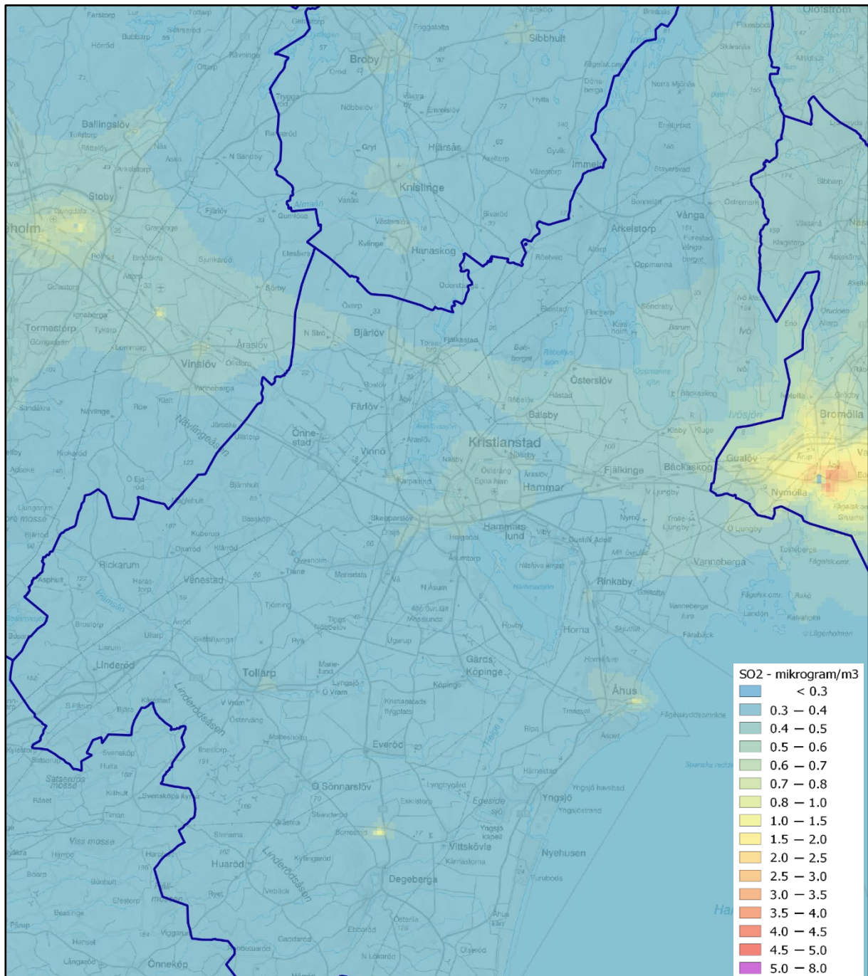
Figur 26. Beräknade årsmedelvärden av svaveldioxid (SO 2 ) inom kommunen (µg/m 3 ).
