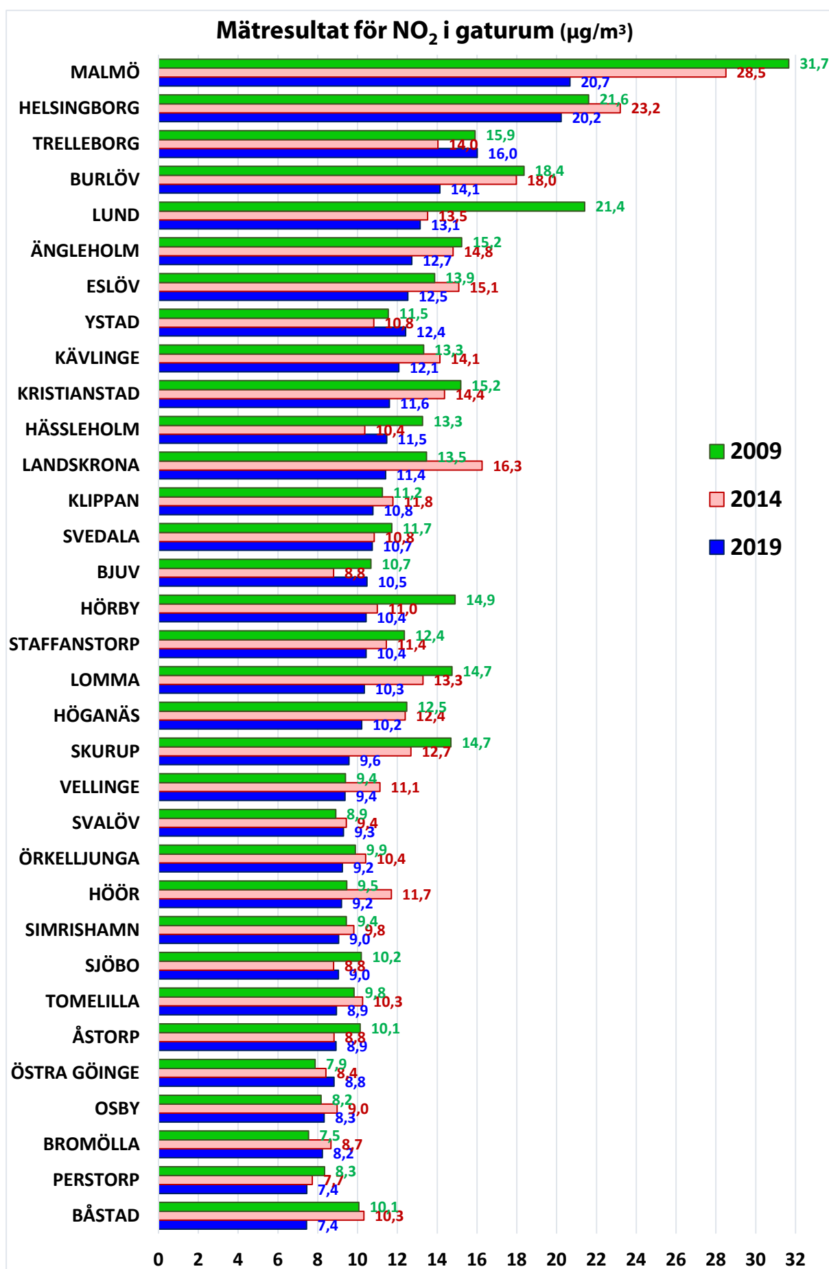
Figur 4. Uppmätta halter av kvävedioxid (NO 2 ) i gaturum under 2009, 2014 samt 2019 inom samverkansområdet Skåne.
