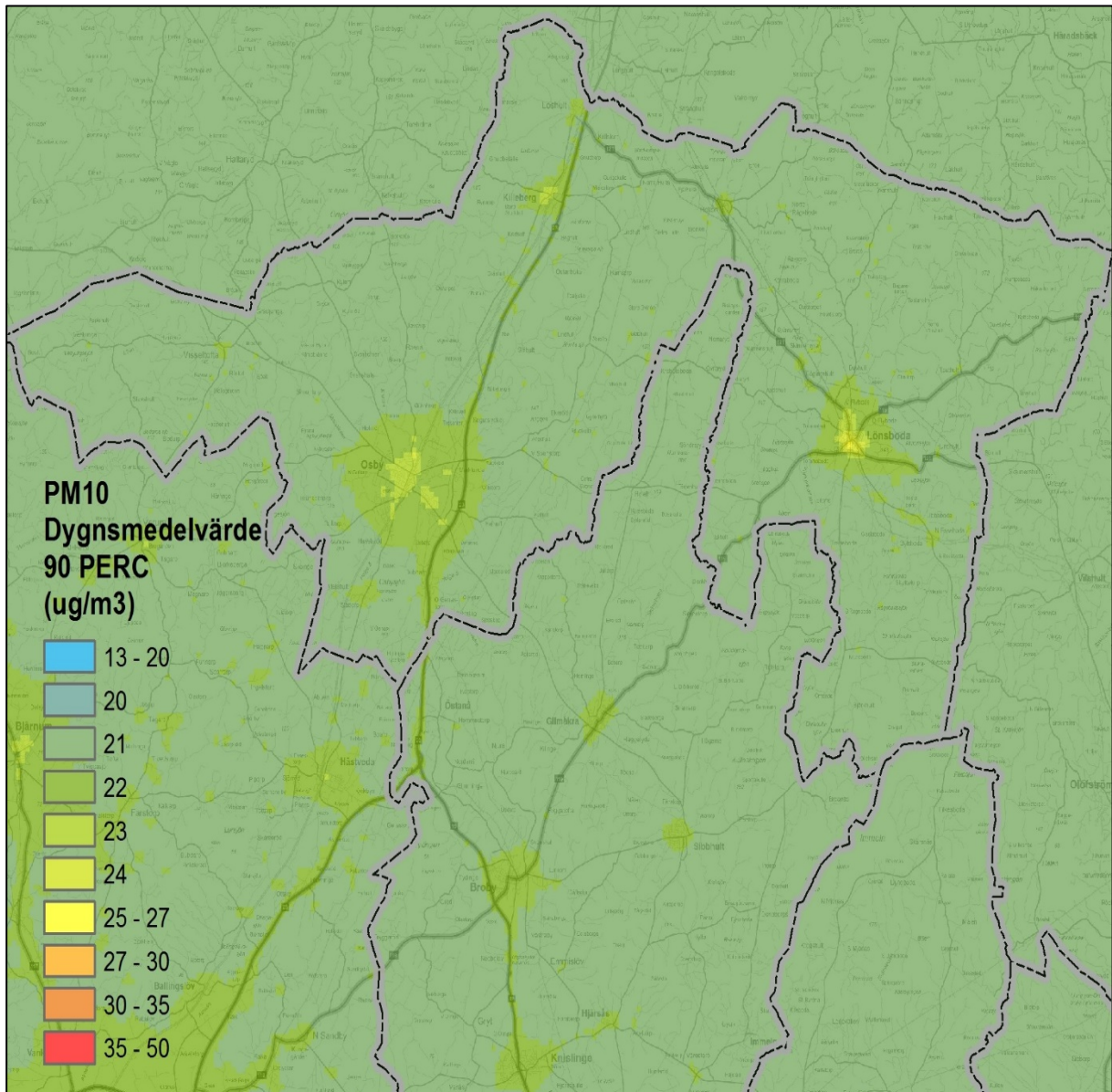
Figur 18. Beräknade dygnsmedelvärden av partiklar PM_{10} inom kommunen ( \mu\text{g}/\text{m}^3 ).
