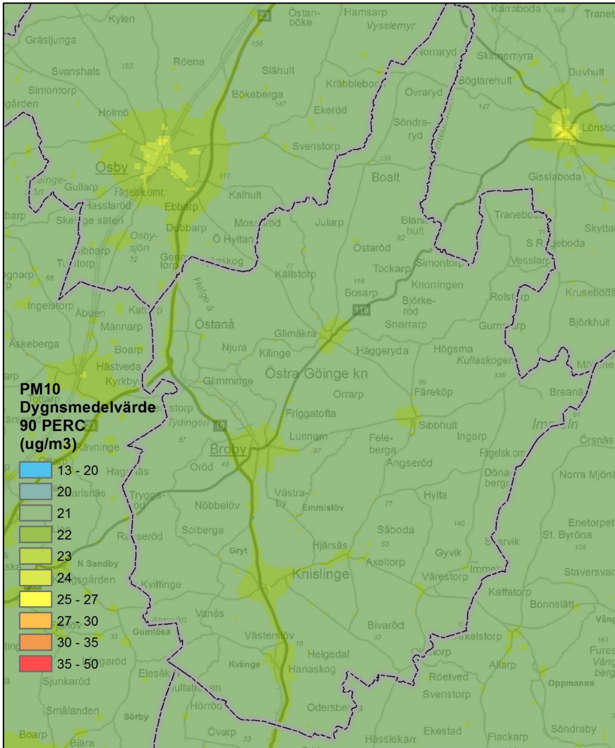
Figur 18. Beräknade dygnsmedelvärderna av partiklar PM 10 inom kommunen (µg/m 3 ).
