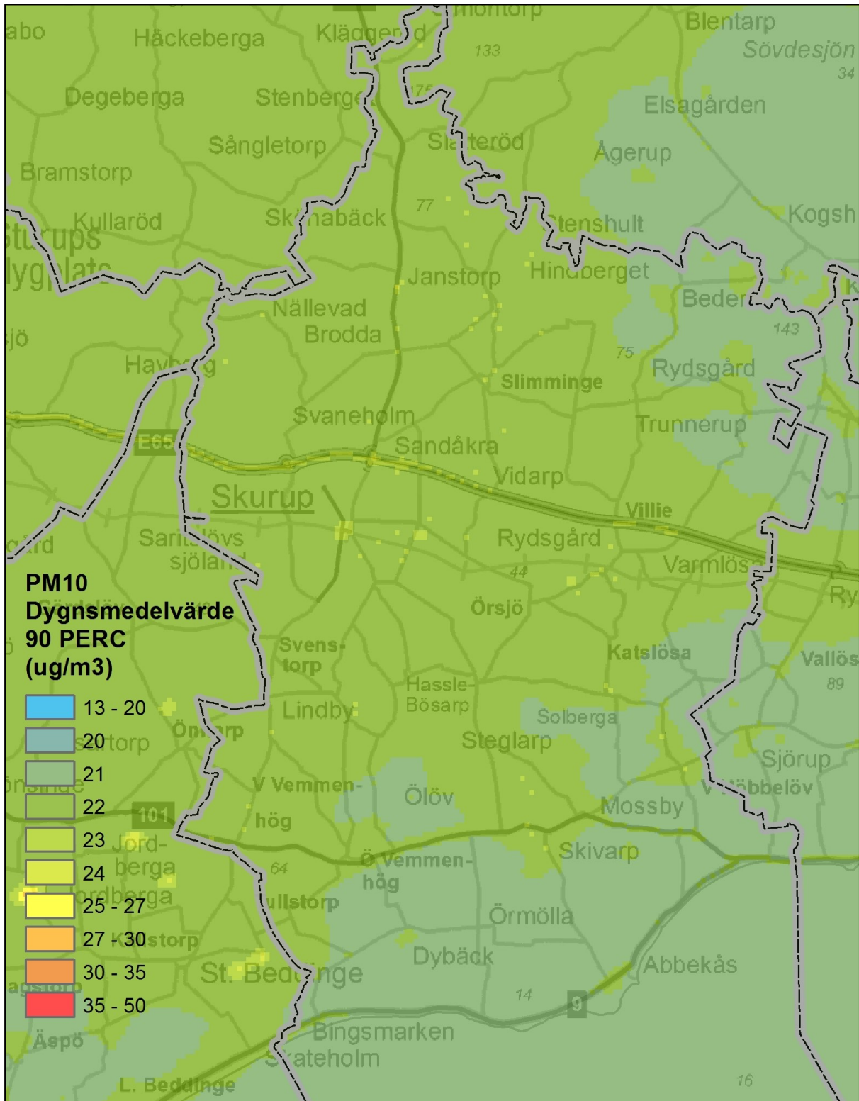
Figur 18. Beräknade dygnsmedelvärden av partiklar PM_{10} inom kommunen ( \mu\text{g}/\text{m}^3 ).
