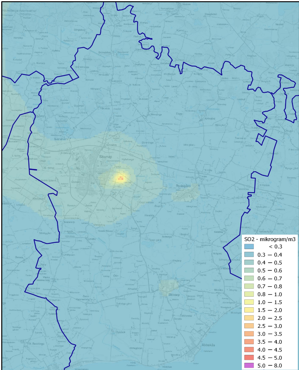
Figur 26. Beräknade årsmedelvärden av svaveldioxid (SO 2 ) inom kommunen (µg/m 3 ).
