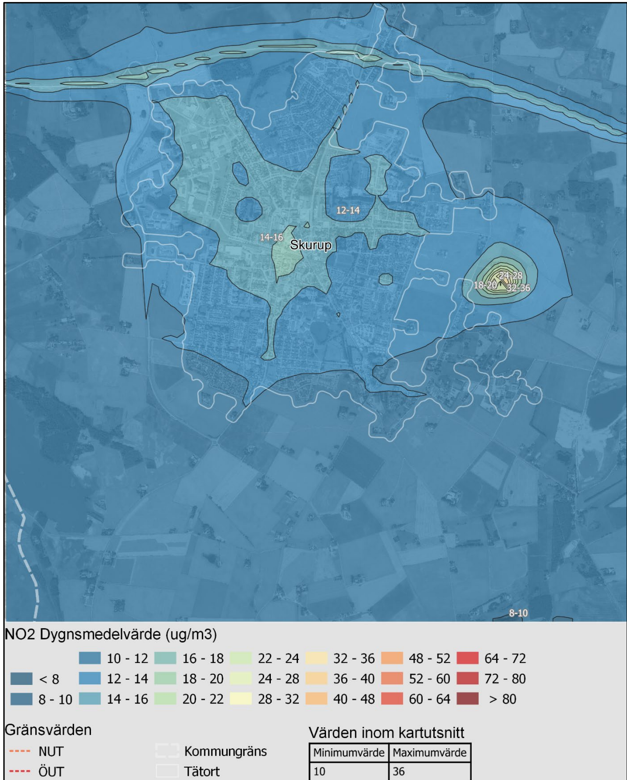
Figur 8. Beräknade dygnsmedelvärden av kvävedioxid i tätorten ( \mu\text{g}/\text{m}^3 ).
