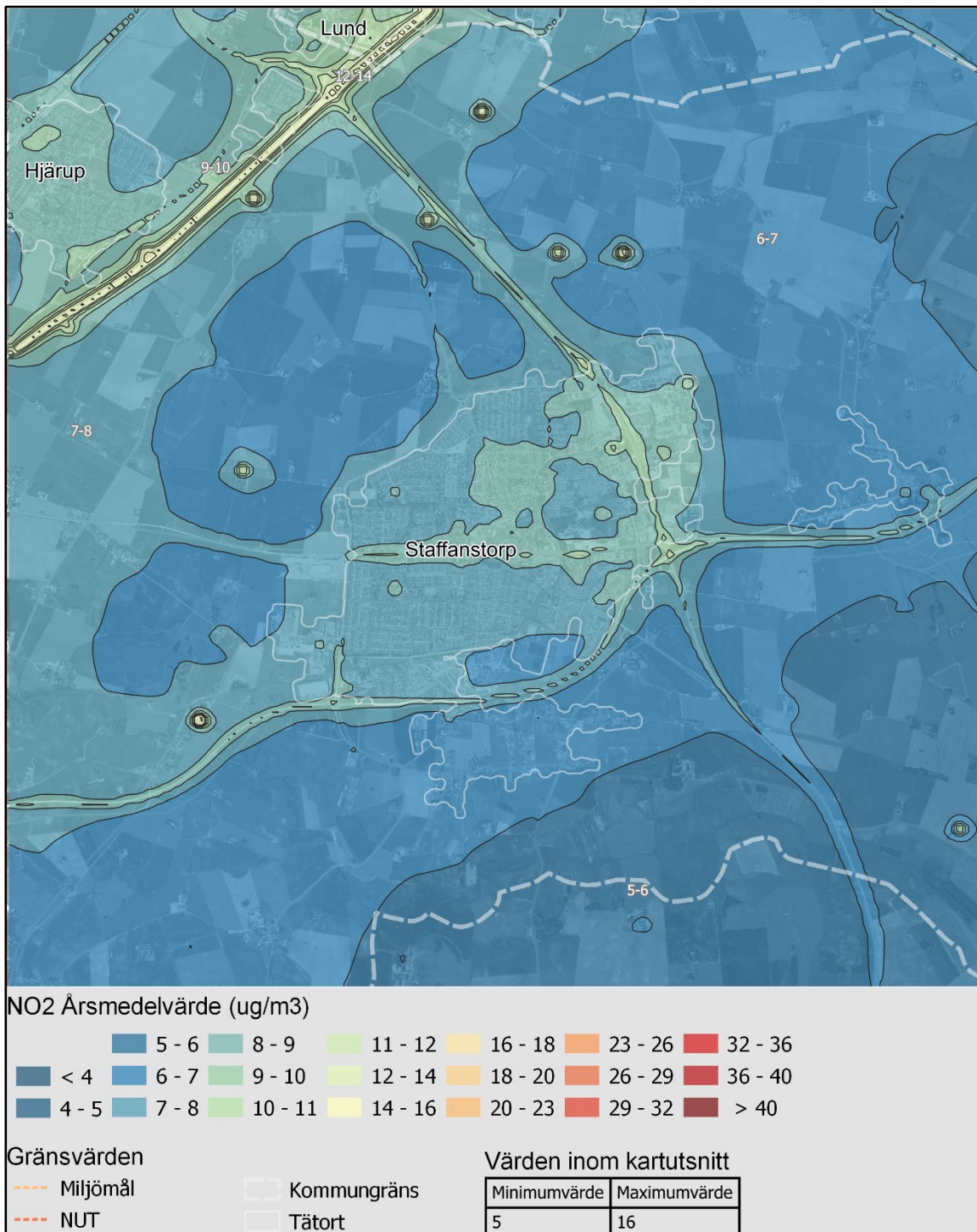
Figur 6. Beräknade årsmedelvärderna av kvävedioxid i tätorten (µg/m 3 ).
