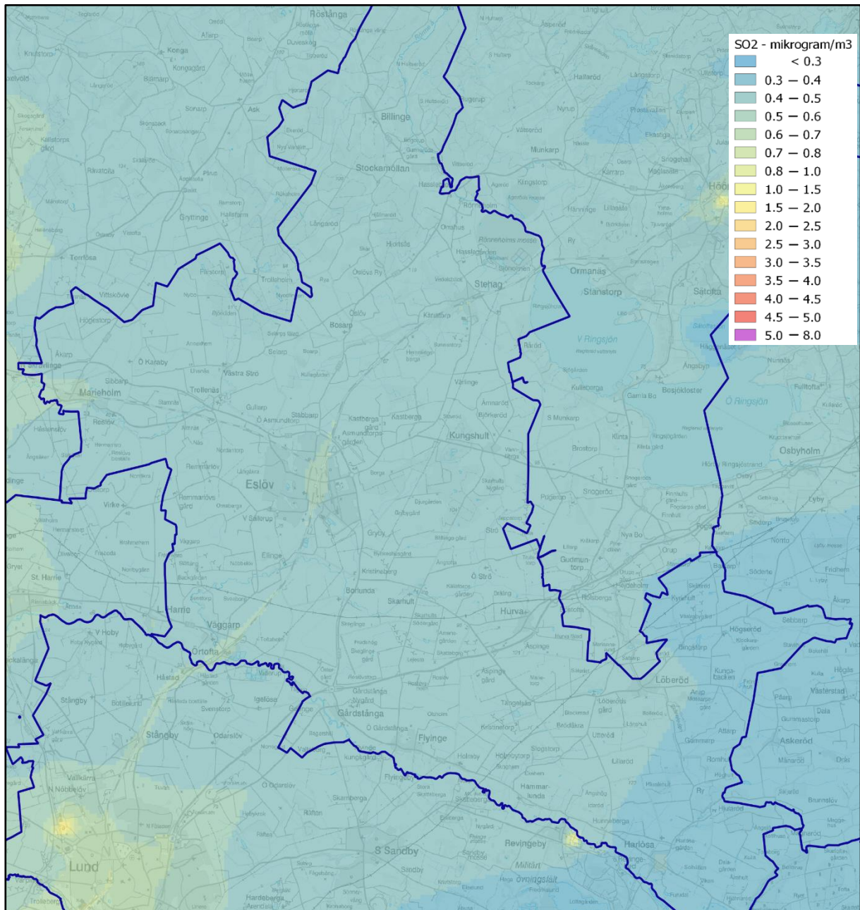
Figur 27. Beräknade årsmedelvärden av svaveldioxid (SO 2 ) inom kommunen (µg/m 3 ).
