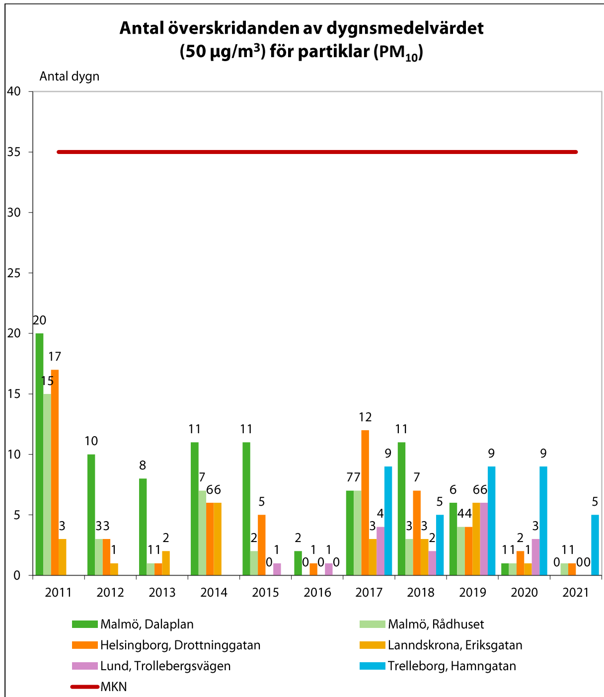
Figur 15. Antal överskridanden av dygnsmedelvärdet för partiklar (PM 10 ) under tio år inom samverkansområdet Skåne.
