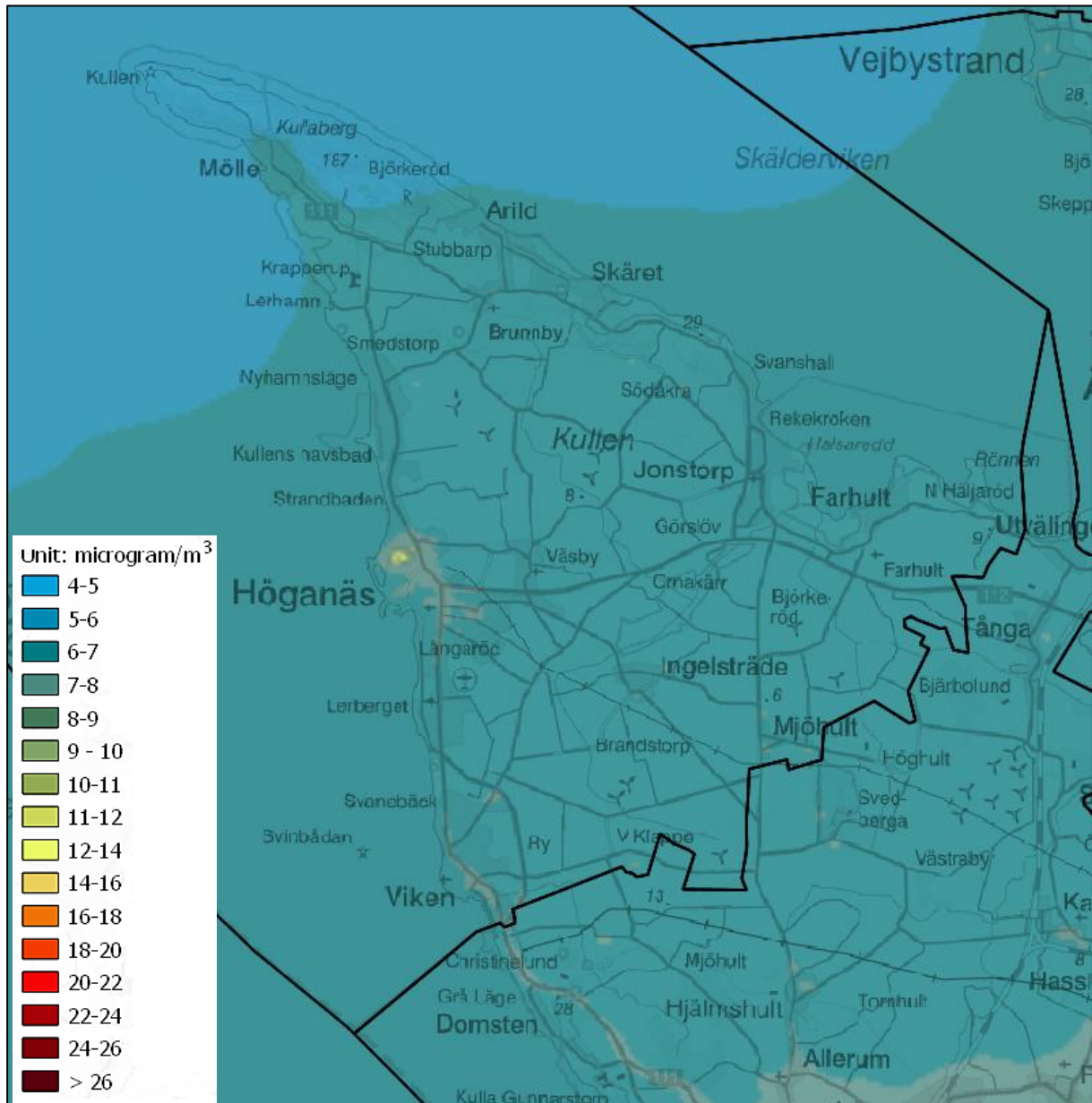
Figur 22. Beräknade årsmedelvärden av partiklar PM_{2.5} inom kommunen ( \mu\text{g}/\text{m}^3 ).
