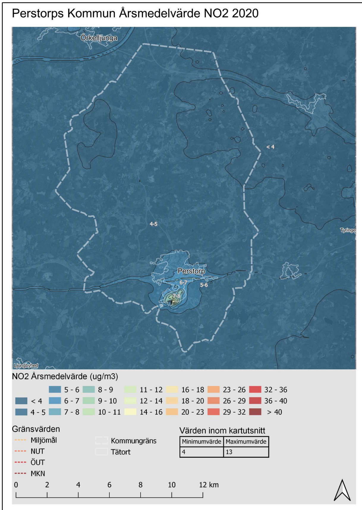
Figur 7. Beräknade årsmedelvärden av kvävedioxid inom kommunen ( \mu\text{g}/\text{m}^3 ).
