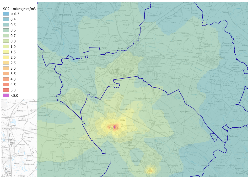
Figur 6. Karta som visar årsmedelvärdet av SO x för år 2019 i Åstorp.
