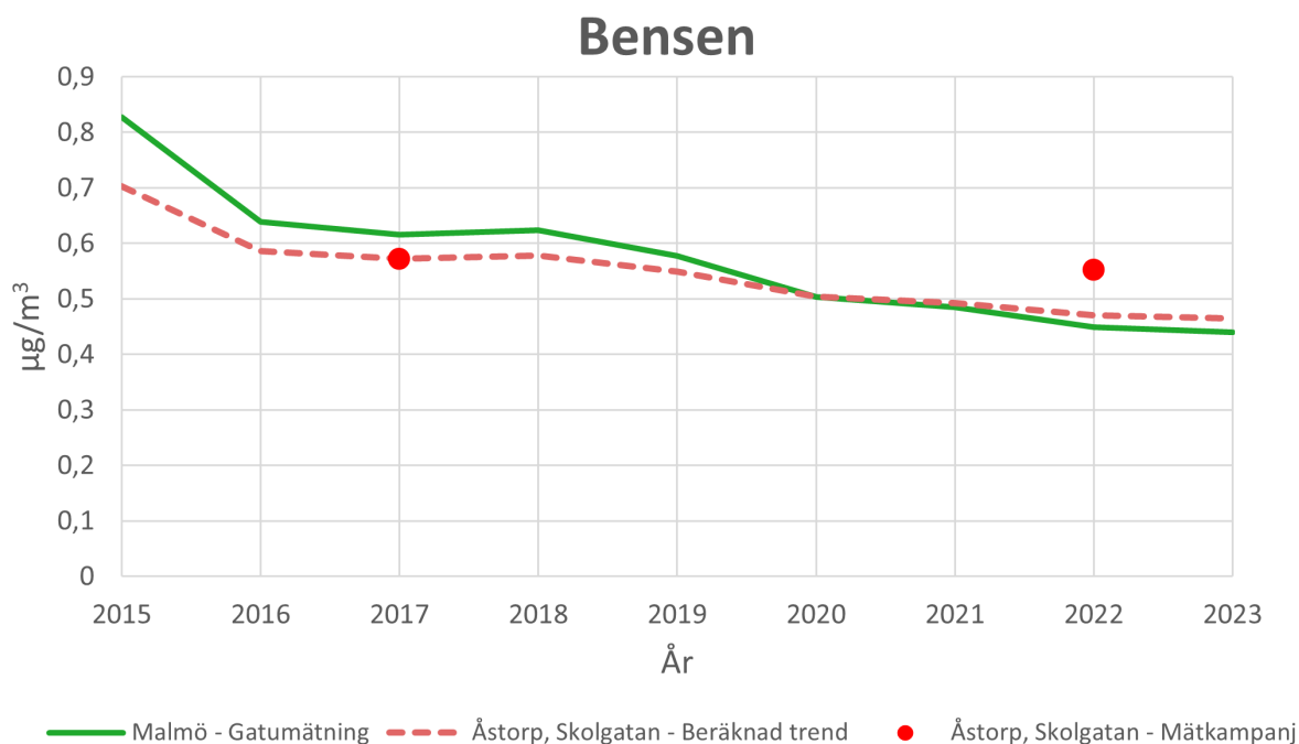
Figur 19. Visar hur koncentrationen av bensen i atmosfären har förändrats för år 2015 – 2023 i Åstorp jämfört med Malmö.
