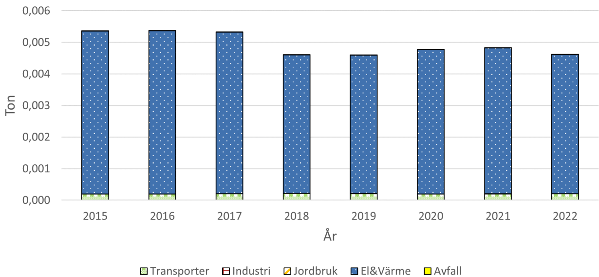
Figur 18. Visar utsläppskällorna av PAH för Åstorp, vilket inkluderar bens(a)pyren. beräknat värde från SMHI.
