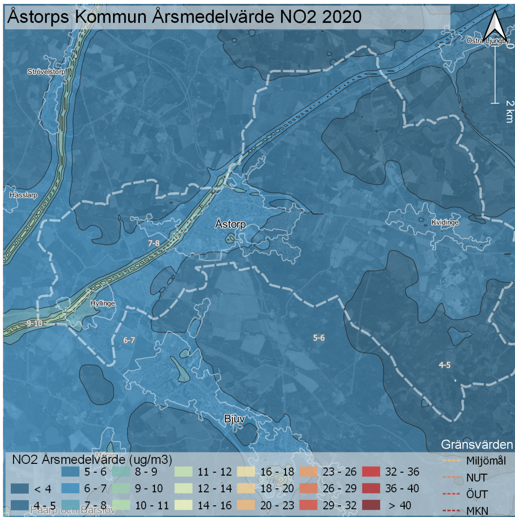
Figur 3. Karta som visar årsmedelvärden av NO 2 för år 2020 i Åstorp kommun.
