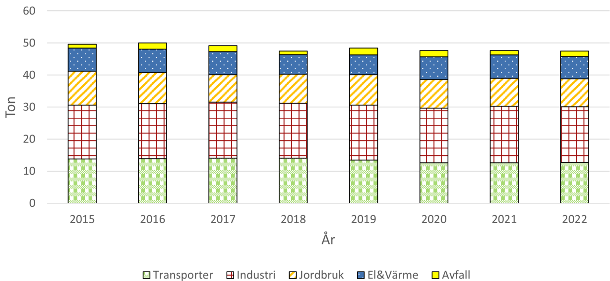
Figur 9. Visar utsläppskällorna av PM10 för Åstorp, beräknat värde från SMHI.
