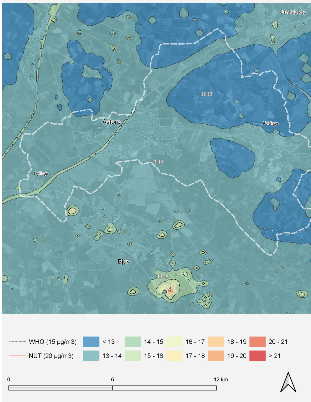
Figur 8. Karta som visar årsmedelvärdet av PM10 för år 2021 i Åstorp.
