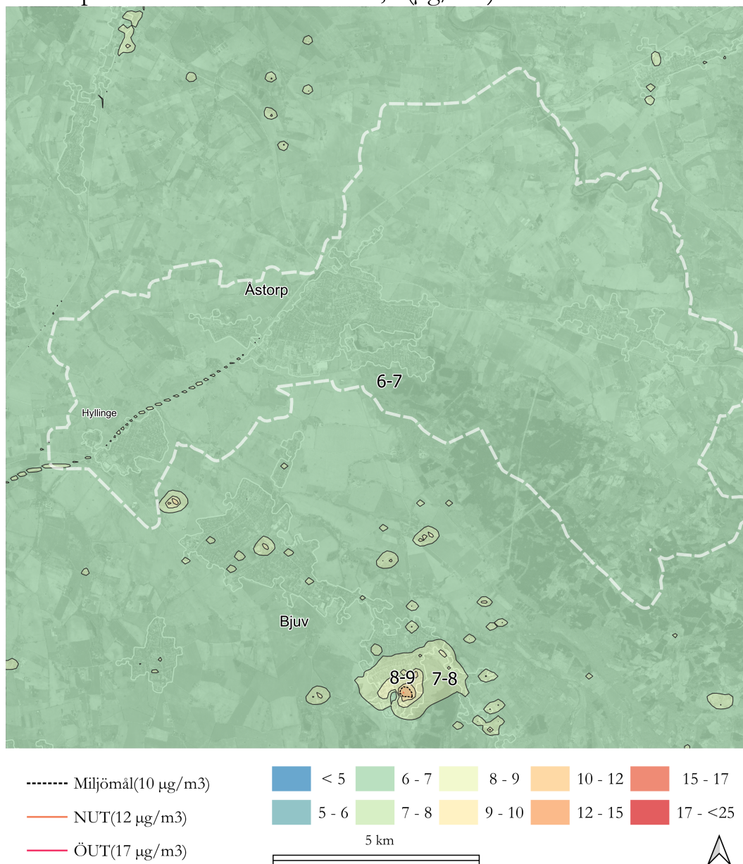
Figur 11. Karta som visar årsmedelvärdet av PM2.5 för år 2022 i Åstorp.
