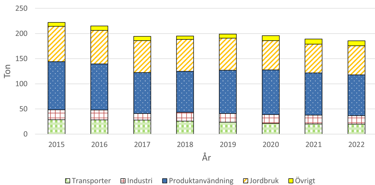
Figur 20. Visar utsläppskällorna av VOC för Åstorp, beräknat värde från SMHI.
