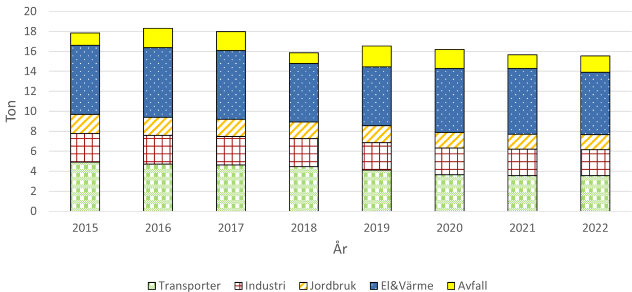
Figur 12. Visar utsläppskällorna av PM2.5 för Åstorp, beräknat värde från SMHI.
