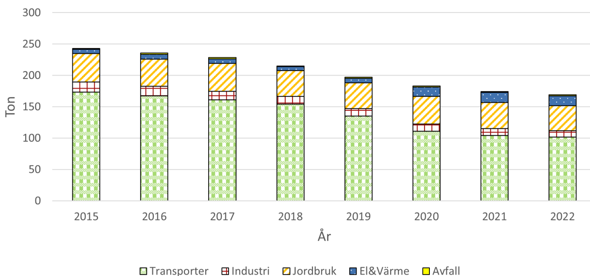
Figur 4. Visar utsläppskällorna av NO x för Åstorp, beräknat värde från SMHI.
