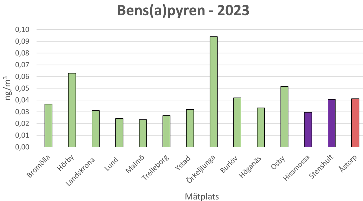
Figur 17. Visar hur medelkoncentrationen av bens(a)pyren i atmosfären såg ut i elva kommuner, två bakgrundstationer samt ett skattat värde för Åstorp i Skåne under en tremånaders mätkampanj i 2023.
