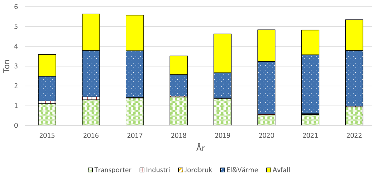
Figur 6. Visar utsläppskällorna av SO x för Åstorp, beräknat värde från SMHI.
