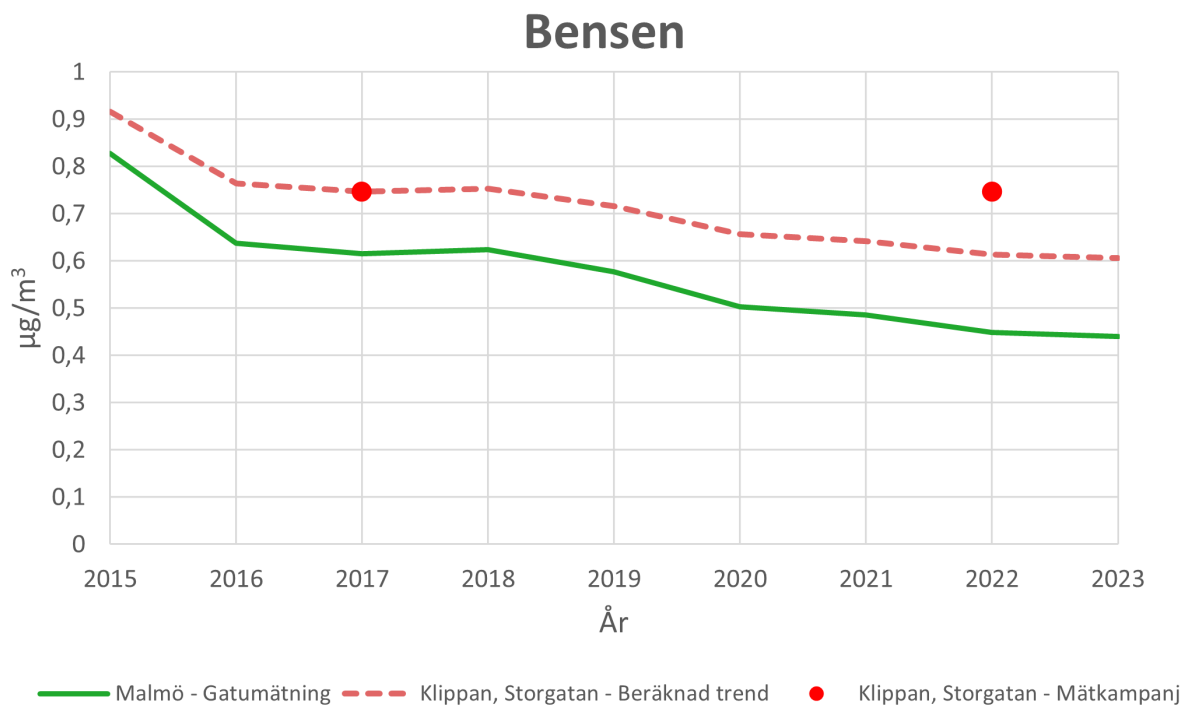
Figur 19. Visar hur koncentrationen av bensen i atmosfären har förändrats för år 2015 – 2023 i Klippan jämfört med Malmö.
