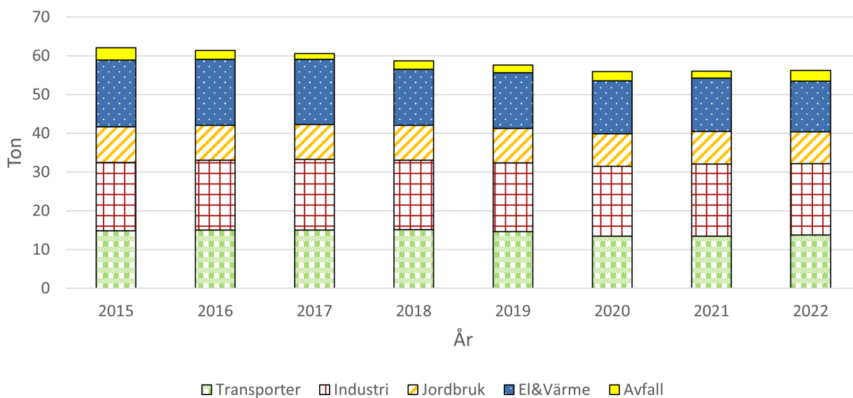
Figur 9. Visar utsläppskällorna av PM10 för Klippan, beräknat värde från SMHI.
