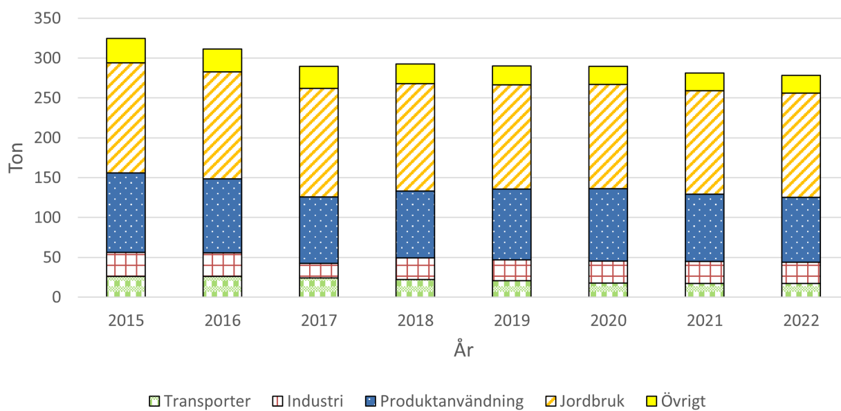
Figur 20. Visar utsläppskällorna av VOC för Klippan, beräknat värde från SMHI.
