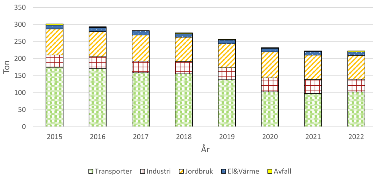
Figur 4. Visar utsläppskällorna av NO x för Klippan, beräknat värde från SMHI.
