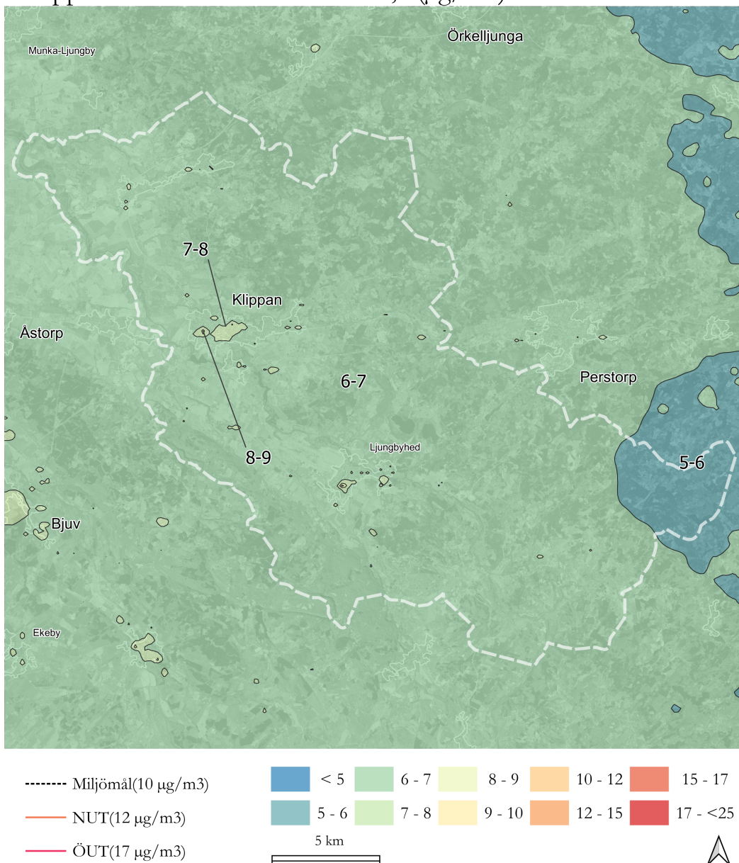
Figur 11. Karta som visar årsmedelvärdet av PM 2.5 för år 2022 i Klippan.
