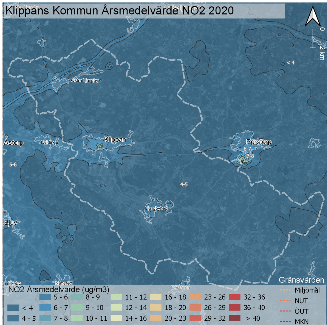
Figur 3. Karta som visar årsmedelvärden av NO 2 för år 2020 i Klippans kommun.
