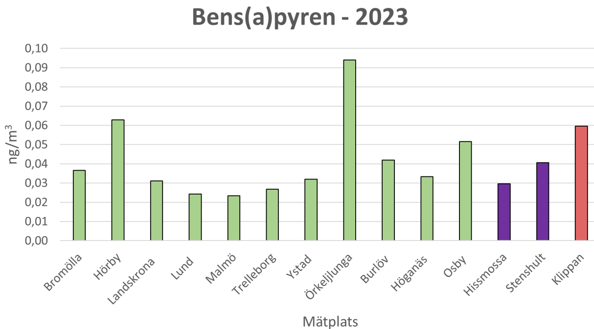
Figur 17. Visar hur medelkoncentrationen av bens(a)pyren i atmosfären såg ut i elva kommuner, två bakgrundstationer samt ett skattat värde för Klippan i Skåne under en tremånaders mätkampanj i 2023.
