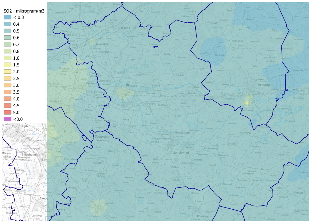
Figur 6. Karta som visar årsmedelvärde av SO x för år 2019 i Klippan.
