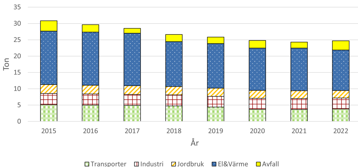
Figur 12. Visar utsläppskällorna av PM2.5 för Klippans, beräknat värde från SMHI.
