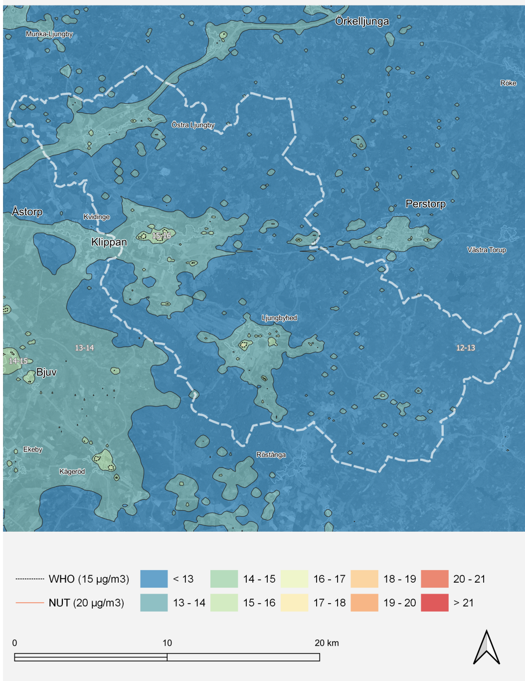
Figur 8. Karta som visar årsmedelvärdet av PM10 för år 2021 i Klippan.
