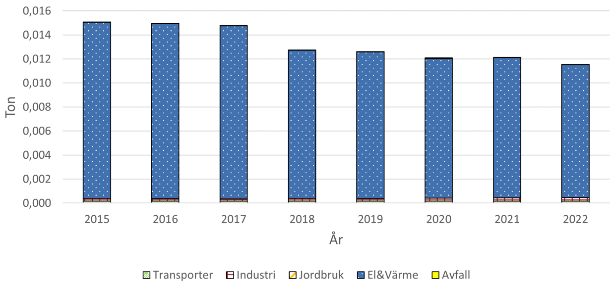
Figur 18. Visar utsläppskällorna av PAH för Klippan, vilket inkluderar bens(a)pyren. beräknat värde från SMHI.
