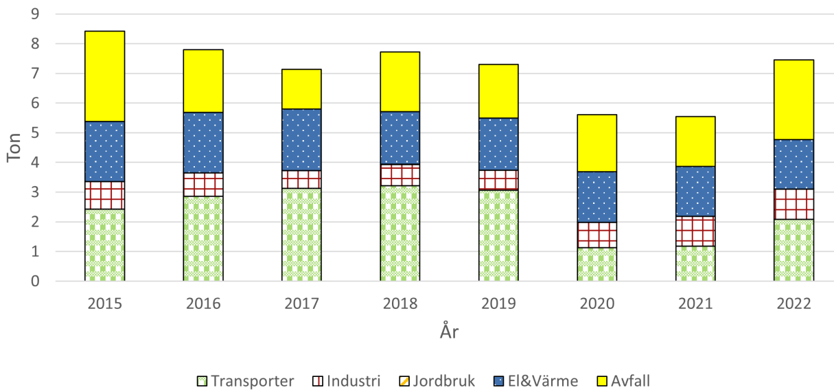
Figur 6. Visar utsläppskällorna av SO x för Klippan, beräknat värde från SMHI.
