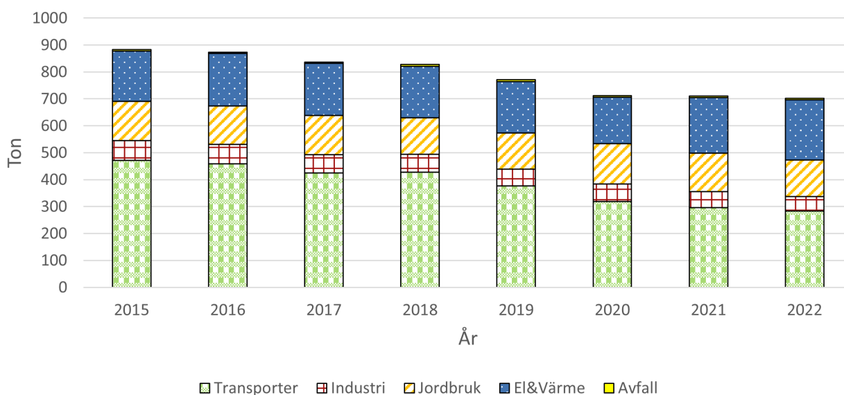
Figur 4. Visar utsläppskällorna av NO x för Lund, beräknat värde från SMHI.
