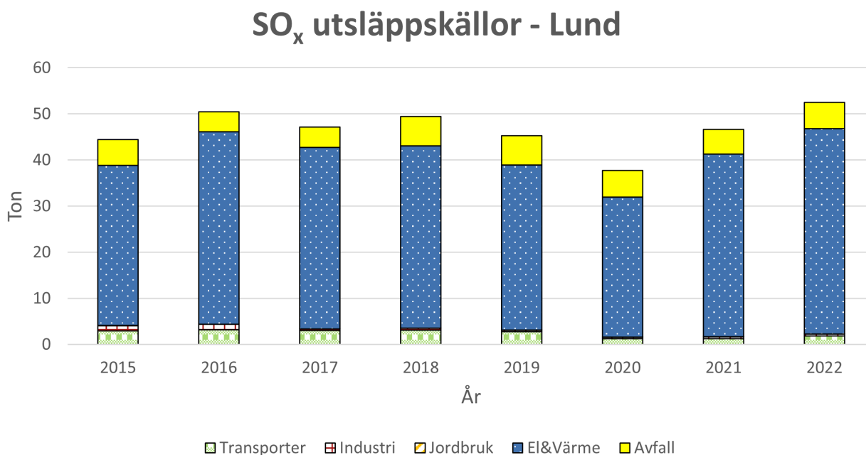
Figur 6. Visar utsläppskällorna av SO x för Lund, beräknat värde från SMHI.
