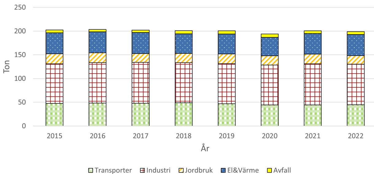
Figur 9. Visar utsläppskällorna av PM10 för Lund, beräknat värde från SMHI.
