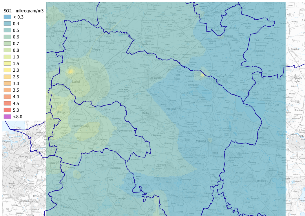
Figur 6. Karta som visar årsmedelvärdet av SO x för år 2019 i Lund.
