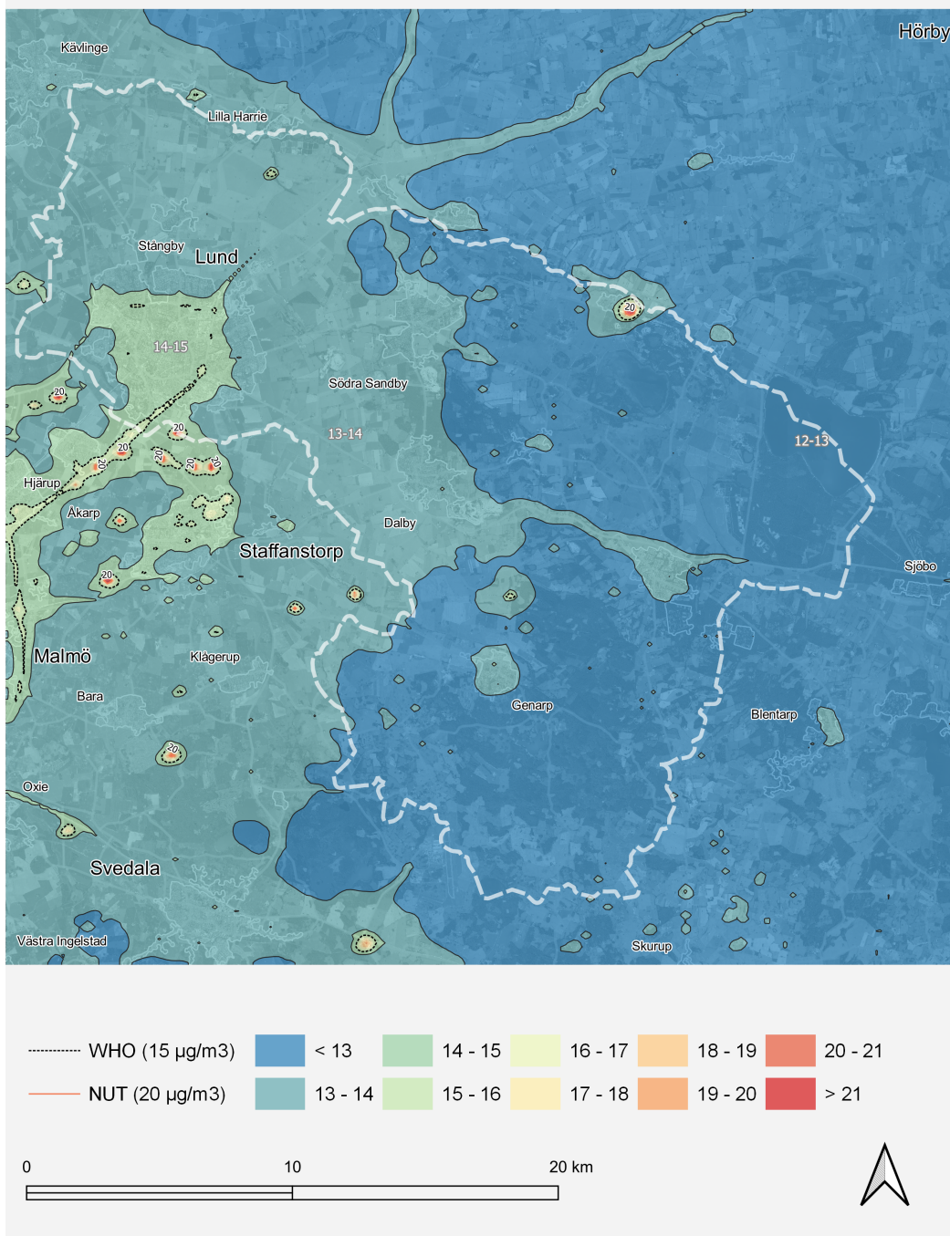
Figur 8. Karta som visar årsmedelvärdet av PM10 för år 2021 i Lund.
