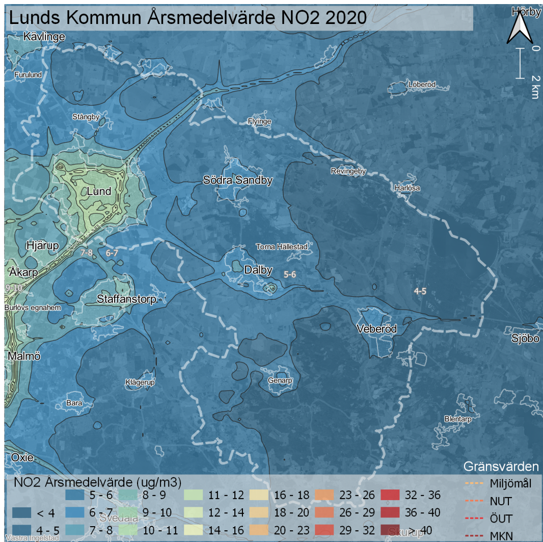
Figur 3. Karta som visar årsmedelvärden av NO 2 för år 2020 i Lunds kommun.
