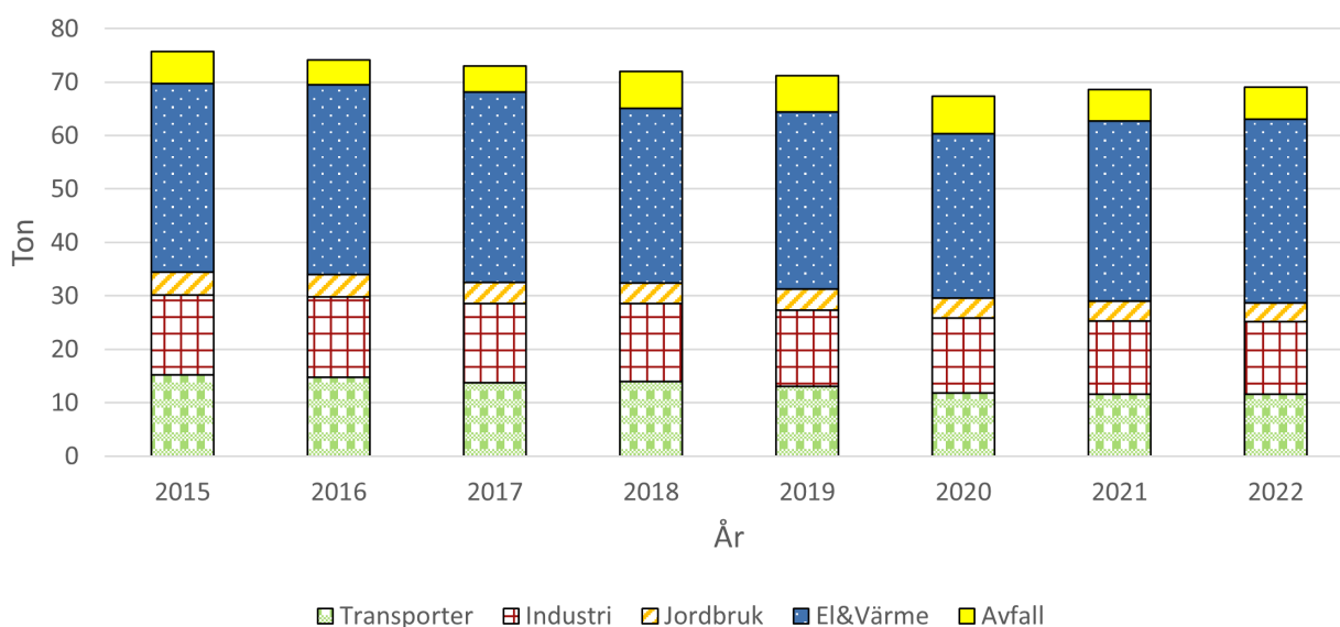
Figur 12. Visar utsläppskällorna av PM2.5 för Lund, beräknat värde från SMHI.
