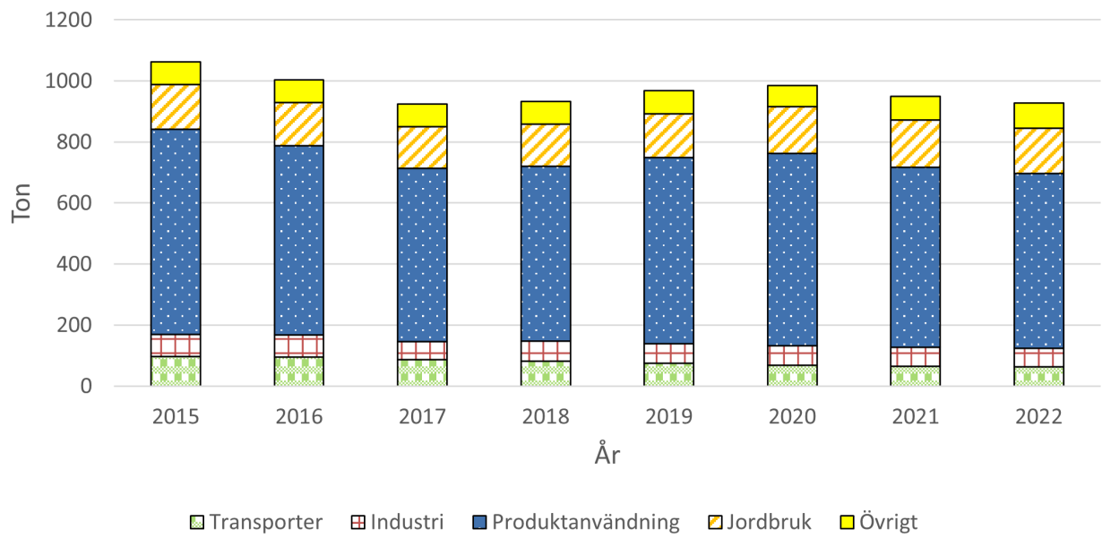
Figur 20. Visar utsläppskällorna av VOC för Lund, beräknat värde från SMHI.
