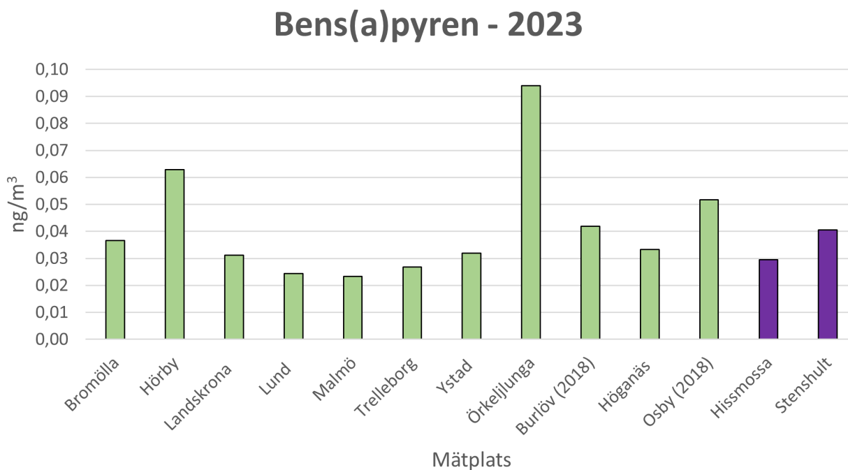
Figur 17. Visar hur medelkoncentrationen av bens(a)pyren i atmosfären såg ut i elva kommuner, två bakgrundstationer samt ett skattat värde för Lund i Skåne under en tremånaders mätkampanj i 2023.
