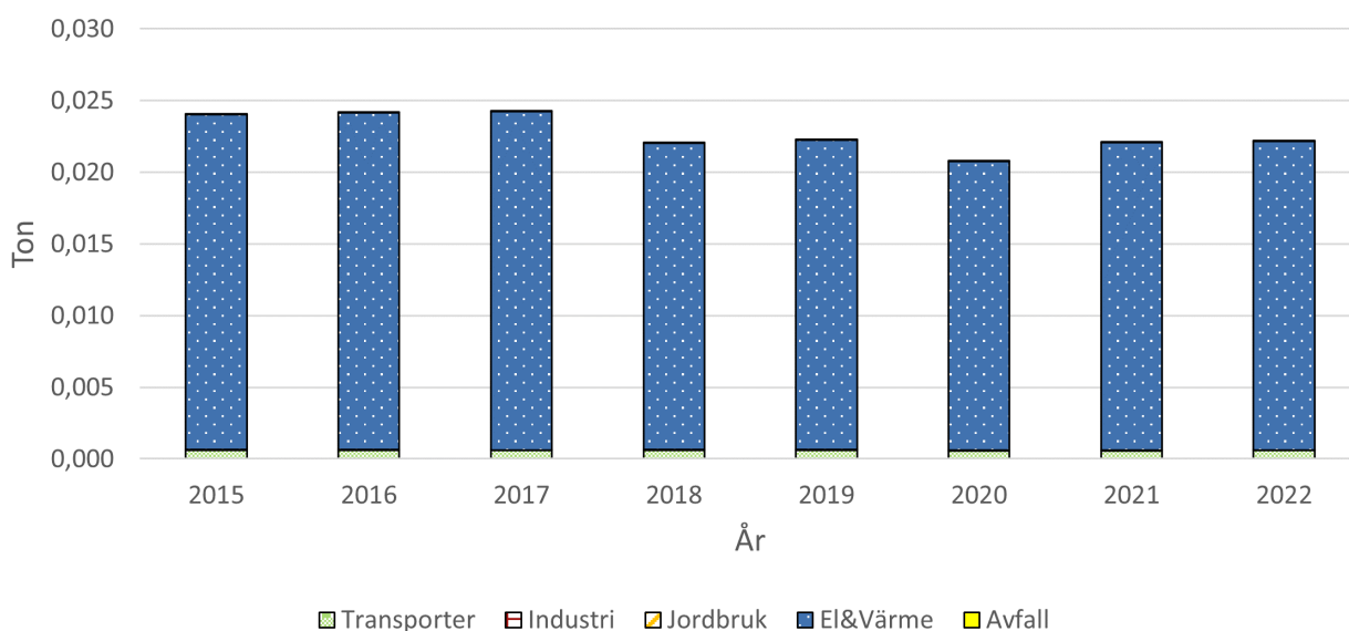
Figur 18. Visar utsläppskällorna av PAH för Lund, vilket inkluderar bens(a)pyren. beräknat värde från SMHI.
