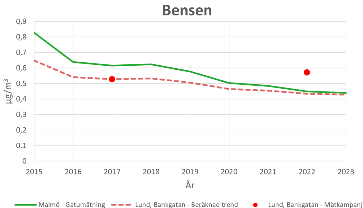
Figur 19. Visar hur koncentrationen av bensen i atmosfären har förändrats för år 2015 – 2023 i Lund jämfört med Malmö.
