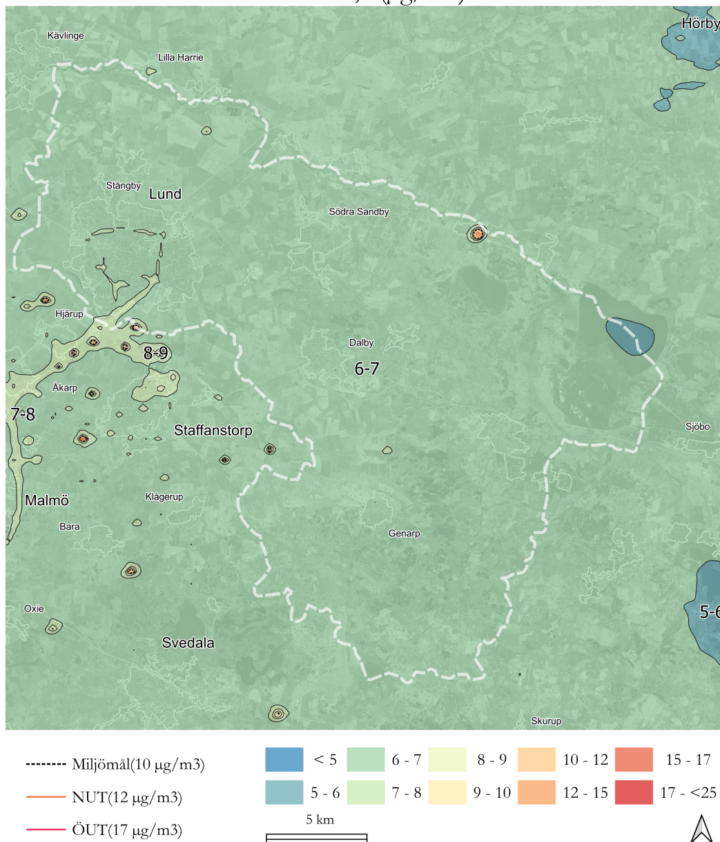
Figur 11. Karta som visar årsmedelvärdet av PM2.5 för år 2022 i Lund.
