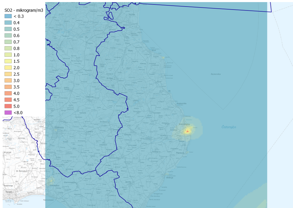
Figur 6. Karta som visar årsmedelvärdet av SO x för år 2019 i Simrishamn.
