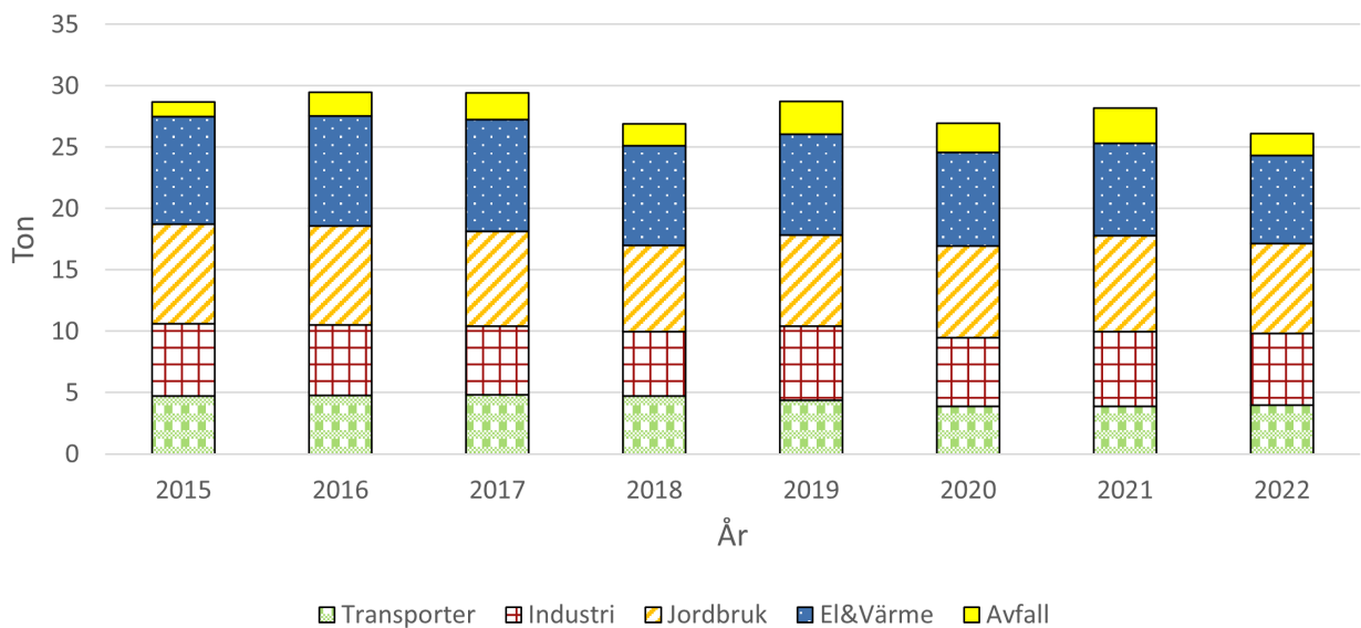
Figur 13. Visar utsläppskällorna av PM2.5 för Simrishamn, beräknat värde från SMHI.
