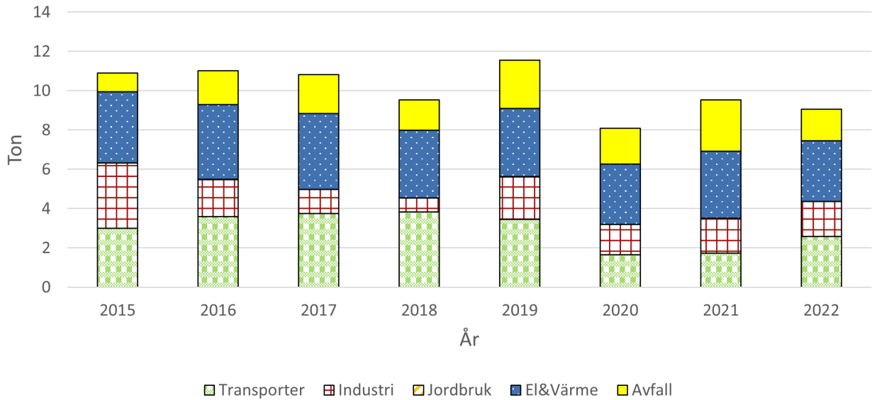
Figur 7. Visar utsläppskällorna av SO x för Simrishamn, beräknat värde från SMHI.
