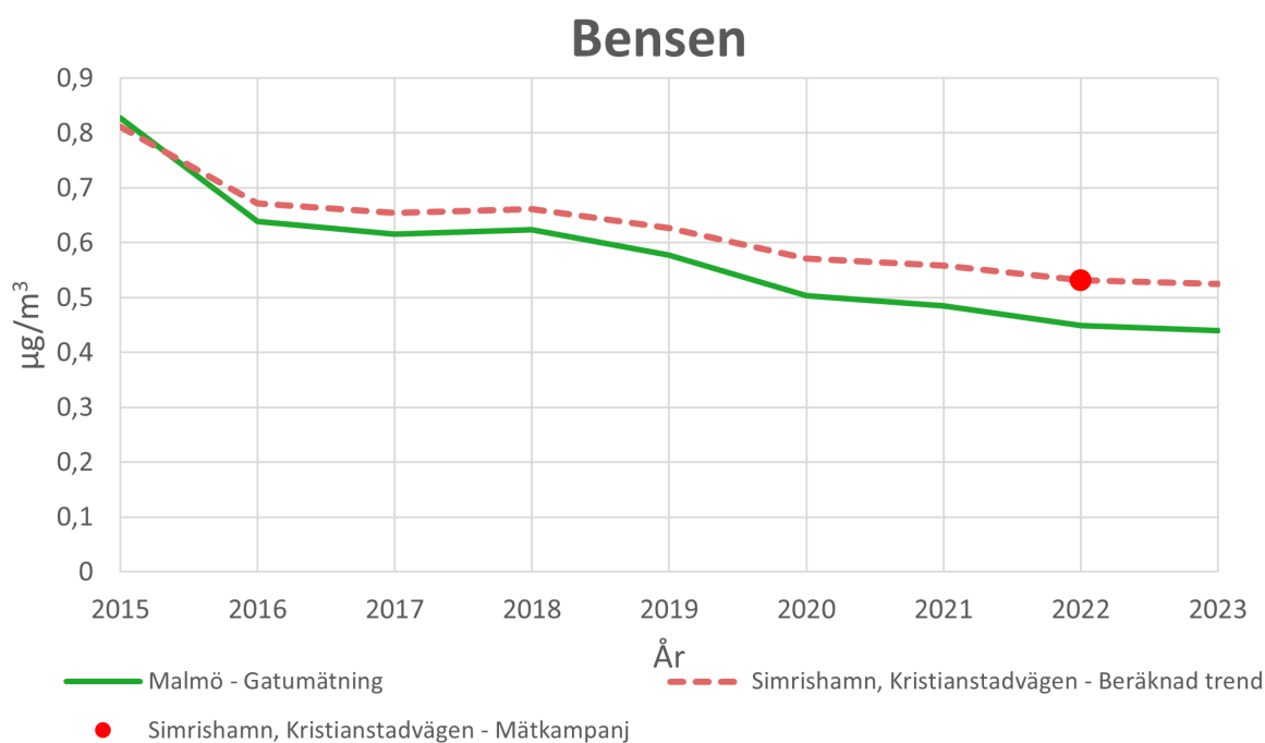
Figur 20. Visar hur koncentrationen av bensen i atmosfären har förändrats för år 2015 – 2023 i Simrishamn jämfört med Malmö.
