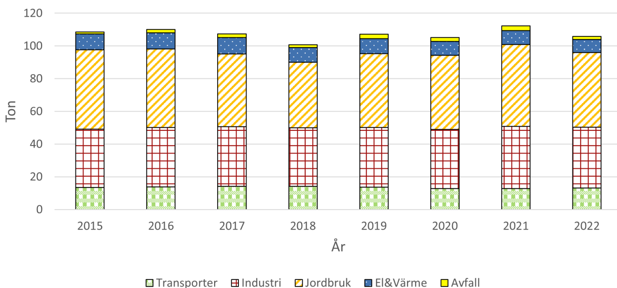
Figur 10. Visar utsläppskällorna av PM10 för Simrishamn, beräknat värde från SMHI.
