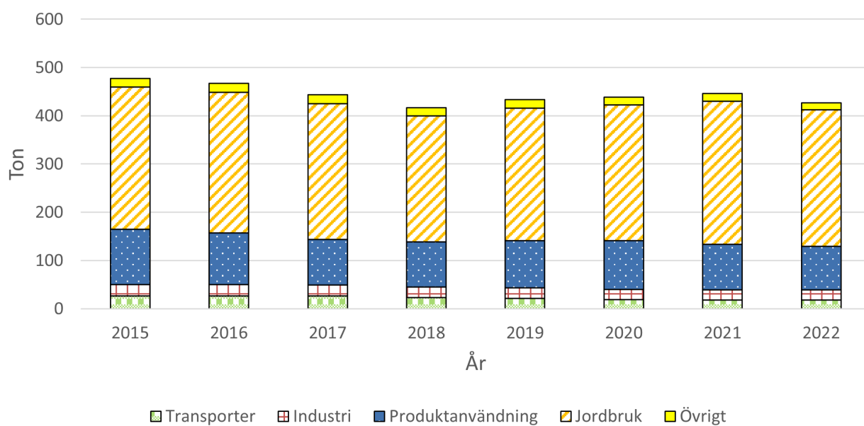
Figur 21. Visar utsläppskällorna av VOC för Simrishamn, beräknat värde från SMHI.
