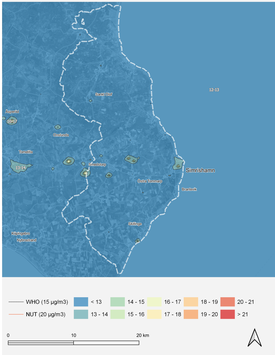
Figur 9. Karta som visar årsmedelvärdet av PM10 för år 2021 i Simrishamn.
