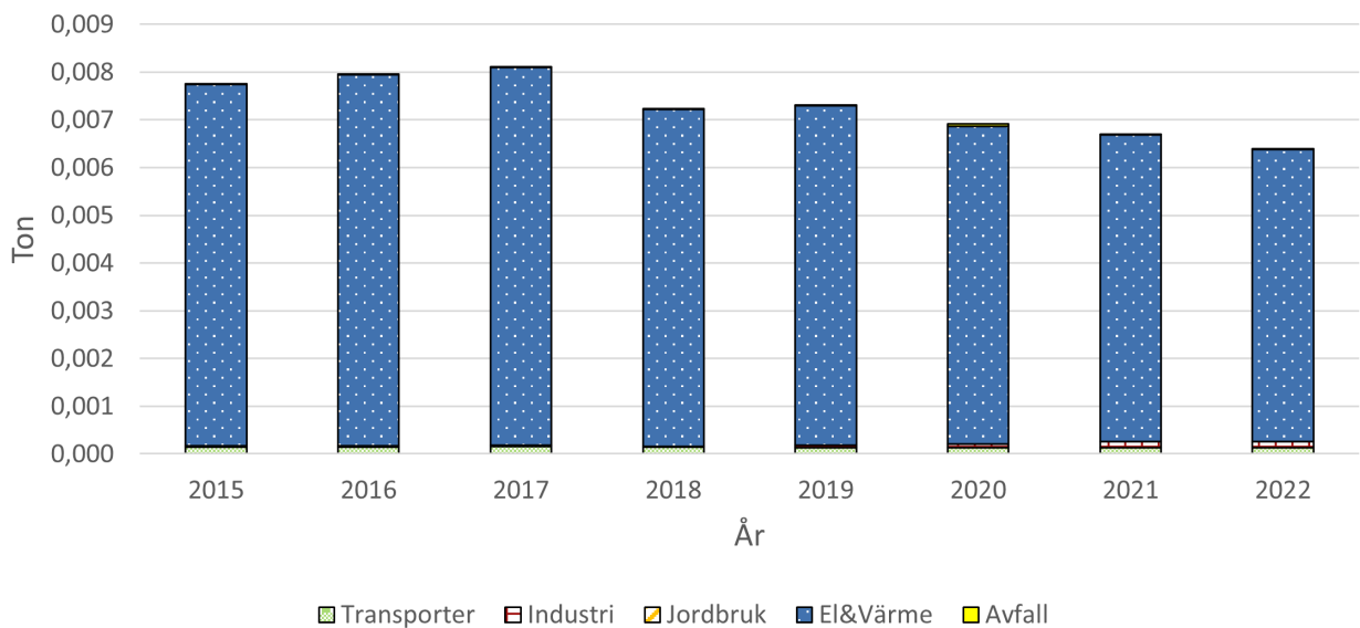
Figur 19. Visar utsläppskällorna av PAH för Simrishamn, vilket inkluderar bens(a)pyren. beräknat värde från SMHI.
