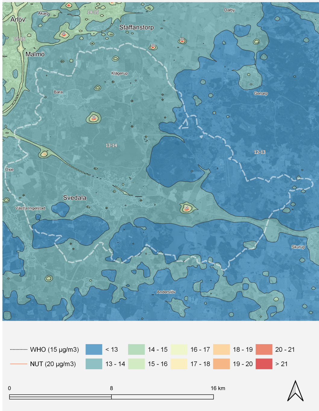
Figur 8. Karta som visar årsmedelvärdet av PM10 för år 2021 i Svedala.
