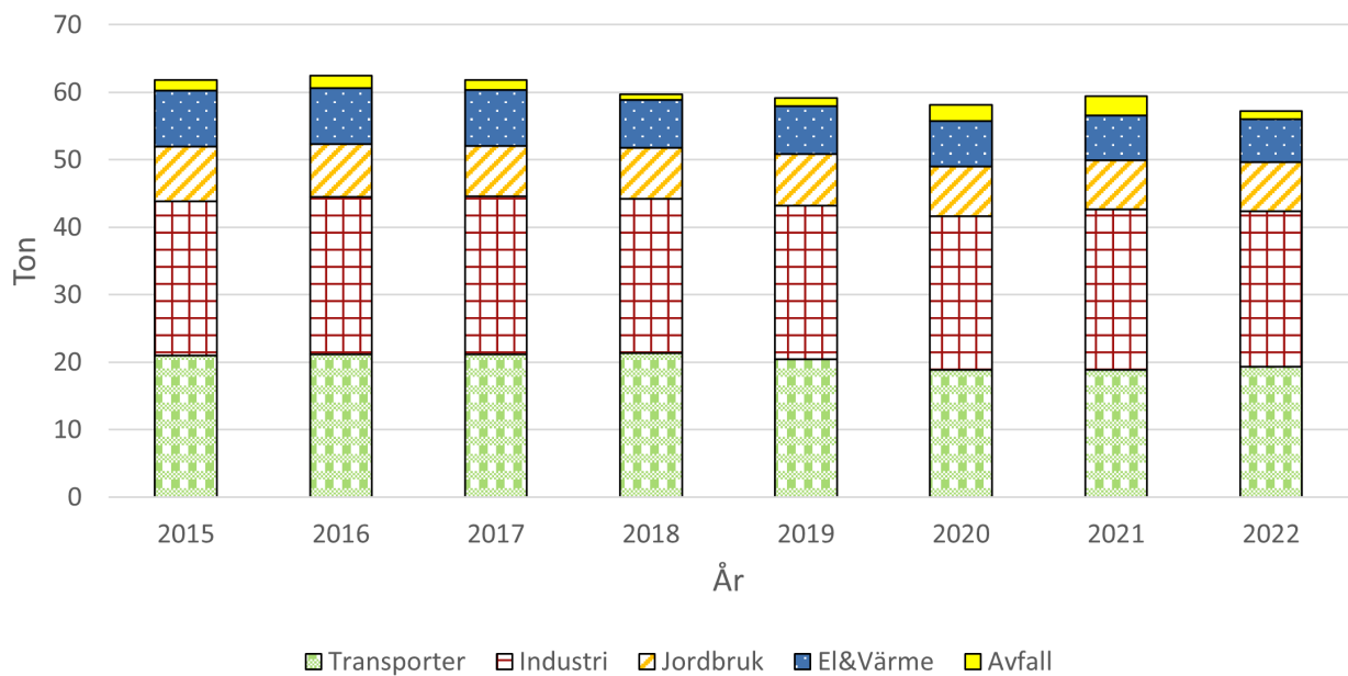
Figur 9. Visar utsläppskällorna av PM10 för Svedala, beräknat värde från SMHI.
