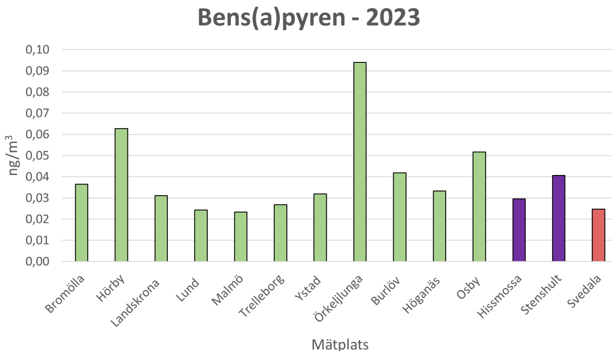
Figur 17. Visar hur medelkoncentrationen av bens(a)pyren i atmosfären såg ut i elva kommuner, två bakgrundstationer samt ett skattat värde för Svedala i Skåne under en tremånaders mätkampanj i 2023.
