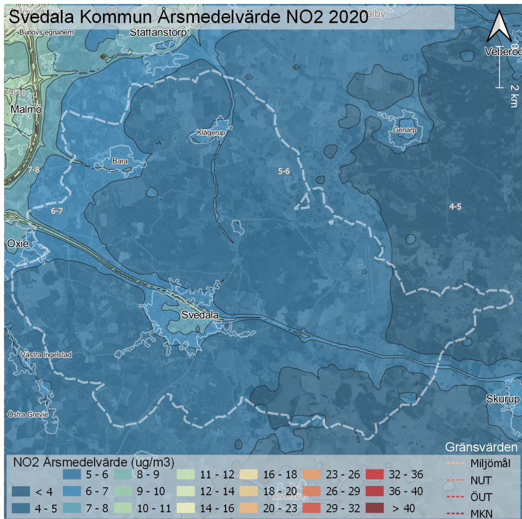
Figur 3. Karta som visar årsmedelvärden av NO 2 för år 2020 i Svedala kommun.
