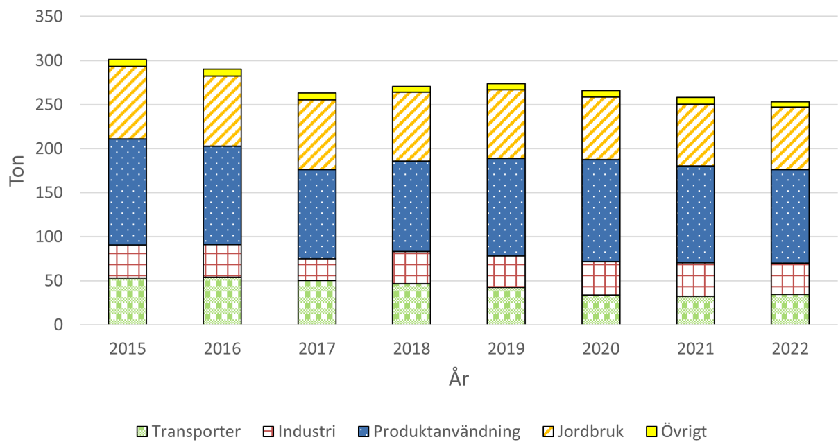
Figur 20. Visar utsläppskällorna av VOC för Svedala, beräknat värde från SMHI.
