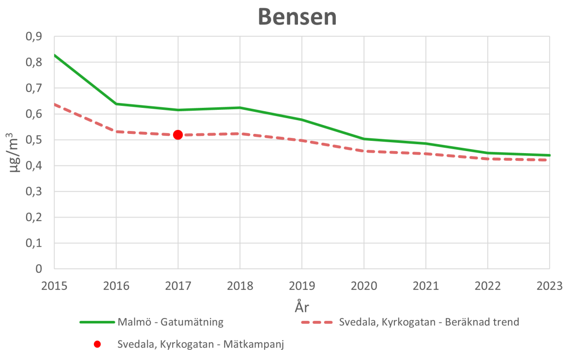
Figur 19. Visar hur koncentrationen av bensen i atmosfären har förändrats för år 2015 – 2023 i Svedala jämfört med Malmö.
