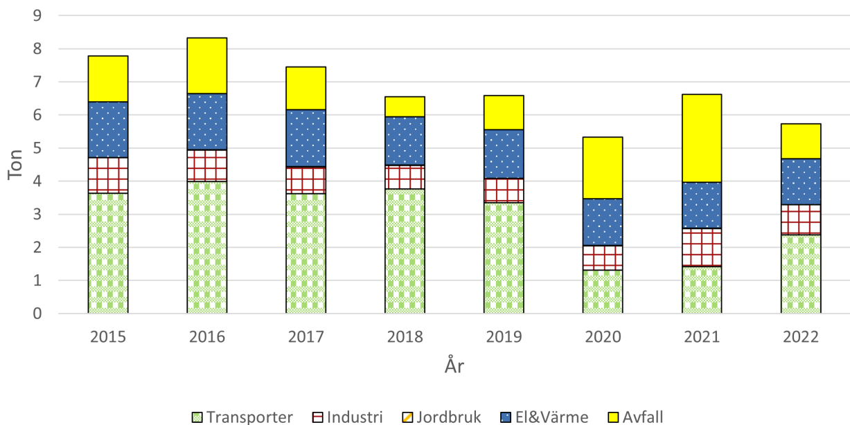
Figur 6. Visar utsläppskällorna av SO x för Svedala, beräknat värde från SMHI.
