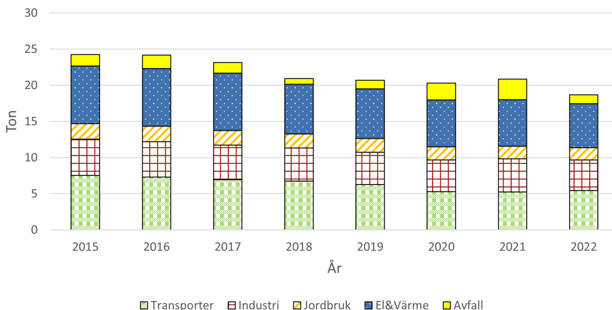
Figur 12. Visar utsläppskällorna av PM2.5 för Svedala, beräknat värde från SMHI.
