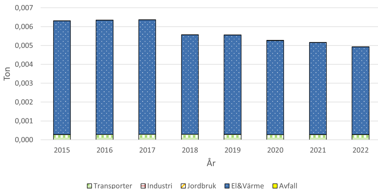
Figur 18. Visar utsläppskällorna av PAH för Svedala, vilket inkluderar bens(a)pyren. beräknat värde från SMHI.
