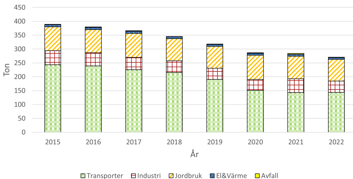
Figur 4. Visar utsläppskällorna av NO x för Svedala, beräknat värde från SMHI.
