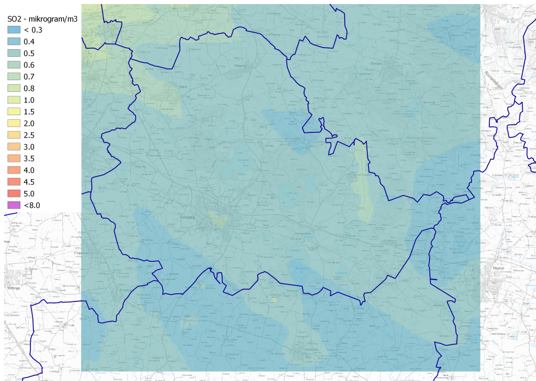
Figur 6. Karta som visar årsmedelvärdet av SO x för år 2019 i Svedala.
