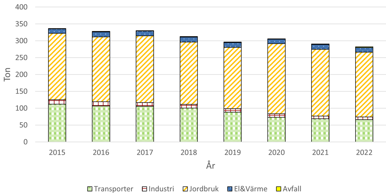
Figur 4. Visar utsläppskällorna av NO x för Tomelilla, beräknat värde från SMHI.
