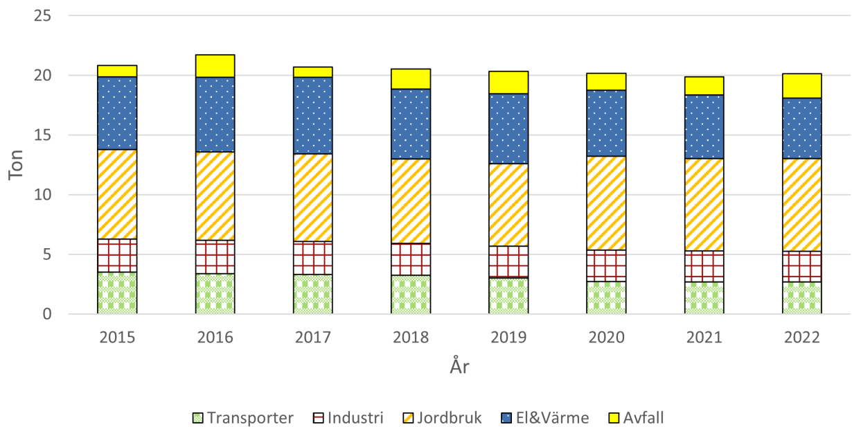
Figur 12. Visar utsläppskällorna av PM2.5 för Tomelilla, beräknat värde från SMHI.
