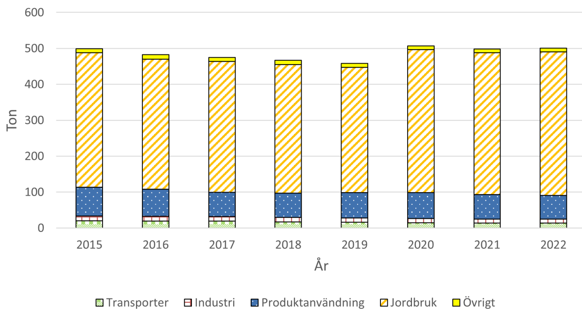
Figur 20. Visar utsläppskällorna av VOC för Tomelilla, beräknat värde från SMHI.
