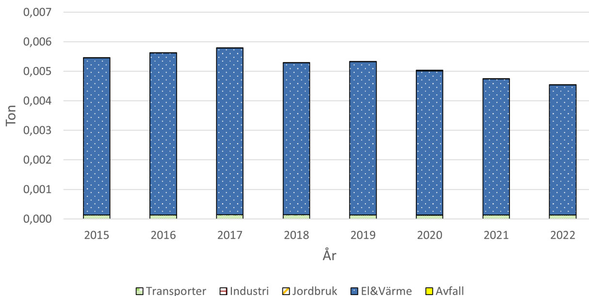
Figur 18. Visar utsläppskällorna av PAH för Tomelilla, vilket inkluderar bens(a)pyren. beräknat värde från SMHI.
