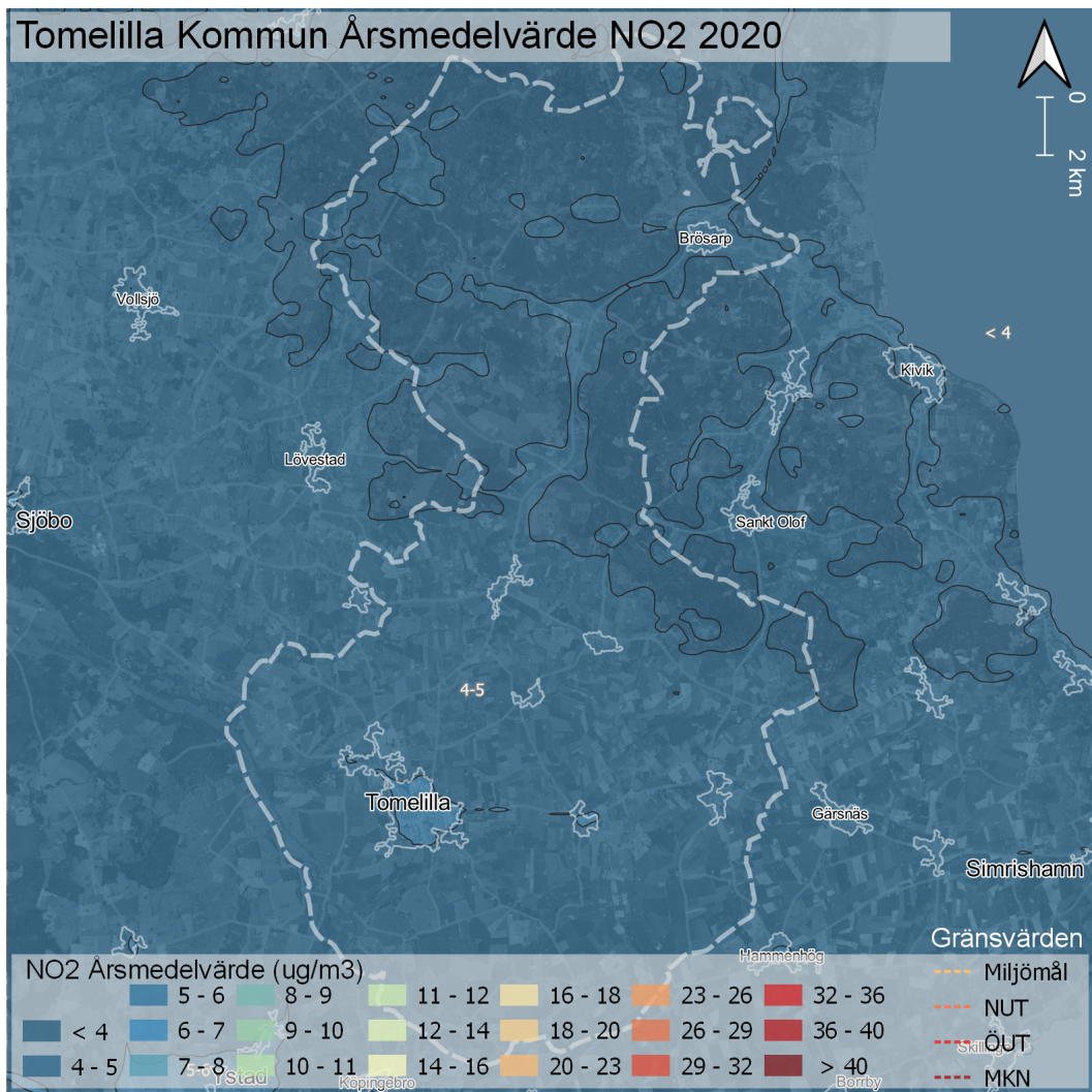
Figur 3. Karta som visar årsmedelvärden av NO 2 för år 2020 i Tomelilla kommun.
