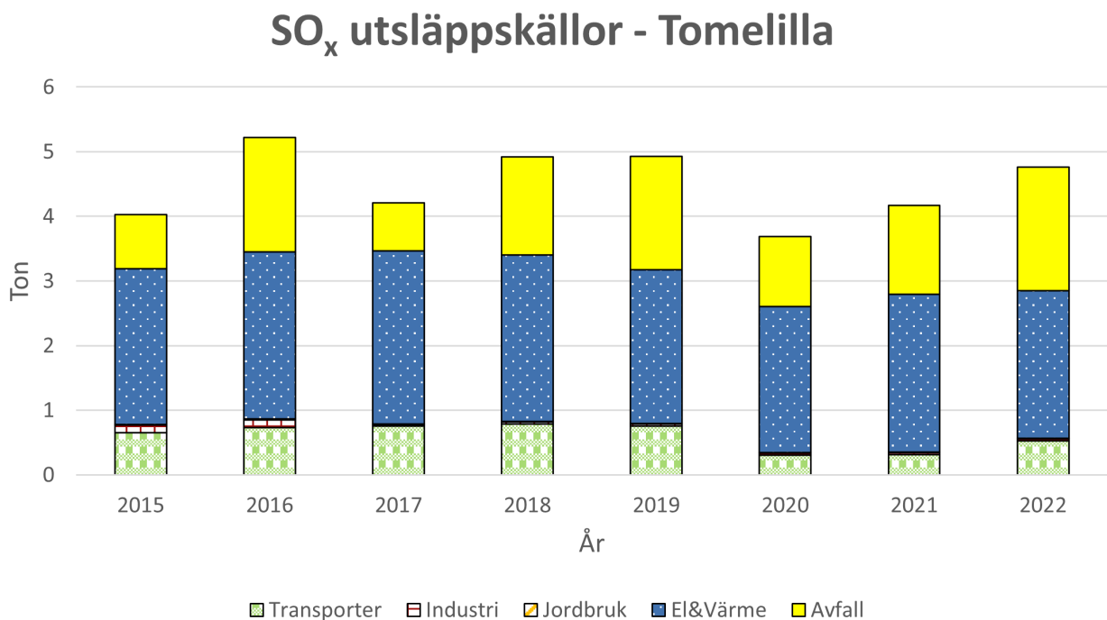
Figur 6. Visar utsläppskällorna av SO x för Tomelilla, beräknat värde från SMHI.
