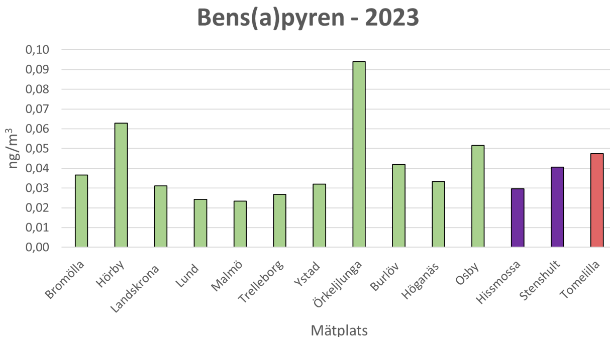
Figur 17. Visar hur medelkoncentrationen av bens(a)pyren i atmosfären såg ut i elva kommuner, två bakgrundstationer samt ett skattat värde för Tomelilla i Skåne under en tremånaders mätkampanj i 2023.
