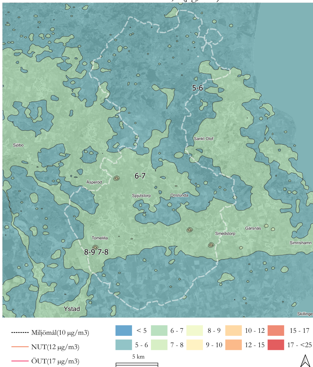
Figur 11. Karta som visar årsmedelvärdet av PM 2.5 för år 2022 i Tomelilla.
