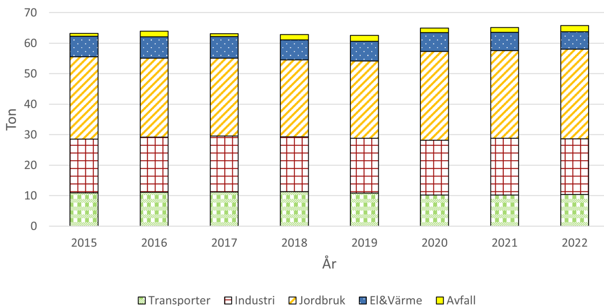
Figur 9. Visar utsläppskällorna av PM10 för Tomelilla, beräknat värde från SMHI.
