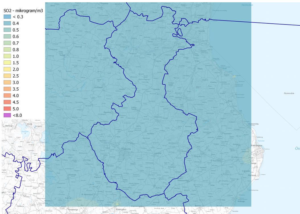
Figur 6. Karta som visar årsmedelvärdet av SO x för år 2019 i Tomelilla.
