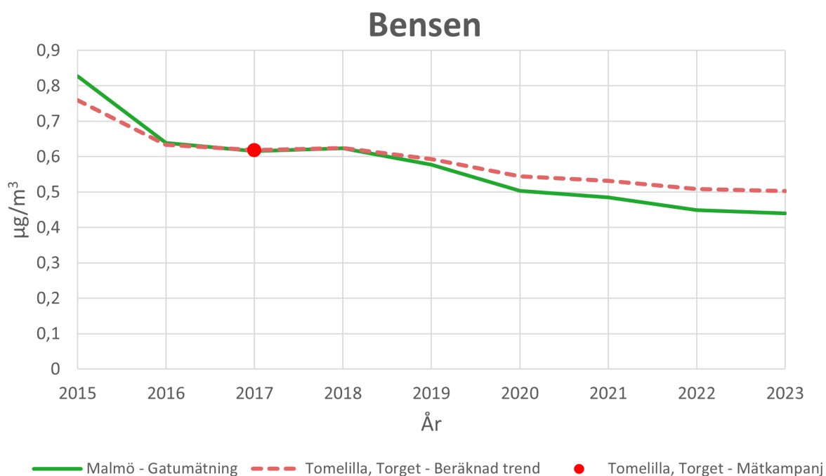
Figur 19. Visar hur koncentrationen av bensen i atmosfären har förändrats för år 2015 – 2023 i Tomelilla jämfört med Malmö.
