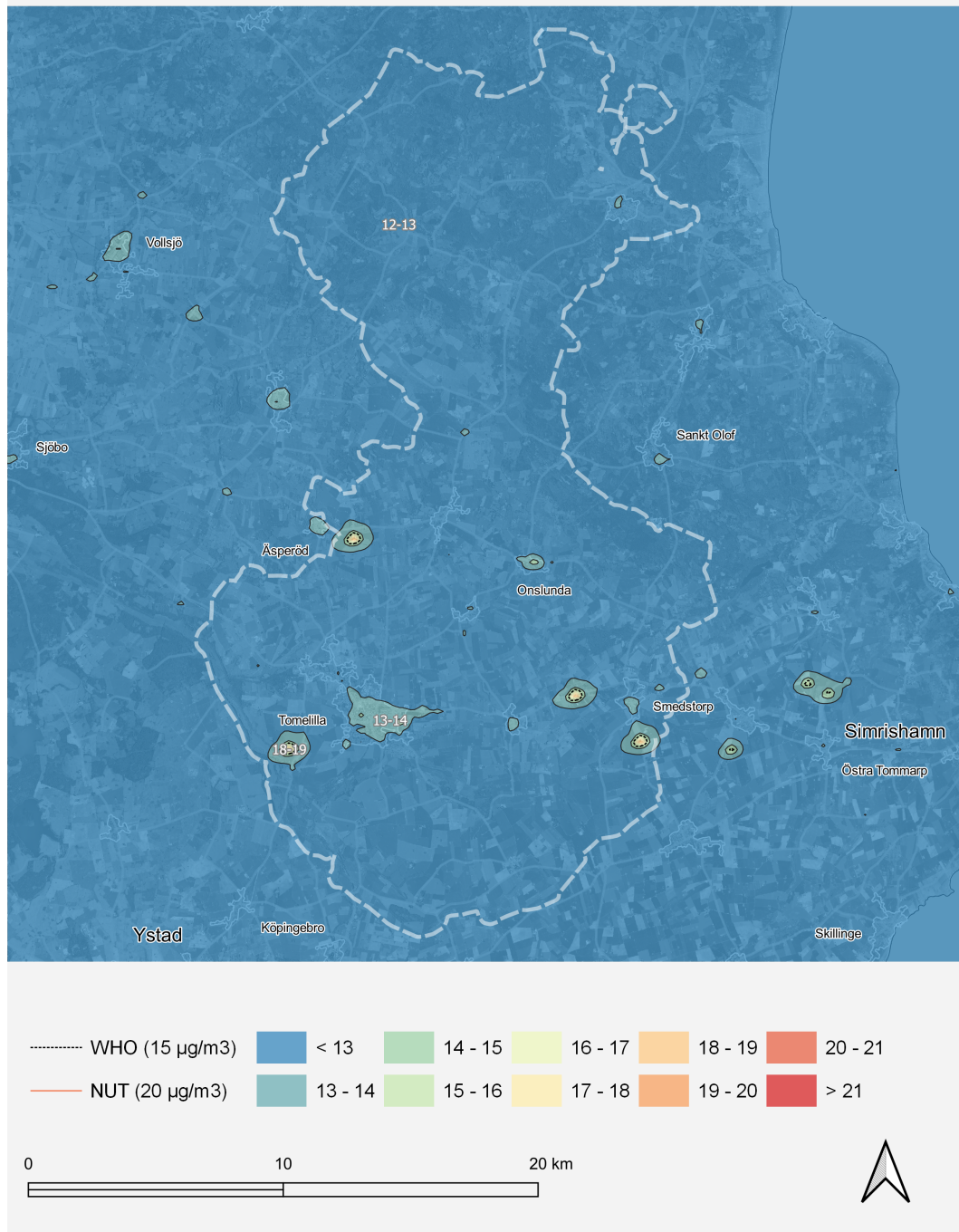
Figur 8. Karta som visar årsmedelvärdet av PM10 för år 2021 i Tomelilla.
