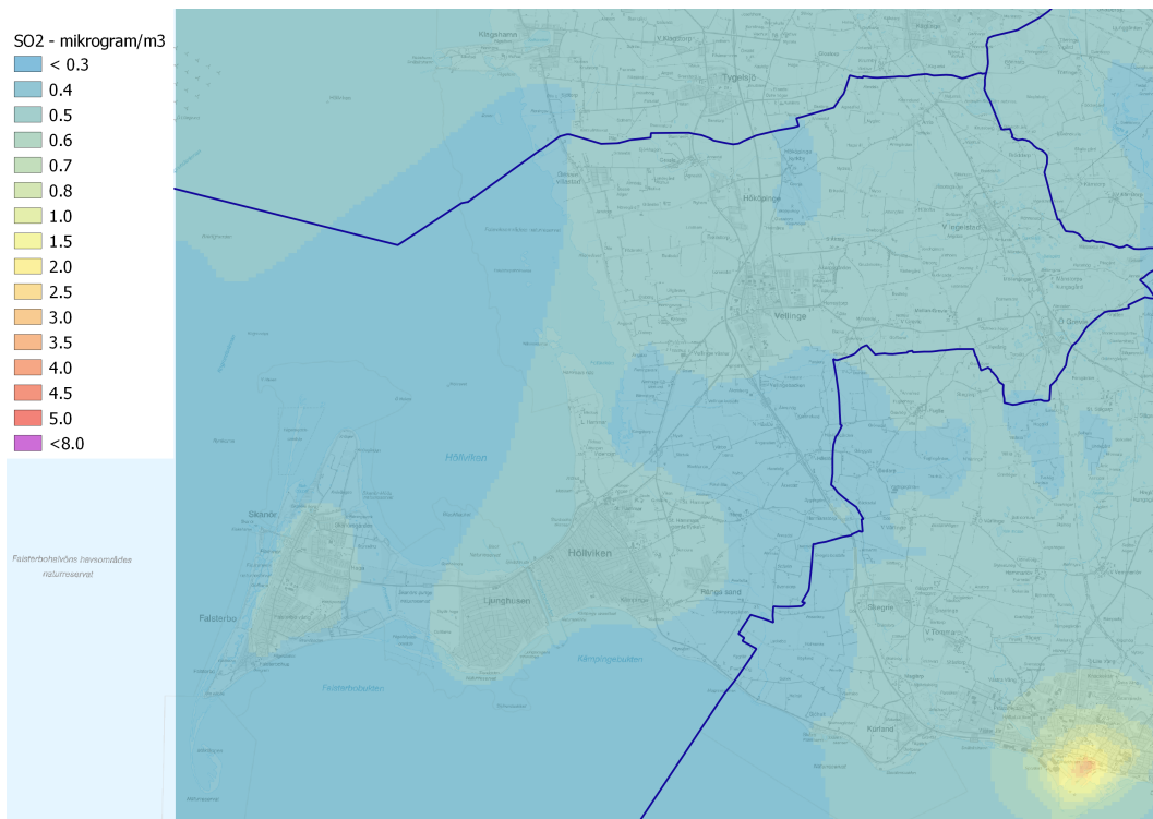
Figur 6. Karta som visar årsmedelvärdet av SO x för år 2019 i Vellinge.
